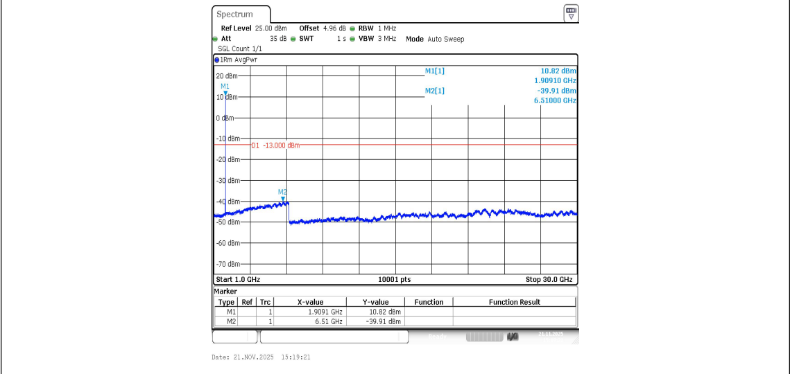
Band2-9538-4-1000~30000MHz-PASS
