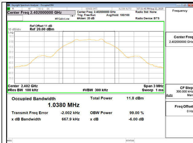
OBW_BLE 1M_LowCH00-2402MHz
