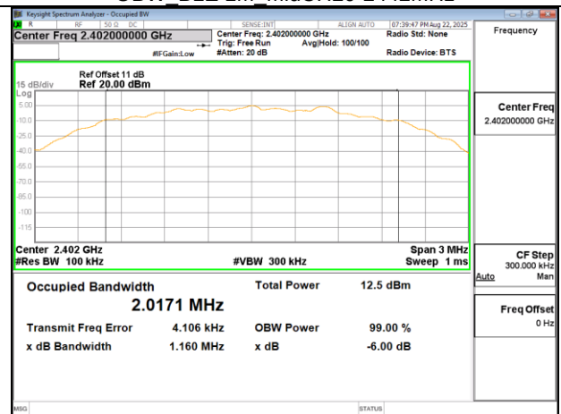
OBW_BLE 2M_LowCH00-2402MHz
