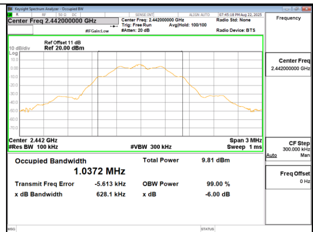
OBW_BLE 125k MidCH20-2442MHz
