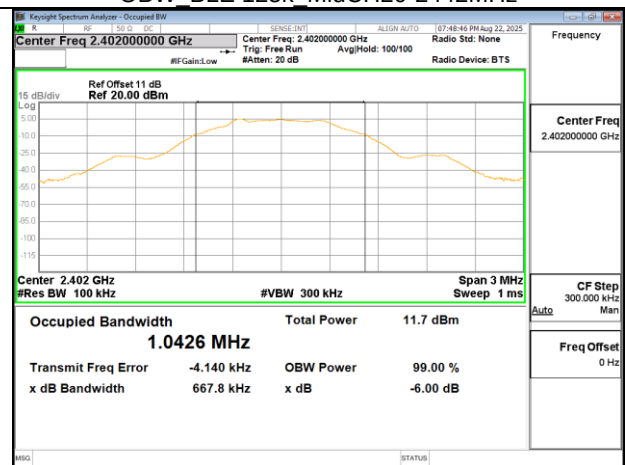
OBW_BLE 500k LowCH00-2402MHz
