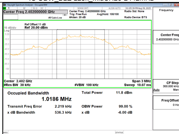
IC OBW_BLE 500k_LowCH00-2402MHz
