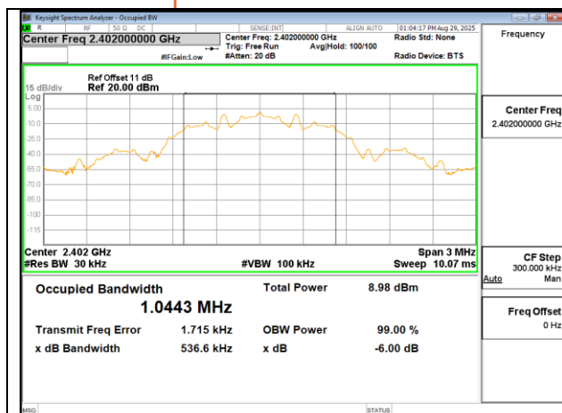
IC OBW_BLE 125k_LowCH00-2402MHz
