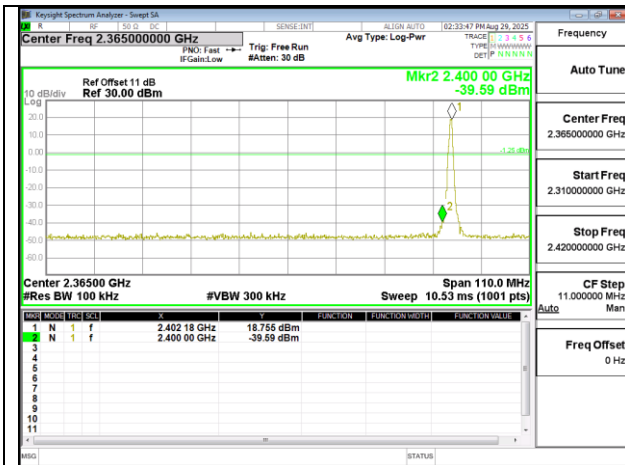
Band Edge GFSK 1M DH5 2402MHz
