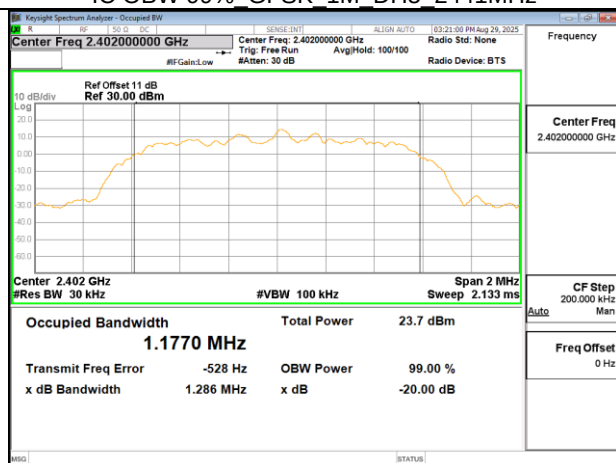
IC OBW 99% \pi/4 DQPSK 2M DH5 2402MHz
