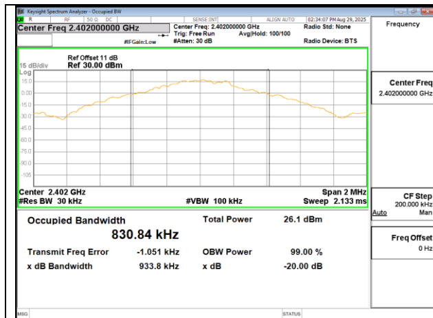
IC OBW 99% GFSK 1M DH5 2402MHz
