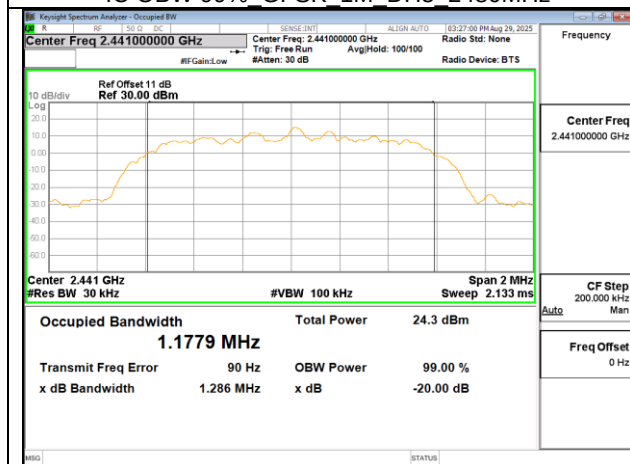
IC OBW 99% \pi/4 DQPSK 2M DH5 2441MHz
