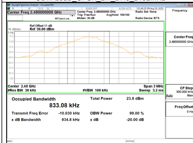
OBW 20dB GFSK 1M DH5 2480MHz
