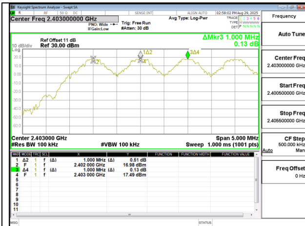
GFSK 1M DH5 CH0CH1CH2
