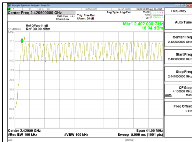
GFSK 1M DH5 2400-2441
