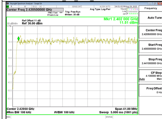
8DPSK 3M DH5 2400-2441
