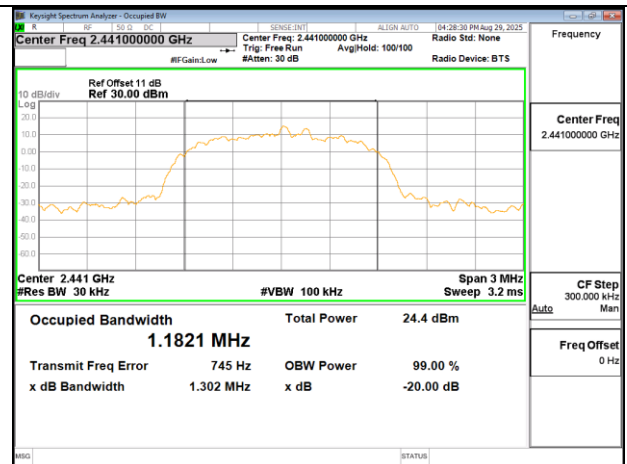
OBW 20dB 8DPSK 3M DH5 2441MHz
