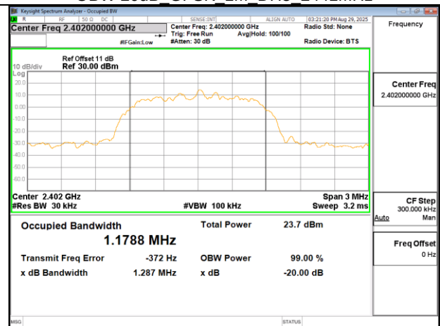
OBW 20dB \pi/4 DQPSK 2M DH5 2402MHz
