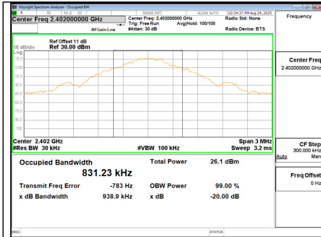
OBW 20dB GFSK 1M DH5 2402MHz
