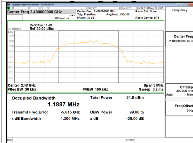
OBW 20dB 8DPSK 3M DH5 2480MHz
