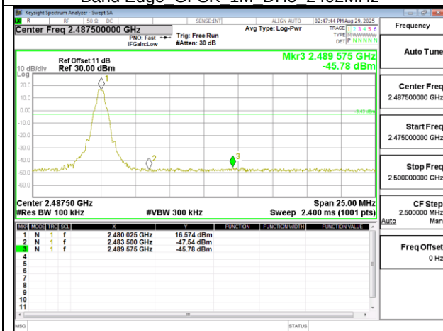
Band Edge GFSK 1M DH5 2480MHz
