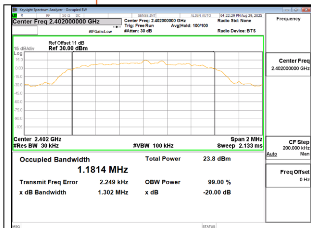
IC OBW 99% 8DPSK 3M DH5 2402MHz
