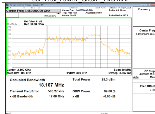
802.11ax 20MHz Chain1 2462MHz RU52 40
