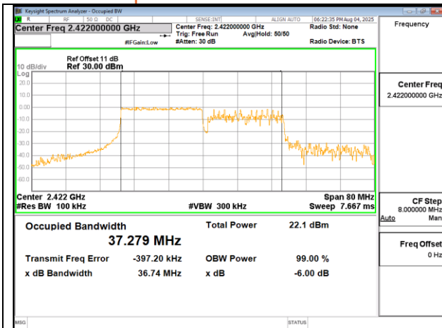
802.11ax 40MHz Chain1 2422MHz RU242 61
