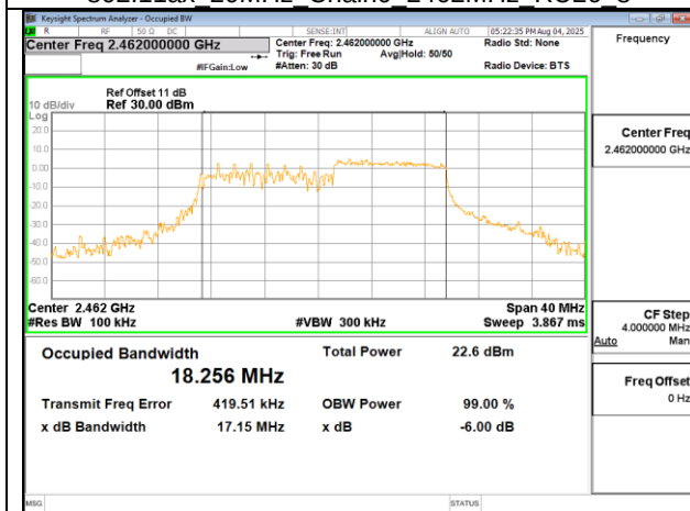
802.11ax 20MHz Chain0 2462MHz RU106 54
