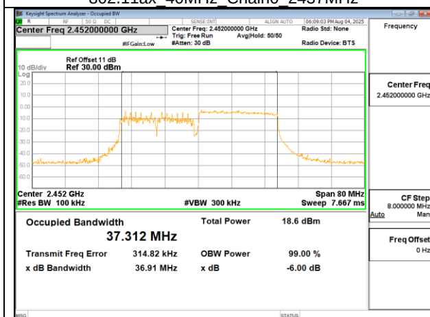
802.11ax 40MHz Chain0 2452MHz RU242 62
