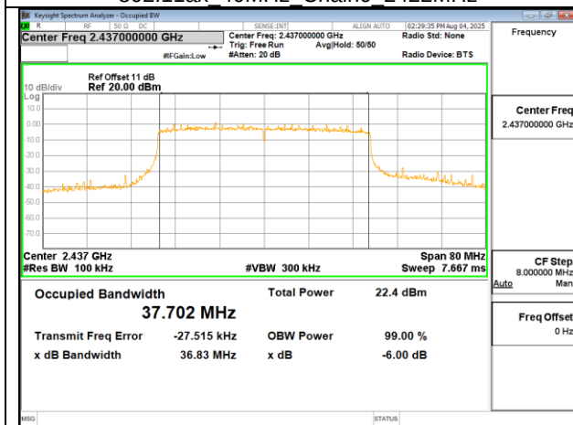
802.11ax 40MHz Chain0 2437MHz
