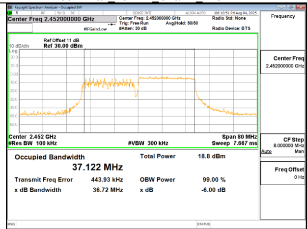
802.11ax 40MHz Chain1 2452MHz RU242 62
