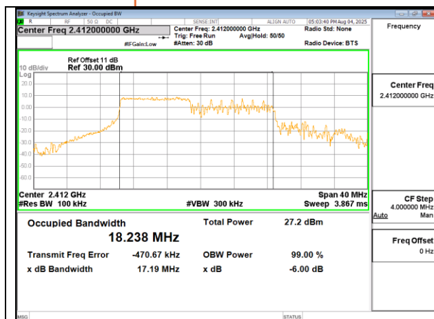
802.11ax 20MHz Chain1 2412MHz RU106 53
