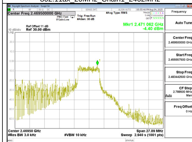
802.11ax 20MHz Chain1 2462MHz RU52 40
