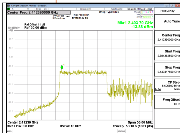
802.11ax 40MHz Chain1 2422MHz RU242 61
