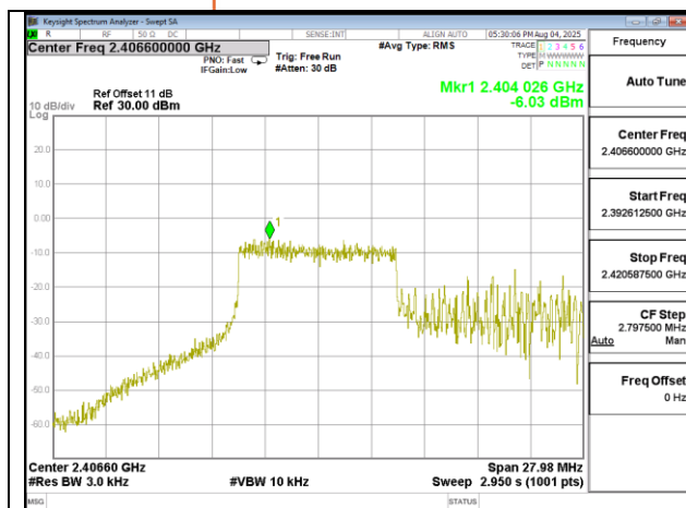
802.11ax 20MHz Chain1 2412MHz RU106 53
