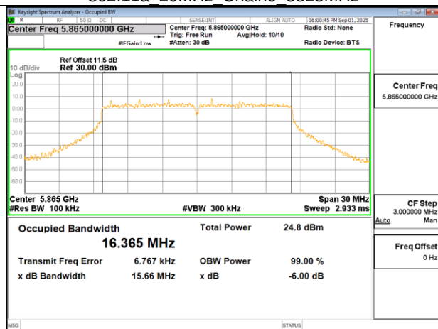
802.11a 20MHz Chain0 5865MHz
