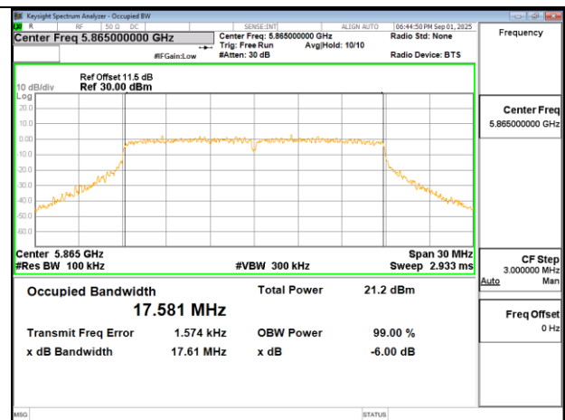
802.11n 20MHz Chain1 5865MHz
