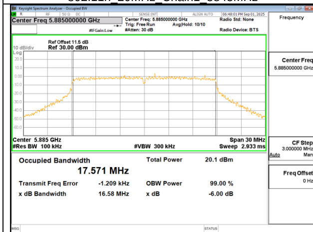
802.11n 20MHz Chain1 5885MHz
