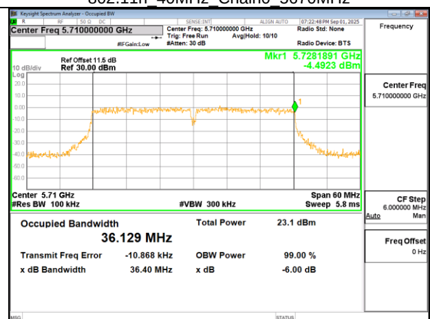
802.11n 40MHz Chain0 5710MHz UNII-3
