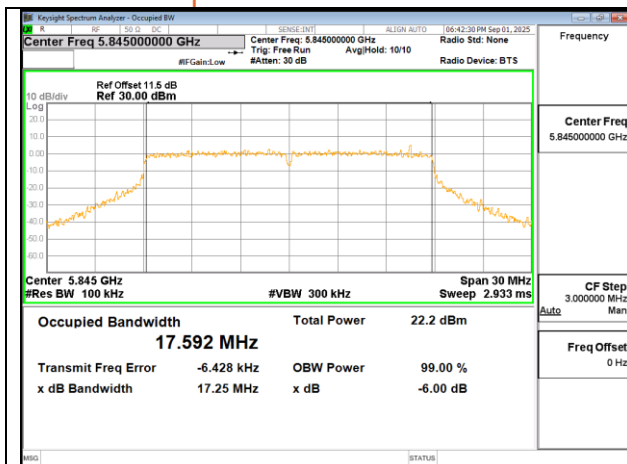
802.11n 20MHz Chain1 5845MHz
