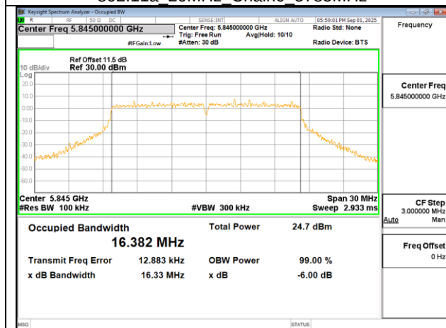
802.11a 20MHz Chain0 5845MHz
