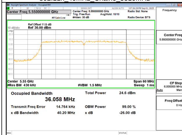
802.11n 40MHz Chain0 5550MHz
