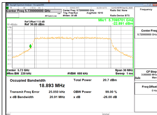
802.11ax 20MHz Chain0 5720MHz UNII-2C
