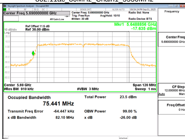
802.11ac 80MHz Chain1 5690MHz UNII-2C
