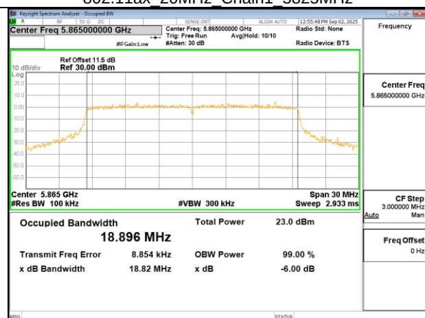
802.11ax 20MHz Chain1 5865MHz
