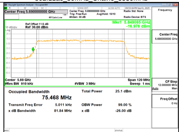
802.11ac 80MHz Chain0 5690MHz UNII-2C
