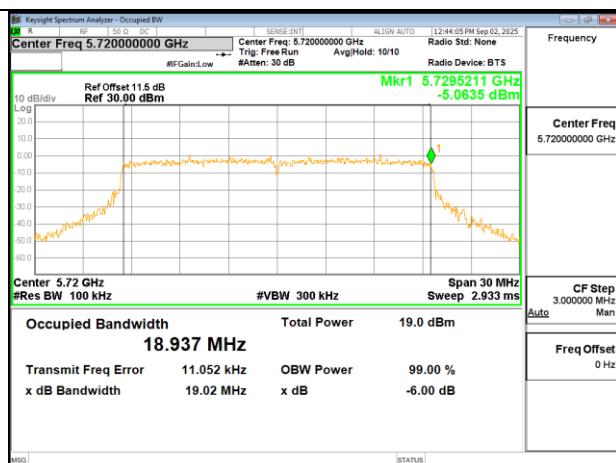
802.11ax 20MHz Chain0 5720MHz UNII-3
