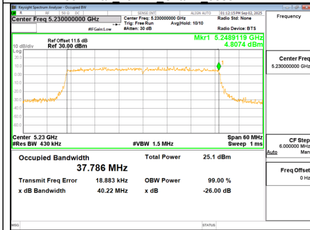
802.11ax 40MHz Chain0 5230MHz
