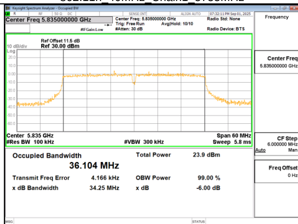
802.11n 40MHz Chain1 5835MHz
