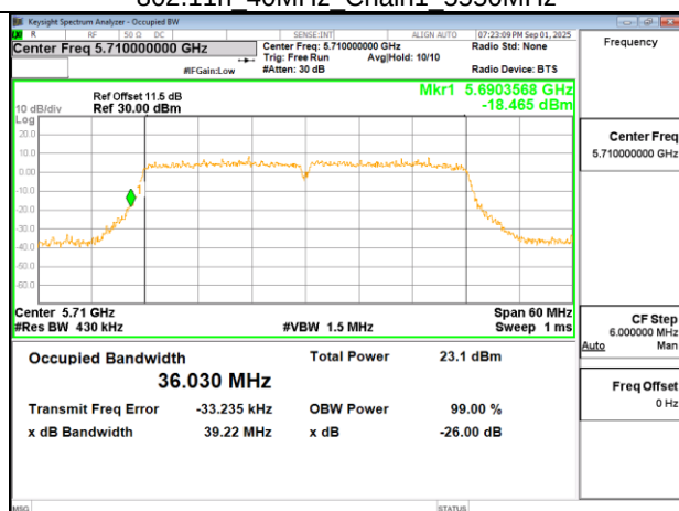
802.11n 40MHz Chain1 5710MHz UNII-2C
