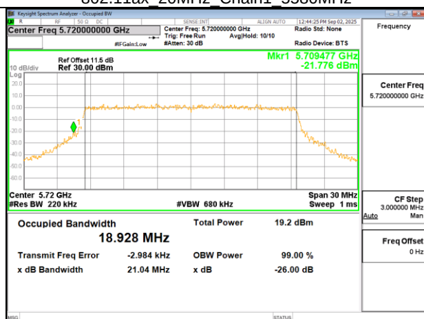
802.11ax 20MHz Chain1 5720MHz_UNII-2C
