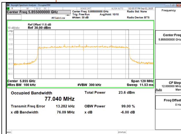
802.11ax 80MHz Chain1 5855MHz
