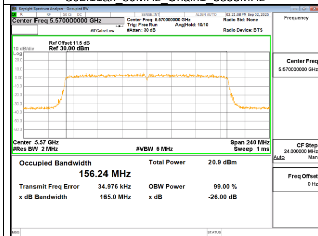
802.11ax 160MHz Chain0 5570MHz
