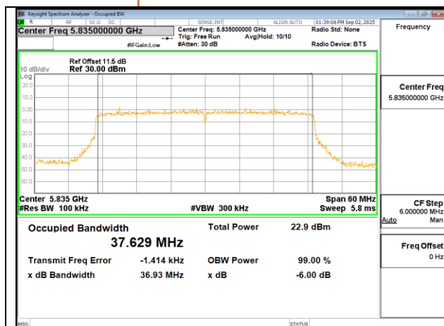
802.11ax 40MHz Chain0 5835MHz
