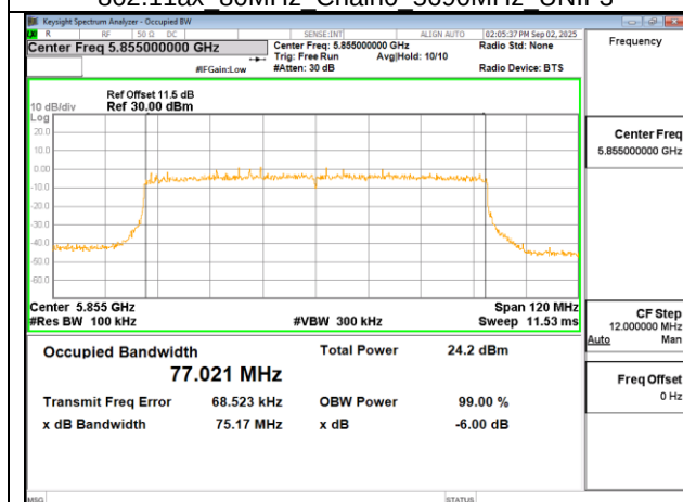
802.11ax 80MHz Chain0 5855MHz
