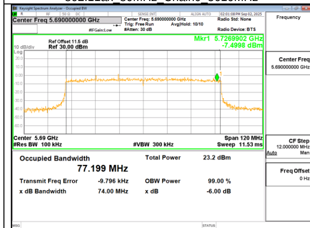
802.11ax 80MHz Chain0 5690MHz UNII-3
