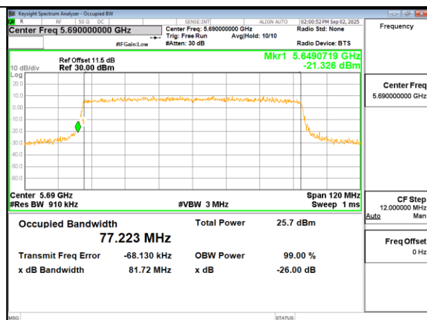
802.11ax 80MHz Chain0 5690MHz UNII-2C
