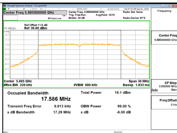
802.11n 20MHz Chain0 5885MHz
