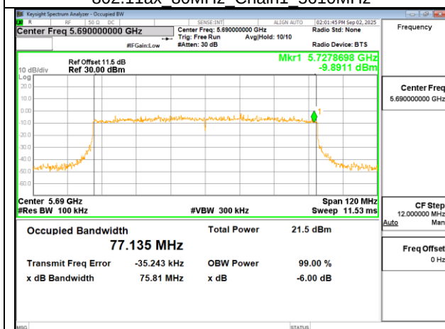
802.11ax 80MHz Chain1 5690MHz UNII-3
