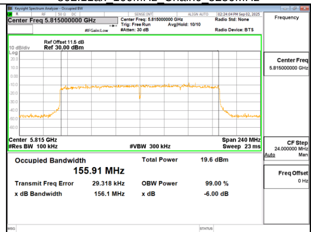
802.11ax 160MHz Chain0 5815MHz
