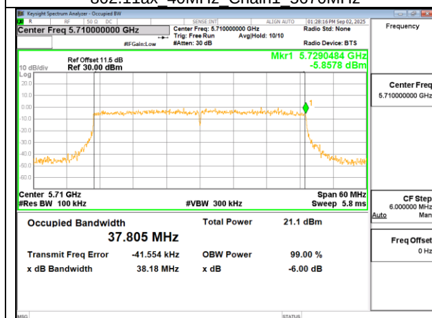
802.11ax 40MHz Chain1 5710MHz UNII-3
