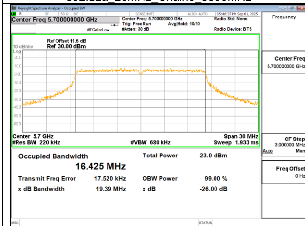
802.11a 20MHz Chain0 5700MHz
