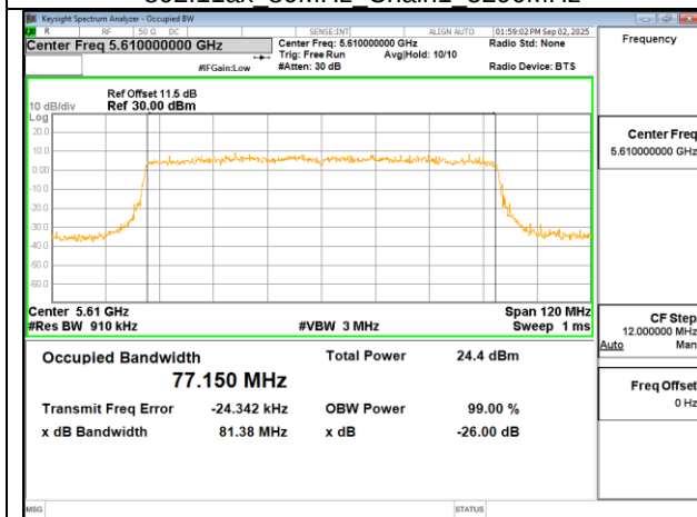
802.11ax 80MHz Chain1 5610MHz
