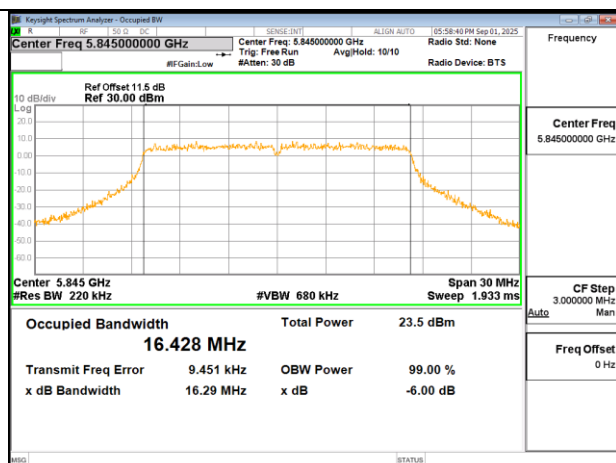
802.11a 20MHz Chain0 5845MHz
