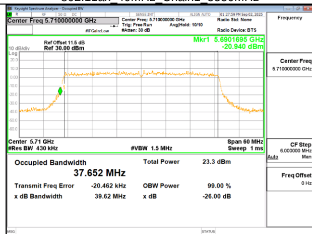
802.11ax 40MHz Chain1 5710MHz UNII-2C
