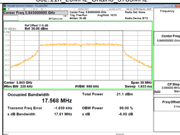
802.11n 20MHz Chain0 5845MHz
