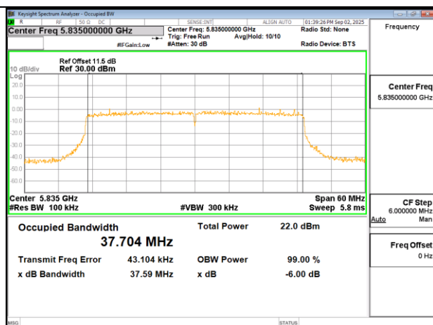
802.11ax 40MHz Chain1 5835MHz
