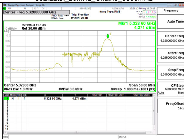
802.11ax 20MHz Chain0 5320MHz RU26 8
