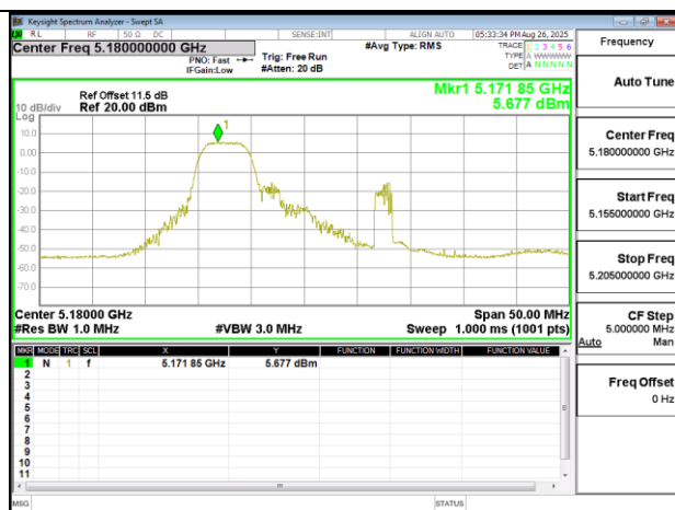
802.11ax 20MHz Chain1 5180MHz RU52_37
