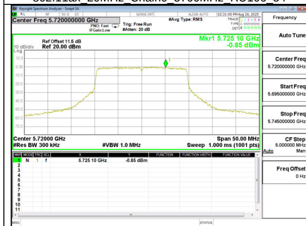
802.11ax 20MHz Chain0 5720MHz UNII 3
