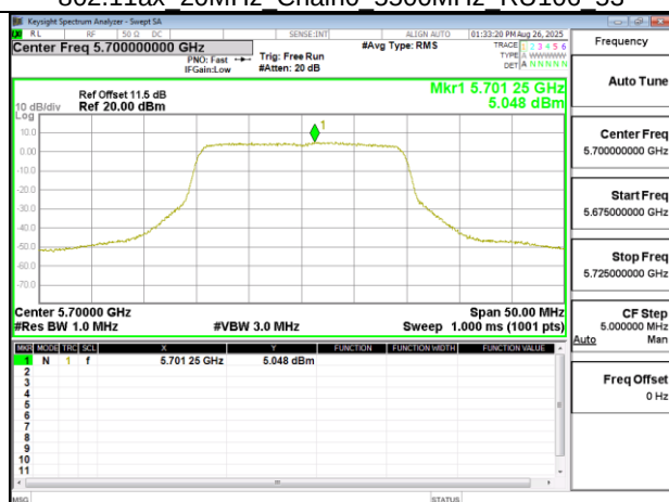
802.11ax 20MHz Chain0 5700MHz
