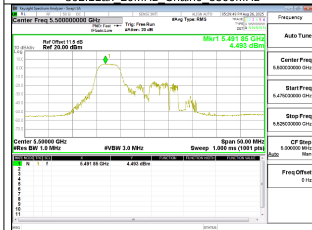
802.11ax 20MHz Chain0 5500MHz RU52 37
