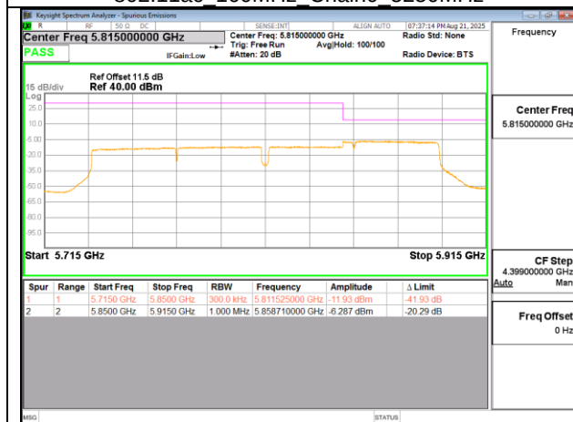
802.11ac 160MHz Chain0 5815MHz UNII 2C
