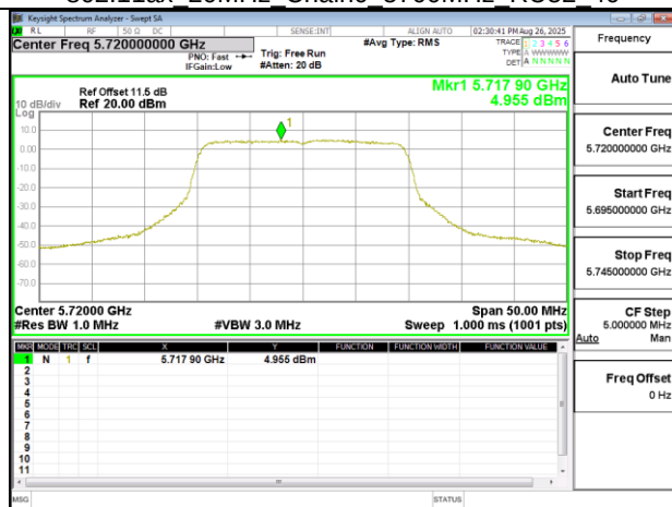
802.11ax 20MHz Chain0 5720MHz UNII 2C
