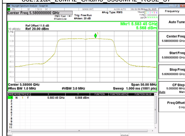
802.11ax 20MHz Chain0 5580MHz
