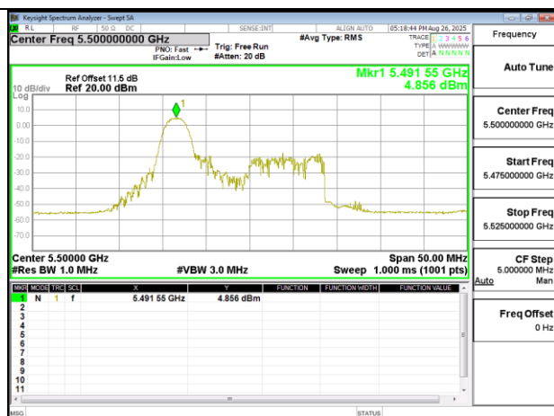
802.11ax 20MHz Chain0 5500MHz RU26 0
