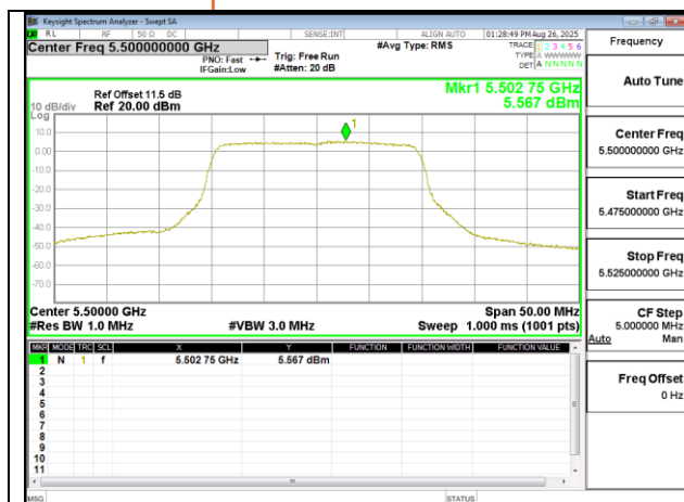
802.11ax 20MHz Chain0 5500MHz
