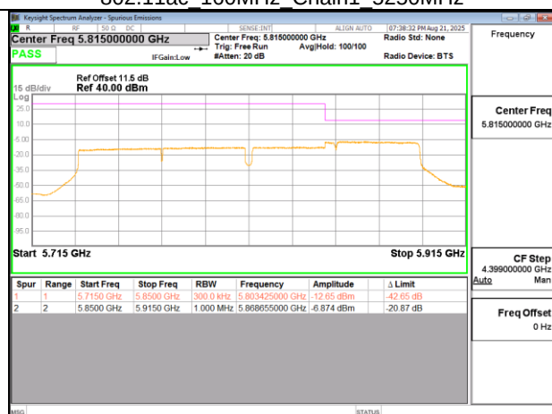
802.11ac 160MHz Chain1 5815MHz UNII 2C
