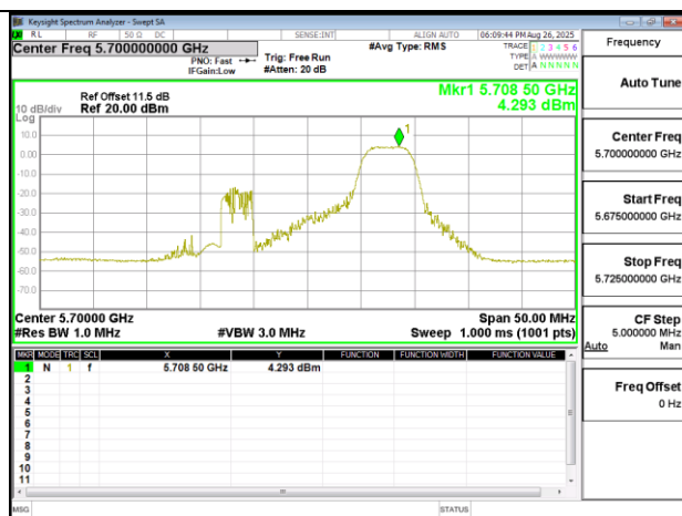
802.11ax 20MHz Chain0 5700MHz RU52 40
