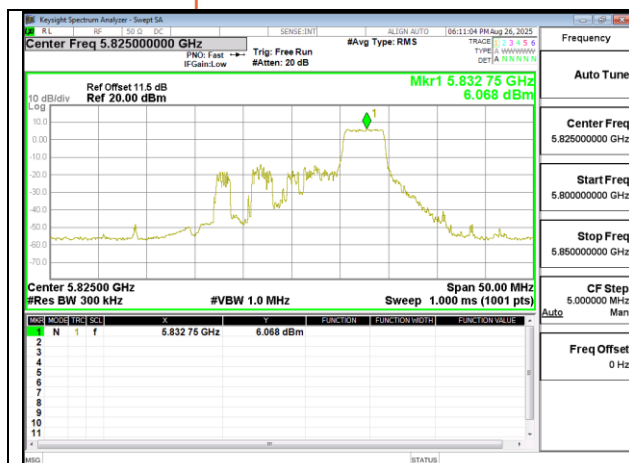
802.11ax 20MHz Chain0 5825MHz RU52 40
