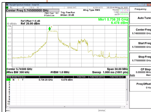
802.11ax 20MHz Chain1 5745MHz RU52 37
