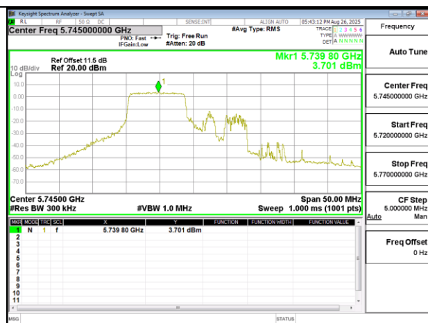
802.11ax 20MHz Chain1 5745MHz RU106 53
