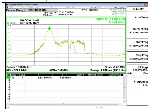
802.11ax 20MHz Chain1 5180MHz RU26_0
