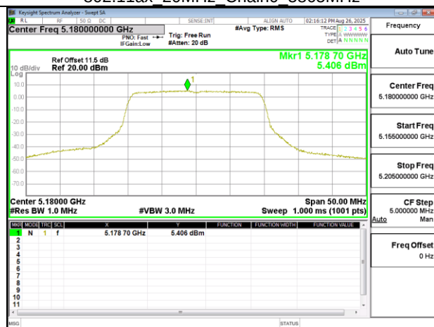
802.11ax 20MHz Chain1 5180MHz
