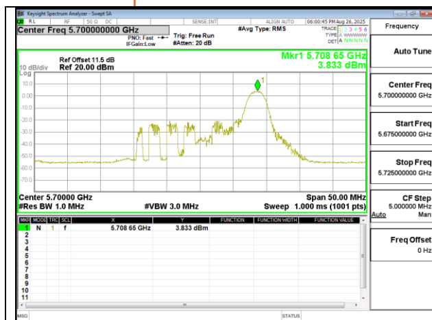
802.11ax 20MHz Chain0 5700MHz RU26 8
