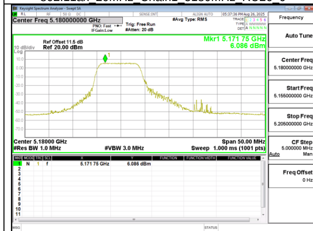
802.11ax 20MHz Chain1 5180MHz RU106_53
