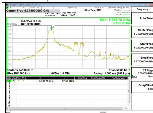
802.11ax 20MHz Chain0 5745MHz RU26_0
