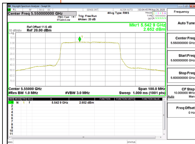
802.11ax 40MHz Chain0 5550MHz
