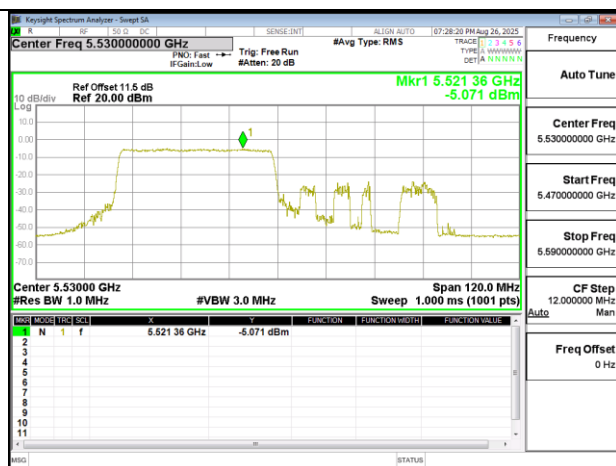
802.11ax 80MHz Chain0 5530MHz RU484 65
