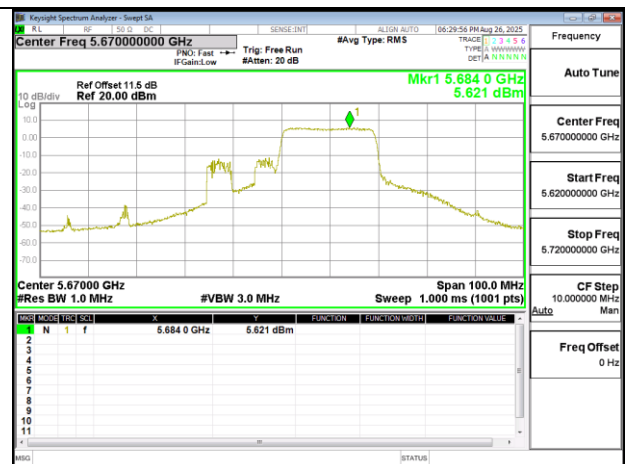
802.11ax 40MHz Chain1 5670MHz RU242 62
