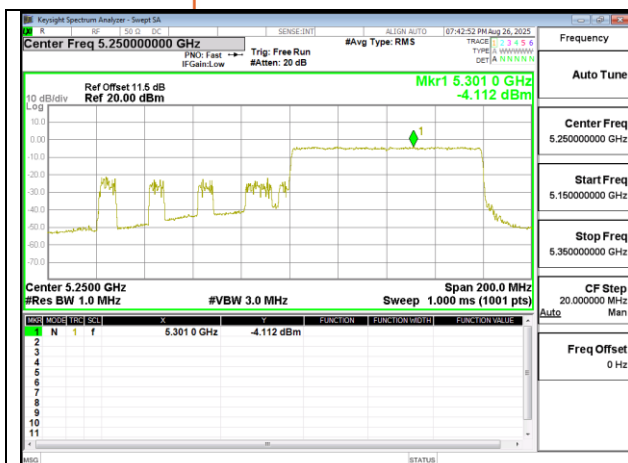
802.11ax 160MHz Chain1 5250MHz RU996 S67
