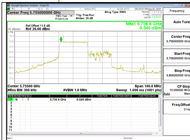
802.11ax 40MHz Chain0 5755MHz RU242 61
