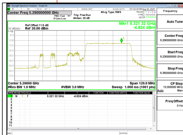
802.11ax 80MHz Chain1 5290MHz RU484 66
