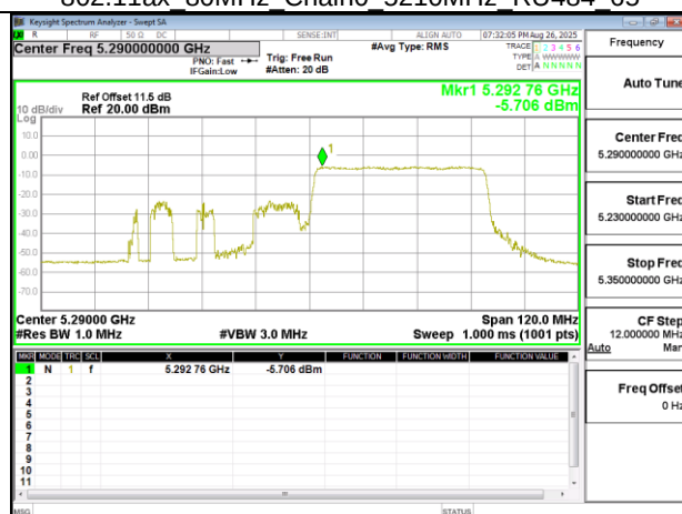
802.11ax 80MHz Chain0 5290MHz RU484 66
