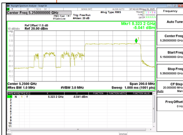
802.11ax 160MHz Chain0 5250MHz RU996 S67
