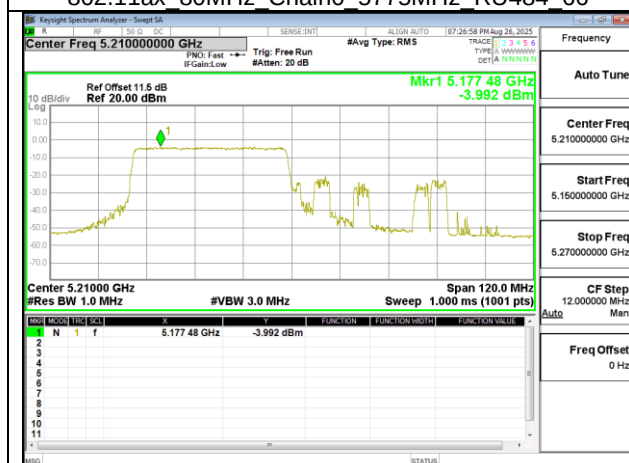
802.11ax 80MHz Chain1 5210MHz RU484 65
