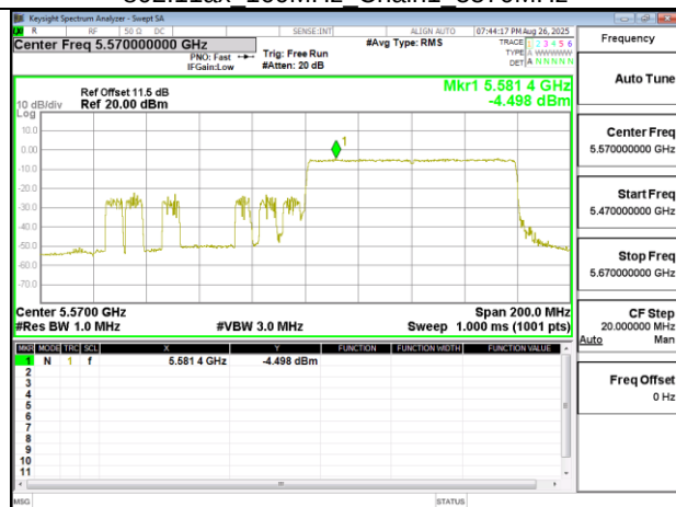
802.11ax 160MHz Chain1 5570MHz RU996 S67
