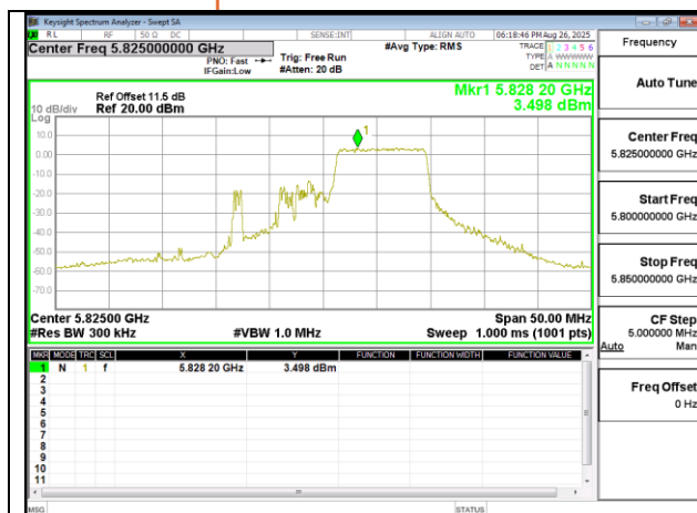
802.11ax 20MHz Chain1 5825MHz RU106 54
