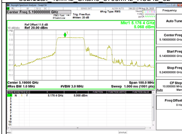
802.11ax 40MHz Chain1 5190MHz RU242 61
