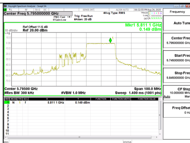
802.11ax 40MHz Chain1 5795MHz RU242 62
