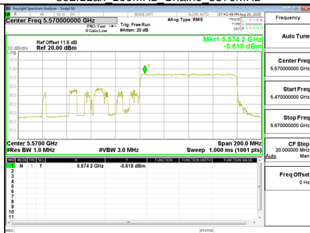
802.11ax 160MHz Chain0 5570MHz RU996 S67
