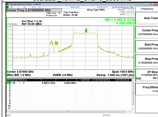
802.11ax 40MHz Chain0 5670MHz RU242 62
