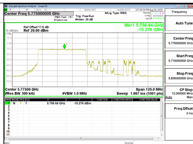
802.11ax 80MHz Chain0 5775MHz RU484 65
