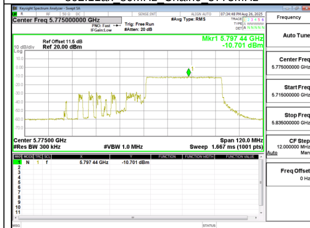
802.11ax 80MHz Chain0 5775MHz RU484 66
