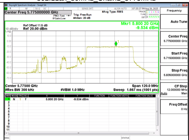
802.11ax 80MHz Chain1 5775MHz RU484 66
