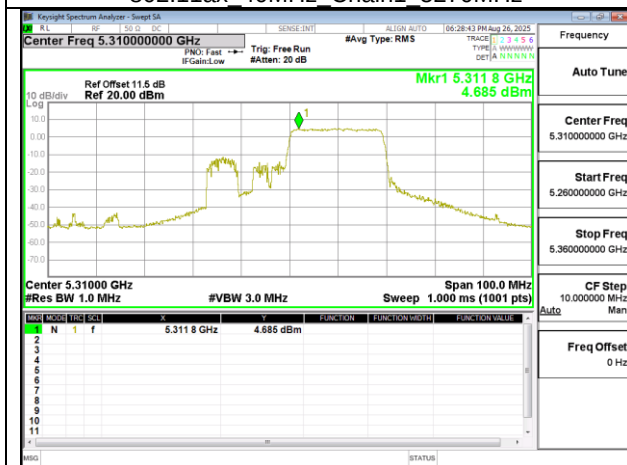
802.11ax 40MHz Chain1 5310MHz RU242 62
