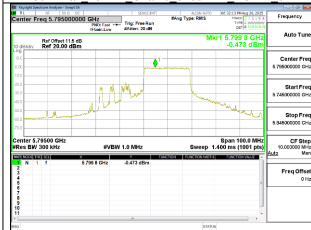
802.11ax 40MHz Chain0 5795MHz RU242 62
