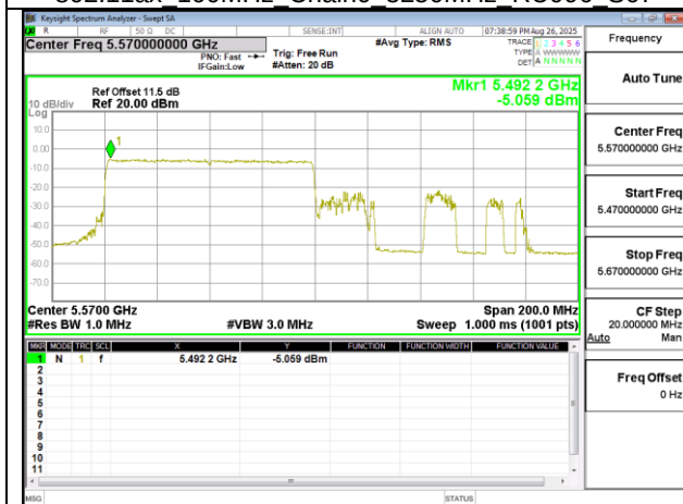
802.11ax 160MHz Chain0 5570MHz RU996 67
