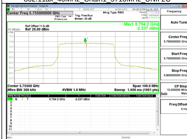
802.11ax 40MHz Chain1 5755MHz
