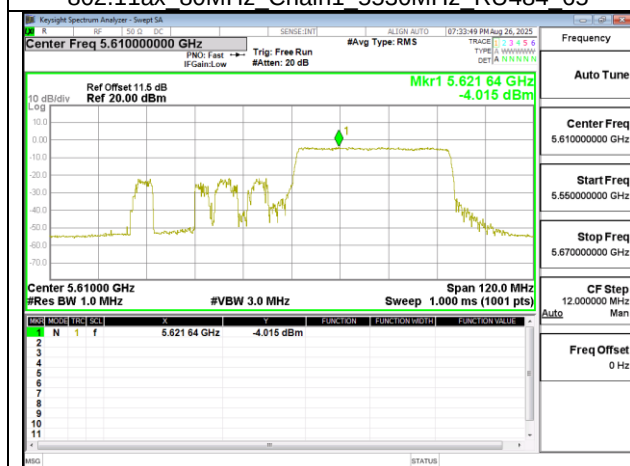
802.11ax 80MHz Chain1 5610MHz RU484 66
