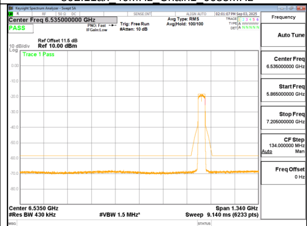
802.11ax 40MHz Chain1 6885MHz
