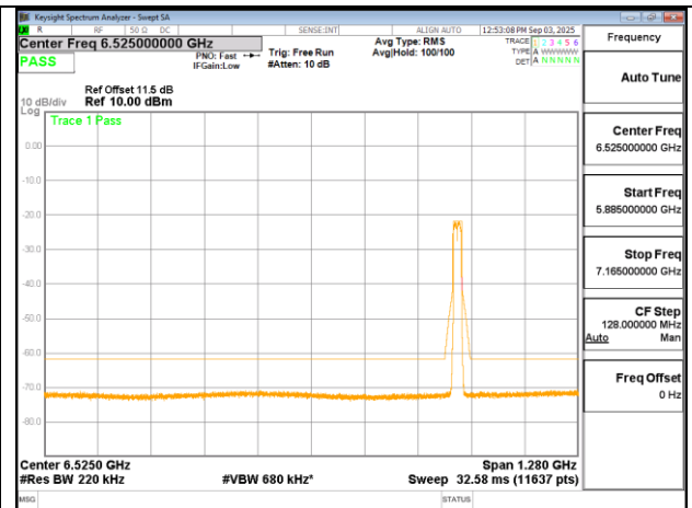
802.11ax 20MHz Chain1 6875MHz
