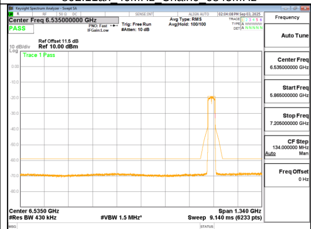
802.11ax 40MHz Chain0 6925MHz
