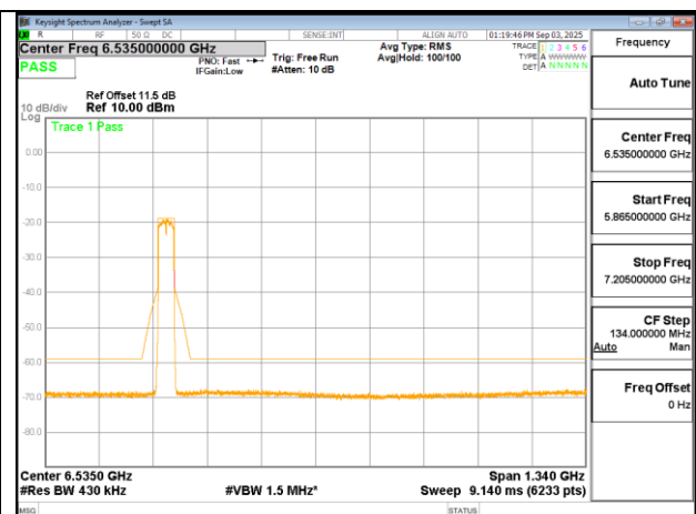
802.11ax 40MHz Chain1 6165MHz
