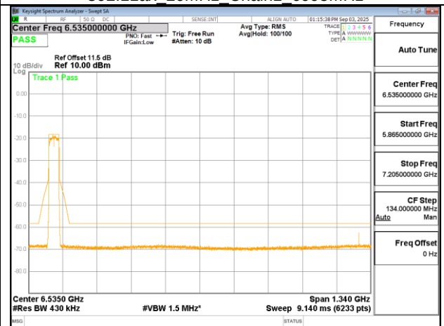
802.11ax 40MHz Chain0 5965MHz
