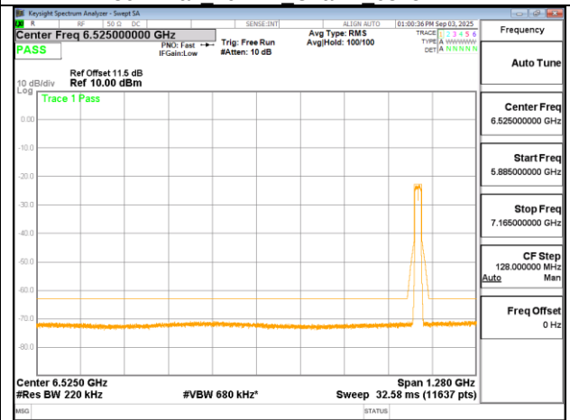
802.11ax 20MHz Chain1 6995MHz
