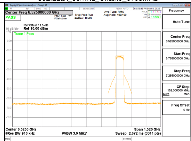
802.11ax 80MHz Chain0 6865MHz
