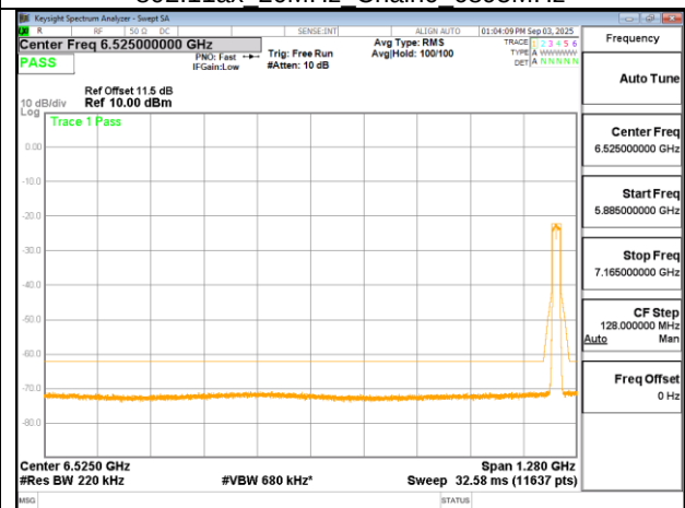
802.11ax 20MHz Chain0 7115MHz
