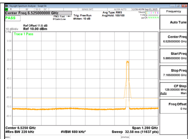
802.11ax 20MHz Chain0 6895MHz
