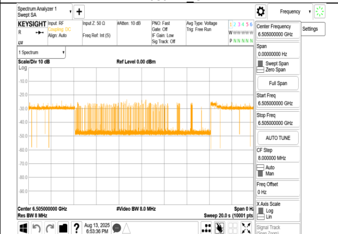
802.11ax_160MHz_CF 6505MHz_Interference_6505MHz_- 65.16dBm_Minimal
