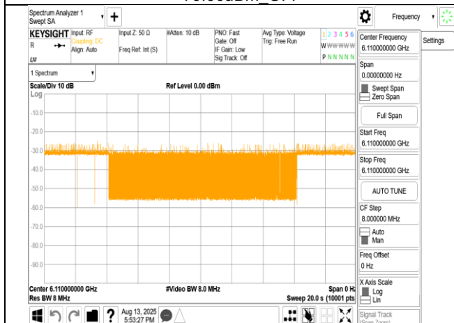
802.11ax_160MHz_CF 6185MHz_Interference_6110MHz_- 76.06dBm_ON
