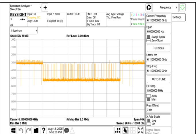
802.11ax_160MHz_CF 6185MHz_Interference_6110MHz_- 73.06dBm_Minimal
