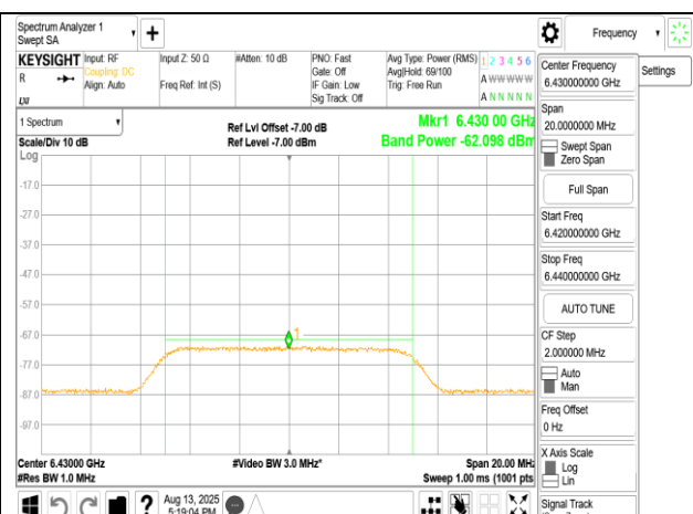
802.11ax 160MHz 6505MHz AWGN:6430
