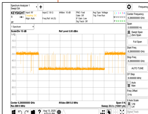
802.11ax_160MHz_CF 6185MHz_Interference_6260MHz_- 73.04dBm_Minimal
