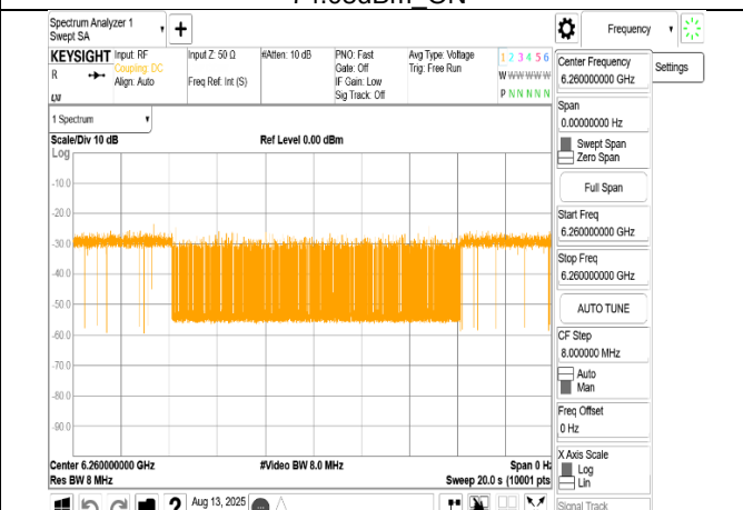
802.11ax_160MHz_CF 6185MHz_Interference_6260MHz_- 76.04dBm_ON
