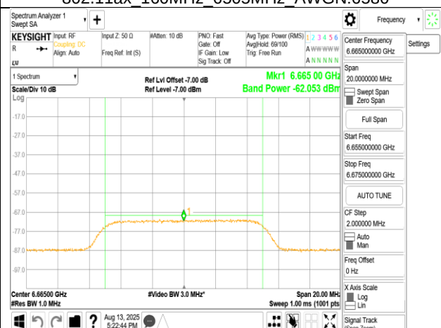
802.11ax 160MHz 6665MHz AWGN:6665MHz
