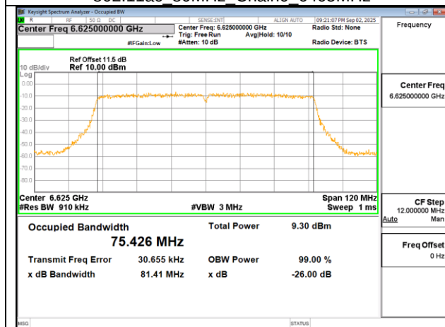
802.11ac 80MHz Chain0 6625MHz
