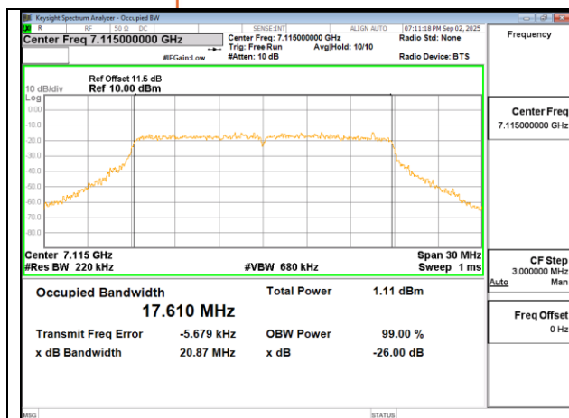
802.11ac 20MHz Chain1 7115MHz
