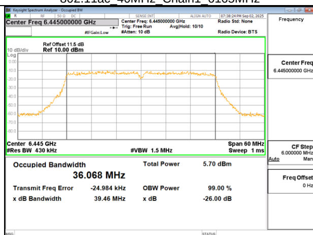
802.11ac 40MHz Chain1 6445MHz
