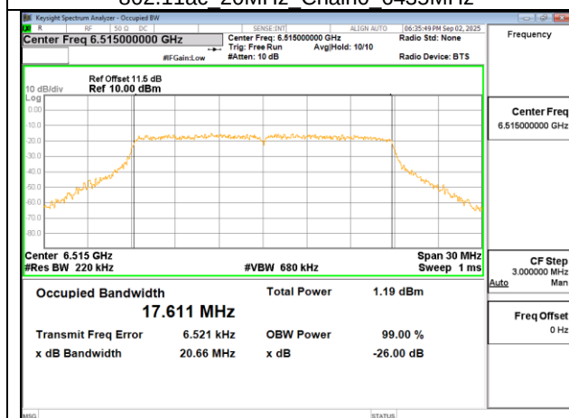
802.11ac 20MHz Chain0 6515MHz
