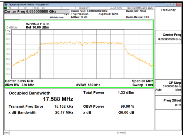
802.11ac 20MHz Chain1 6695MHz
