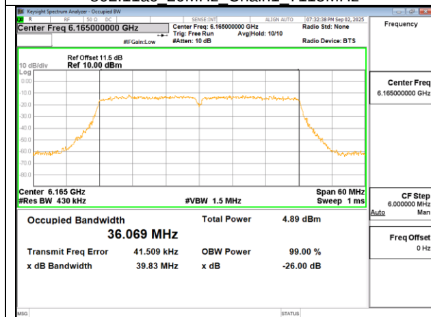
802.11ac 40MHz Chain0 6165MHz
