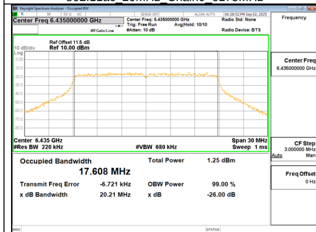
802.11ac 20MHz Chain0 6435MHz
