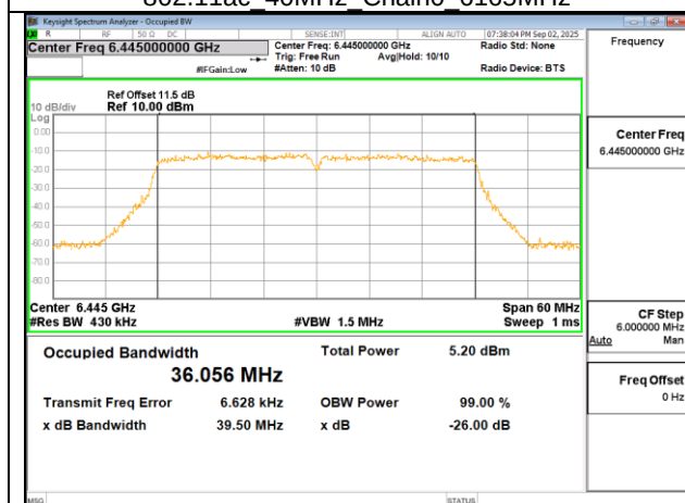
802.11ac 40MHz Chain0 6445MHz
