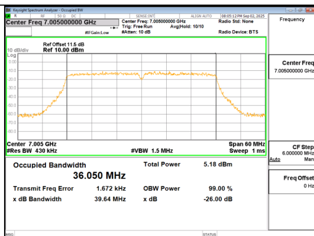
802.11ac 40MHz Chain1 7005MHz
