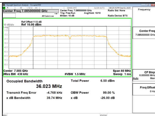
802.11ac 40MHz Chain0 7085MHz
