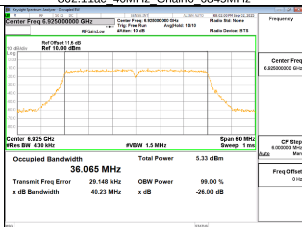
802.11ac 40MHz Chain0 6925MHz
