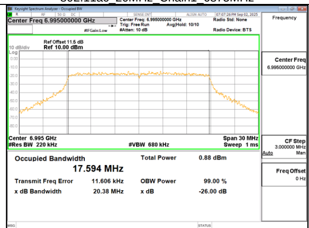
802.11ac 20MHz Chain1 6995MHz
