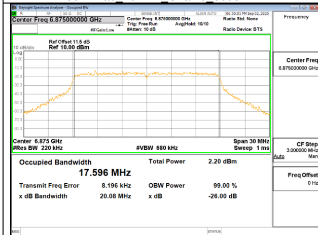
802.11ac 20MHz Chain0 6875MHz
