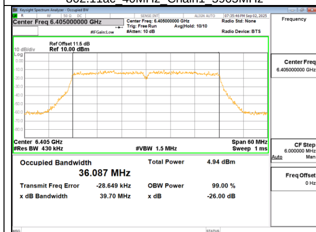
802.11ac 40MHz Chain1 6405MHz
