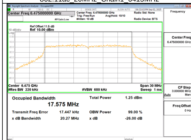
802.11ac 20MHz Chain1 6475MHz
