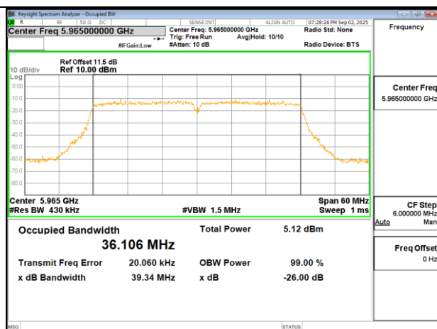
802.11ac 40MHz Chain0 5965MHz
