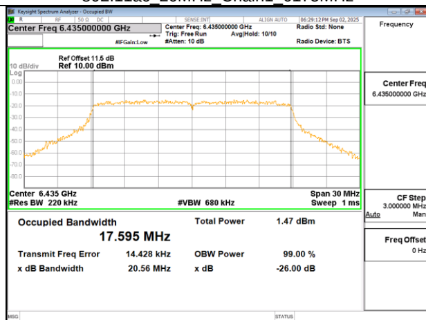
802.11ac 20MHz Chain1 6435MHz
