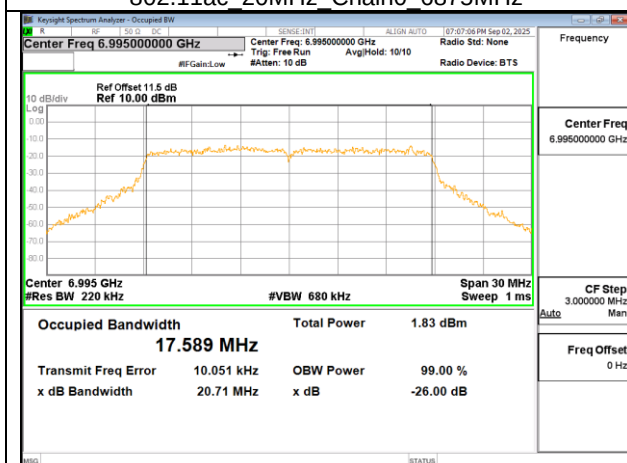
802.11ac 20MHz Chain0 6995MHz
