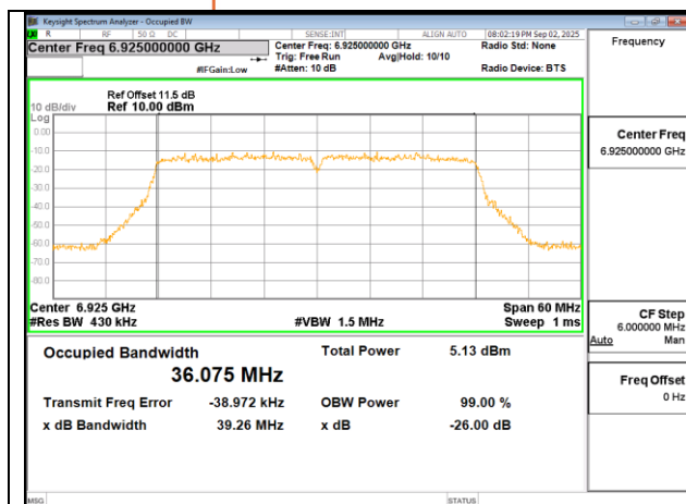
802.11ac 40MHz Chain1 6925MHz
