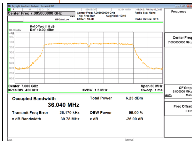
802.11ac 40MHz Chain0 7005MHz
