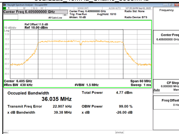
802.11ac 40MHz Chain0 6405MHz
