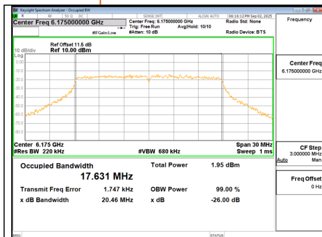
802.11ac 20MHz Chain0 6175MHz
