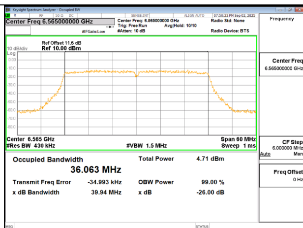
802.11ac 40MHz Chain0 6565MHz
