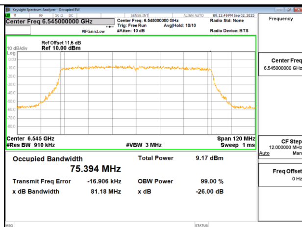
802.11ac 80MHz Chain0 6545MHz
