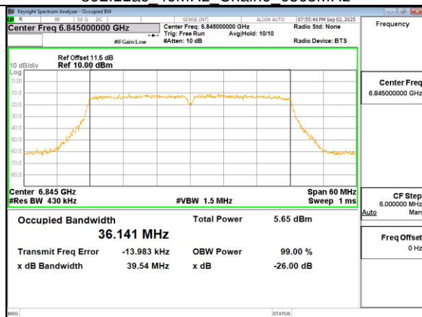
802.11ac 40MHz Chain0 6845MHz
