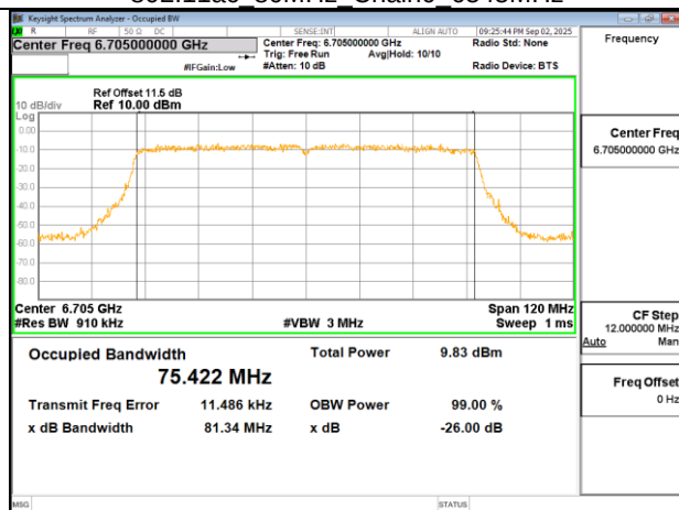
802.11ac 80MHz Chain0 6705MHz
