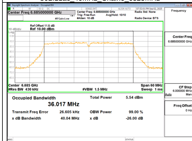
802.11ac 40MHz Chain0 6685MHz
