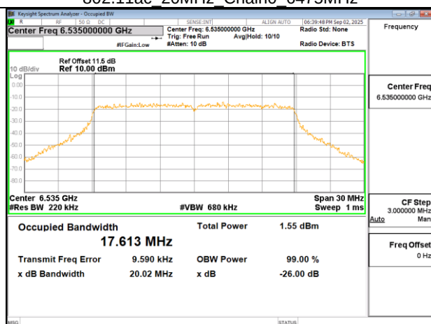
802.11ac 20MHz Chain0 6535MHz
