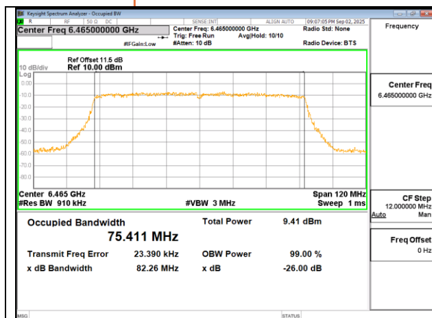
802.11ac 80MHz Chain0 6465MHz
