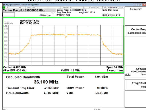
802.11ac 40MHz Chain0 6485MHz
