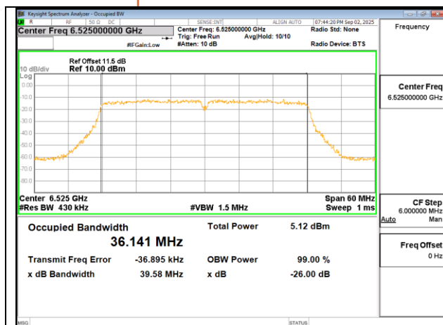
802.11ac 40MHz Chain0 6525MHz
