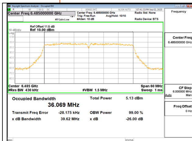
802.11ac 40MHz Chain1 6485MHz
