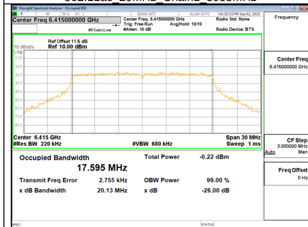
802.11ac 20MHz Chain1 6415MHz
