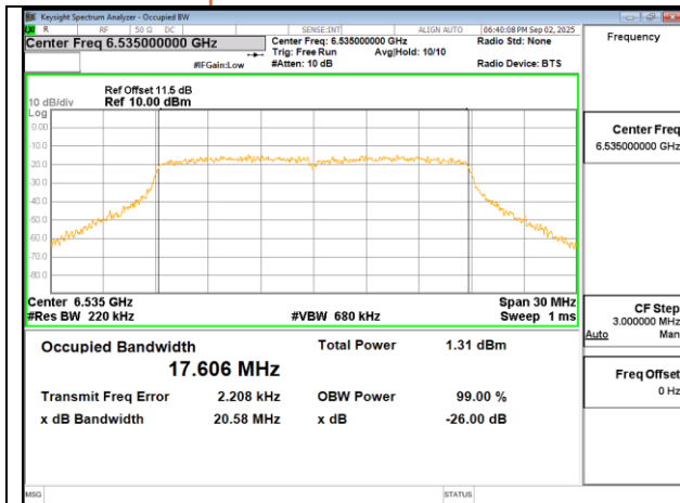
802.11ac 20MHz Chain1 6535MHz
