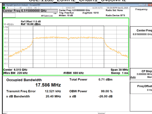
802.11ac 20MHz Chain1 6515MHz
