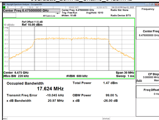
802.11ac 20MHz Chain0 6475MHz
