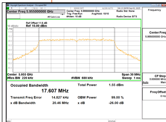
802.11ac 20MHz Chain1 5955MHz
