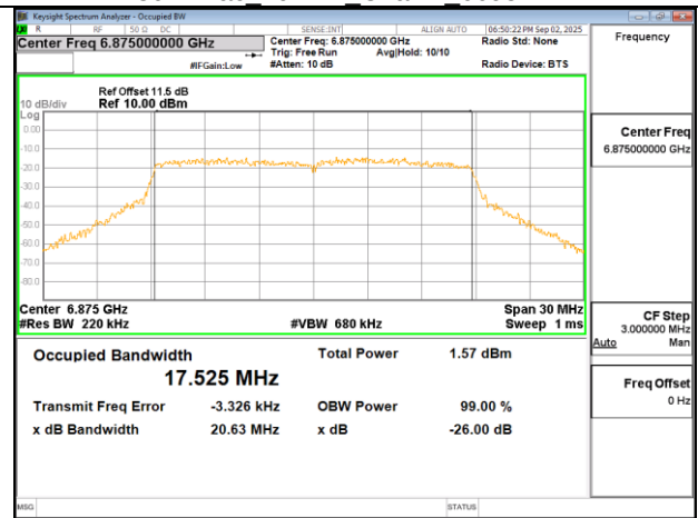
802.11ac 20MHz Chain1 6875MHz
