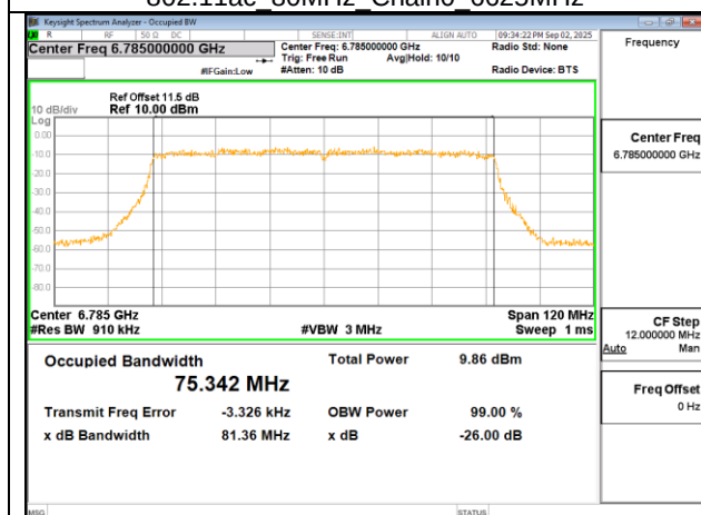
802.11ac 80MHz Chain0 6785MHz
