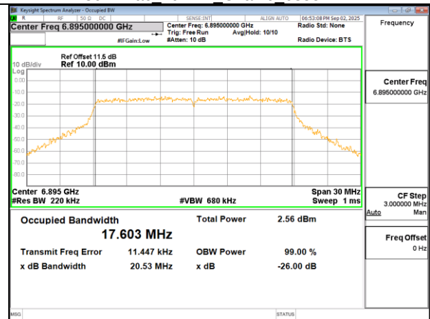
802.11ac 20MHz Chain0 6895MHz
