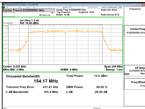
802.11ac 160MHz Chain0 6025MHz
