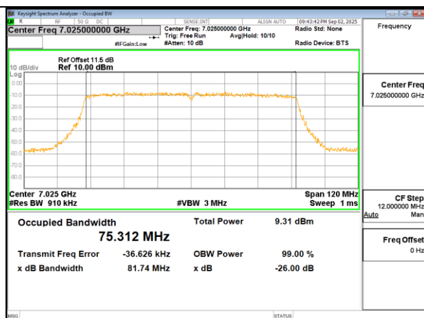
802.11ac 80MHz Chain0 7025MHz
