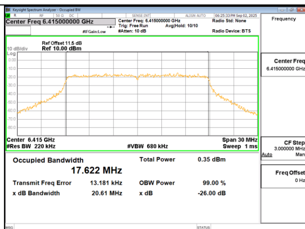
802.11ac 20MHz Chain0 6415MHz
