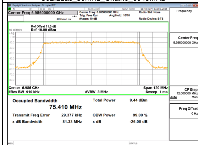
802.11ac 80MHz Chain1 5985MHz
