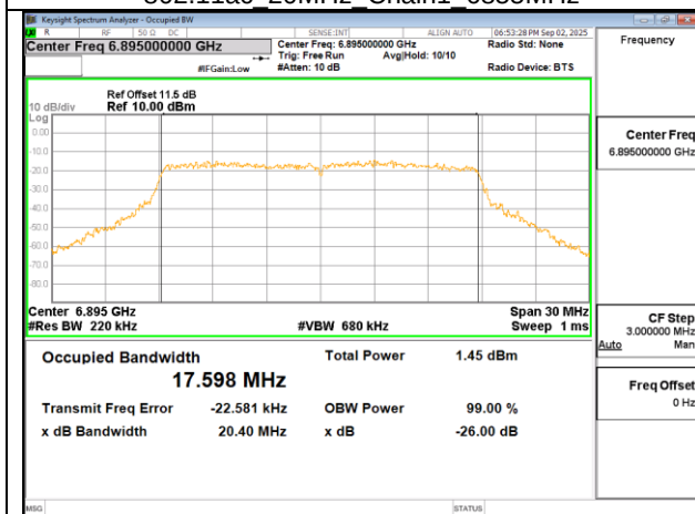
802.11ac 20MHz Chain1 6895MHz
