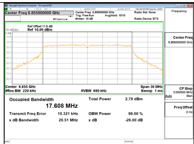
802.11ac 20MHz Chain0 6855MHz
