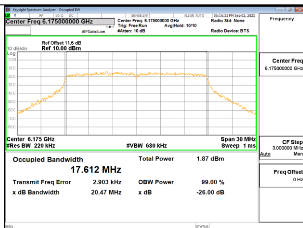
802.11ac 20MHz Chain1 6175MHz
