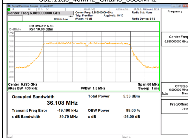
802.11ac 40MHz Chain0 6885MHz
