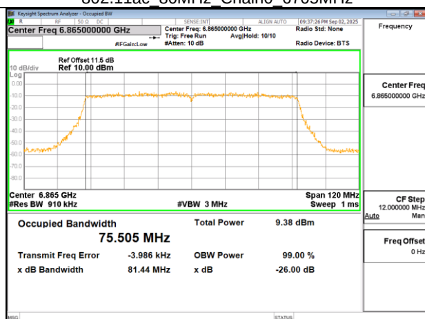
802.11ac 80MHz Chain0 6865MHz
