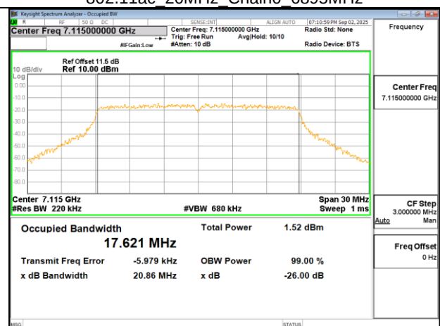
802.11ac 20MHz Chain0 7115MHz
