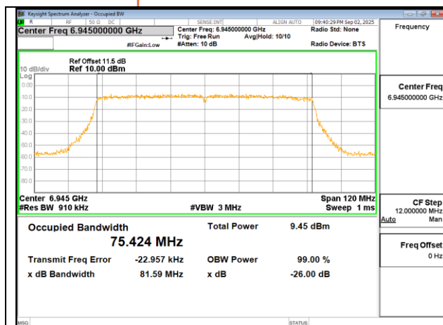
802.11ac 80MHz Chain0 6945MHz
