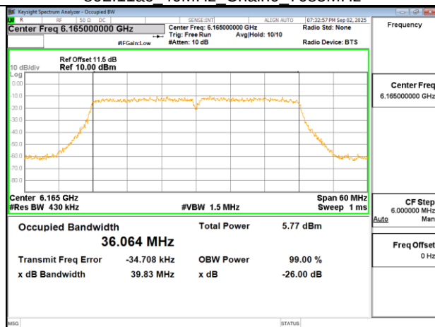
802.11ac 40MHz Chain1 6165MHz
