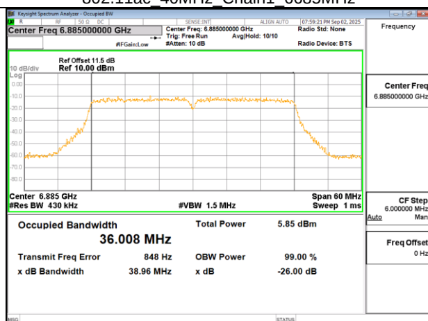
802.11ac 40MHz Chain1 6885MHz
