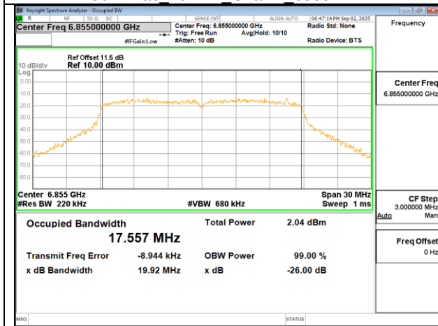
802.11ac 20MHz Chain1 6855MHz
