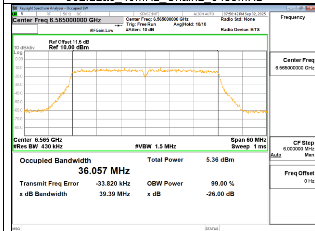
802.11ac 40MHz Chain1 6565MHz
