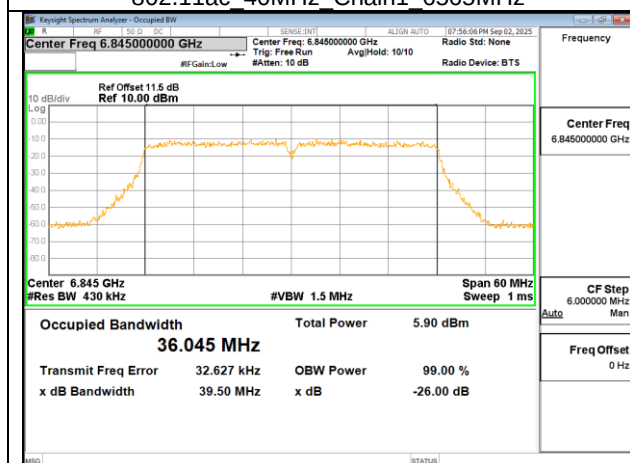
802.11ac 40MHz Chain1 6845MHz
