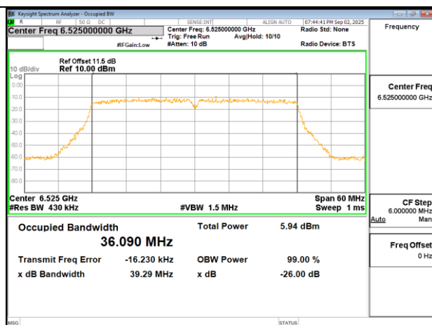
802.11ac 40MHz Chain1 6525MHz
