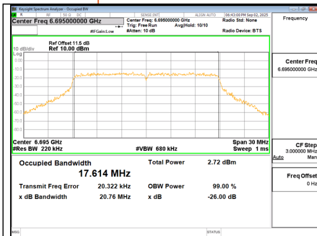
802.11ac 20MHz Chain0 6695MHz
