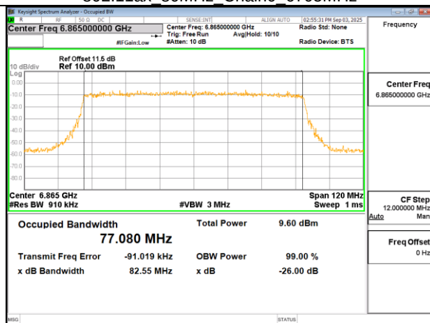
802.11ax 80MHz Chain0 6865MHz
