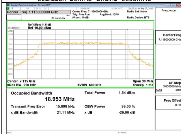
802.11ax 20MHz Chain1 7115MHz
