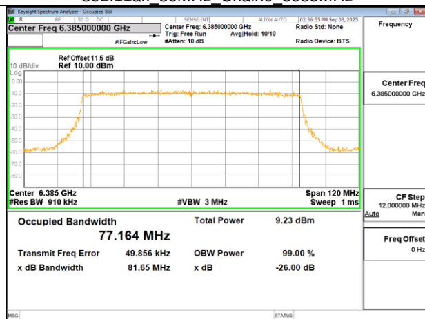
802.11ax 80MHz Chain0 6385MHz
