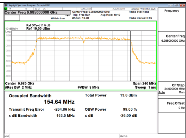
802.11ac 160MHz Chain0 6985MHz
