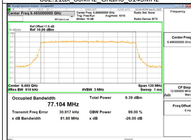
802.11ax 80MHz Chain0 6465MHz
