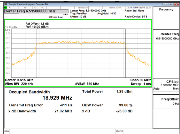
802.11ax 20MHz Chain1 6515MHz
