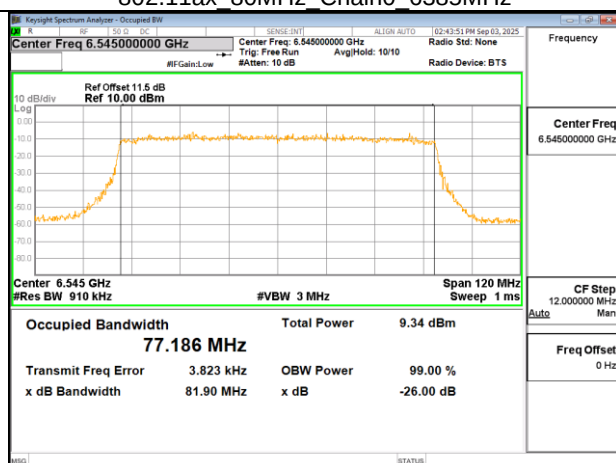
802.11ax 80MHz Chain0 6545MHz
