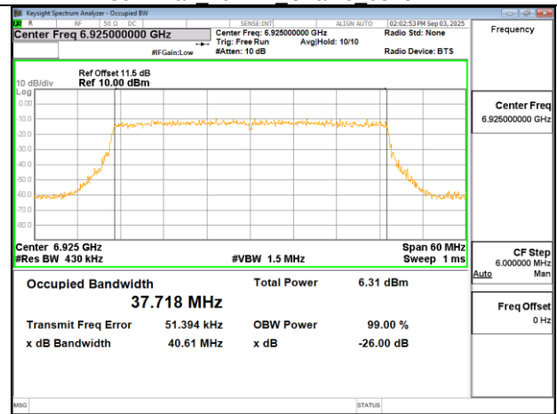
802.11ax 40MHz Chain0 6925MHz
