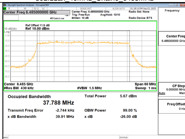
802.11ax 40MHz Chain0 6485MHz
