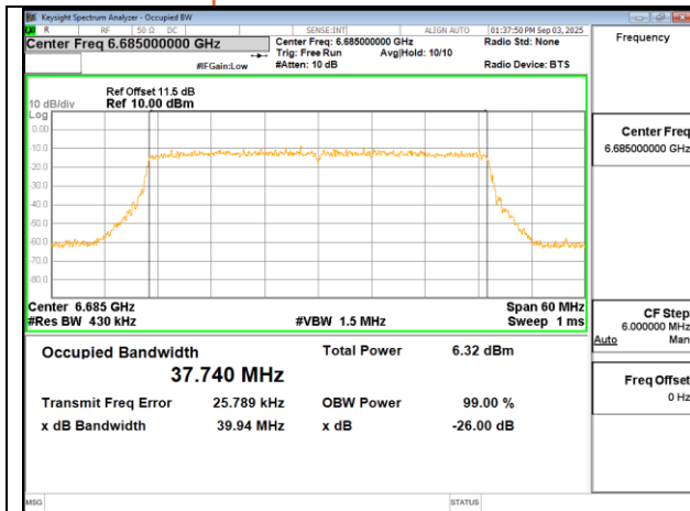
802.11ax 40MHz Chain0 6685MHz
