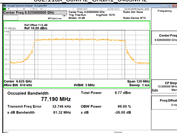
802.11ax 80MHz Chain1 6625MHz
