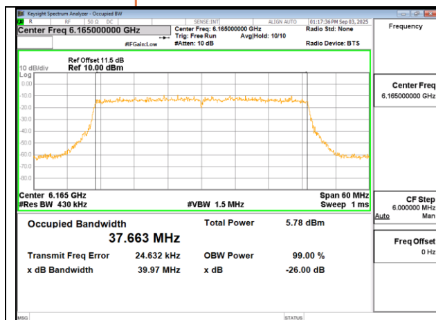
802.11ax 40MHz Chain0 6165MHz
