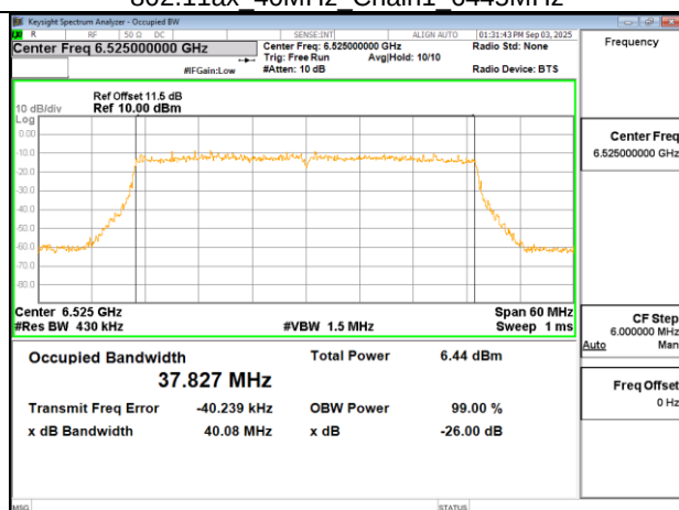
802.11ax 40MHz Chain1 6525MHz
