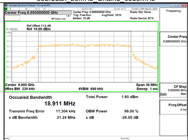
802.11ax 20MHz Chain1 6695MHz
