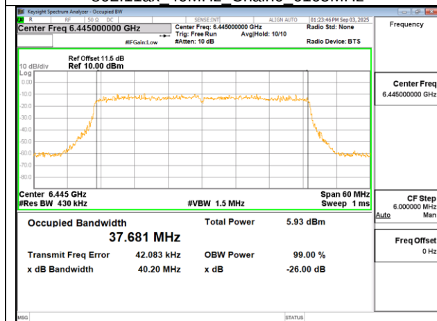
802.11ax 40MHz Chain0 6445MHz
