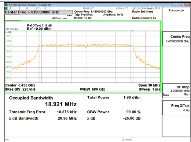
802.11ax 20MHz Chain1 6435MHz
