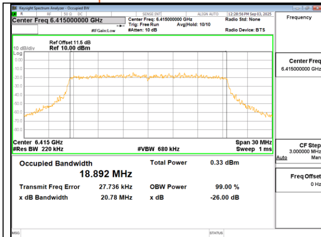
802.11ax 20MHz Chain1 6415MHz
