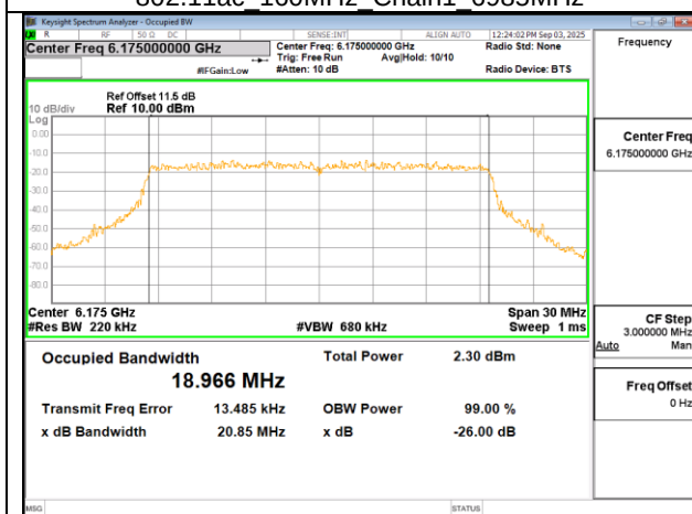
802.11ax 20MHz Chain0 6175MHz
