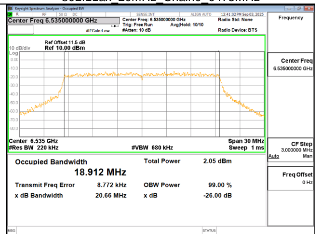
802.11ax 20MHz Chain0 6535MHz
