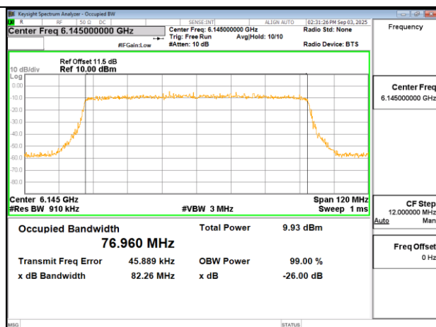
802.11ax 80MHz Chain1 6145MHz
