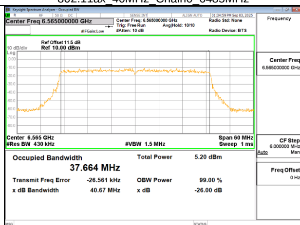
802.11ax 40MHz Chain0 6565MHz
