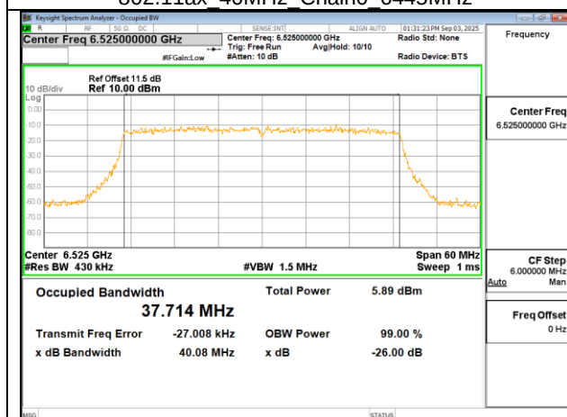
802.11ax 40MHz Chain0 6525MHz
