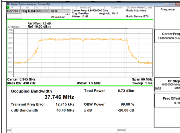
802.11ax 40MHz Chain1 6845MHz
