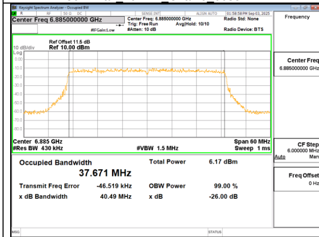
802.11ax 40MHz Chain0 6885MHz
