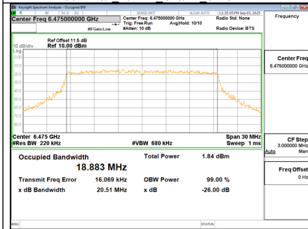
802.11ax 20MHz Chain1 6475MHz
