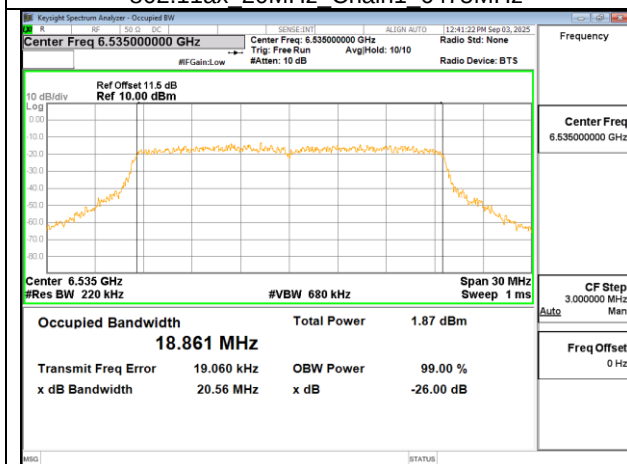
802.11ax 20MHz Chain1 6535MHz
