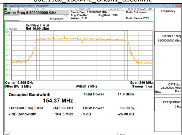
802.11ac 160MHz Chain1 6505MHz
