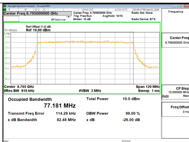
802.11ax 80MHz Chain0 6705MHz
