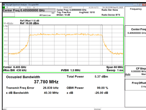
802.11ax 40MHz Chain0 6405MHz
