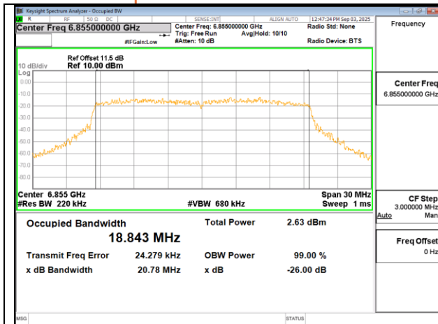
802.11ax 20MHz Chain1 6855MHz
