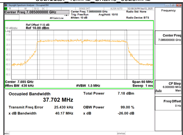
802.11ax 40MHz Chain0 7085MHz
