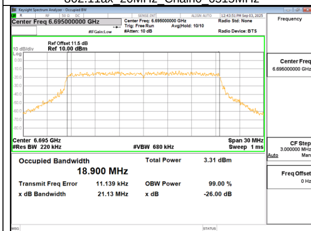
802.11ax 20MHz Chain0 6695MHz
