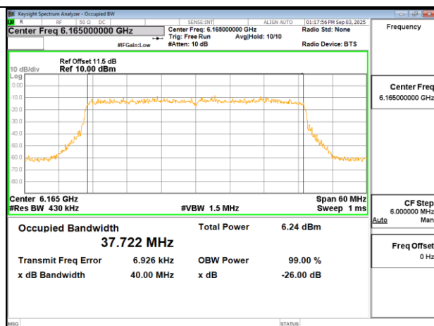
802.11ax 40MHz Chain1 6165MHz
