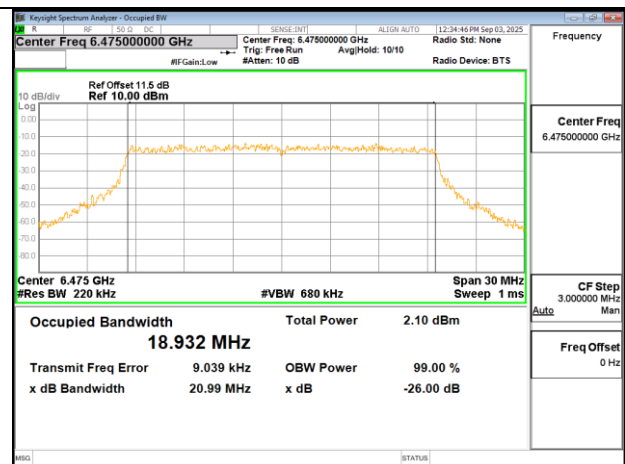
802.11ax 20MHz Chain0 6475MHz
