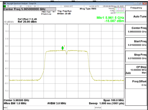
802.11n 40MHz Chain0 5965MHz
