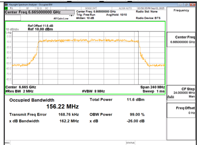
802.11ax 160MHz Chain0 6665MHz
