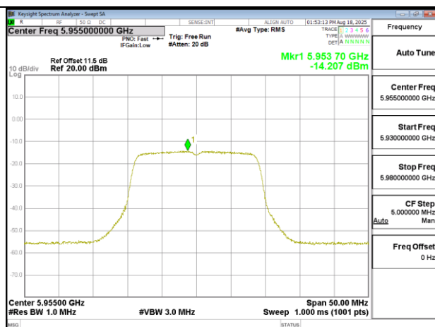
802.11n 20MHz Chain0 5955MHz
