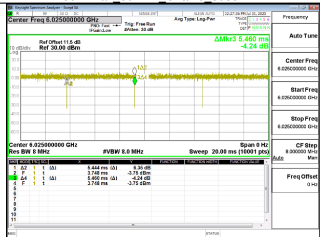
802.11ax 160MHz Chain0 6025MHz
