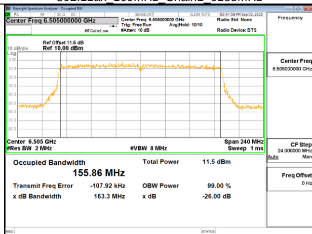
802.11ax 160MHz Chain1 6505MHz
