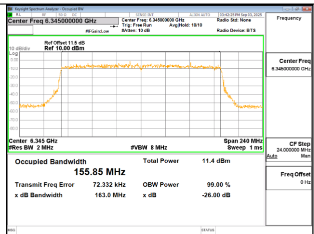
802.11ax 160MHz Chain0 6345MHz
