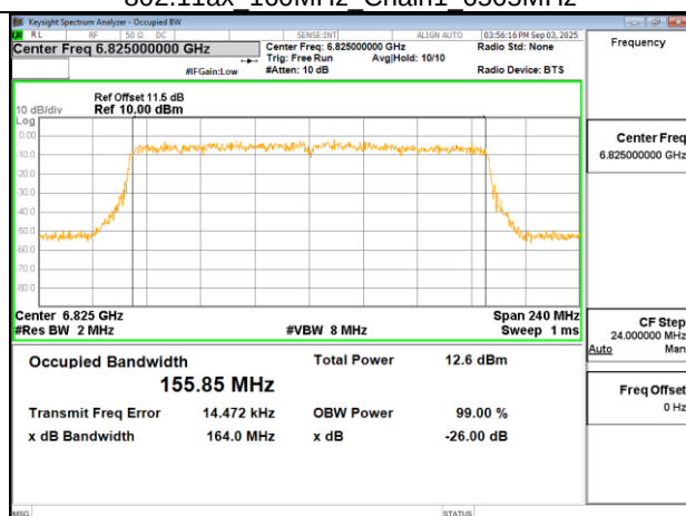
802.11ax 160MHz Chain1 6825MHz
