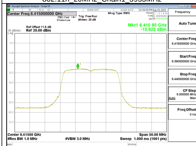
802.11n 20MHz Chain1 6415MHz
