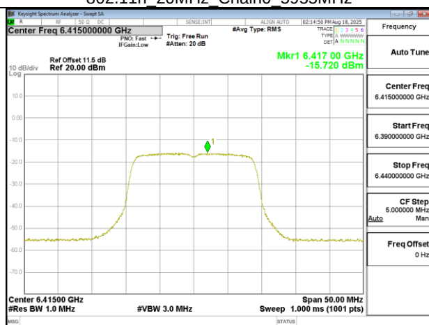
802.11n 20MHz Chain0 6415MHz
