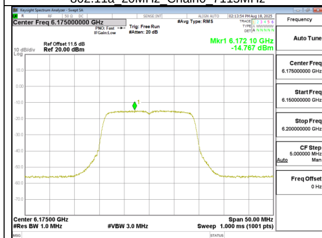
802.11n 20MHz Chain0 6175MHz
