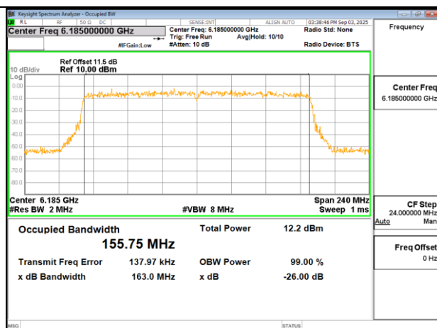
802.11ax 160MHz Chain1 6185MHz
