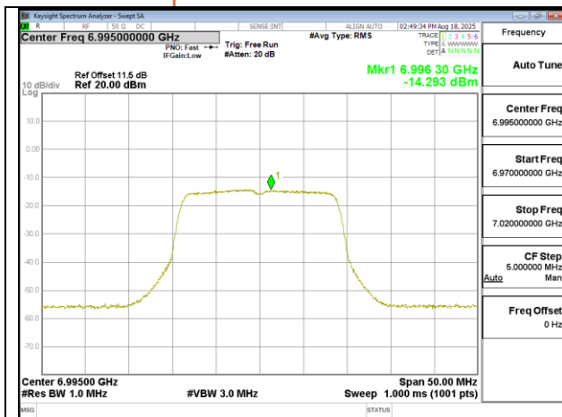
802.11n 20MHz Chain0 6995MHz
