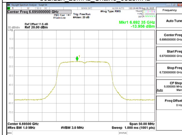
802.11n 20MHz Chain0 6695MHz
