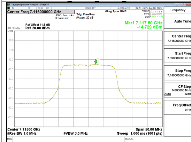
802.11n 20MHz Chain1 7115MHz
