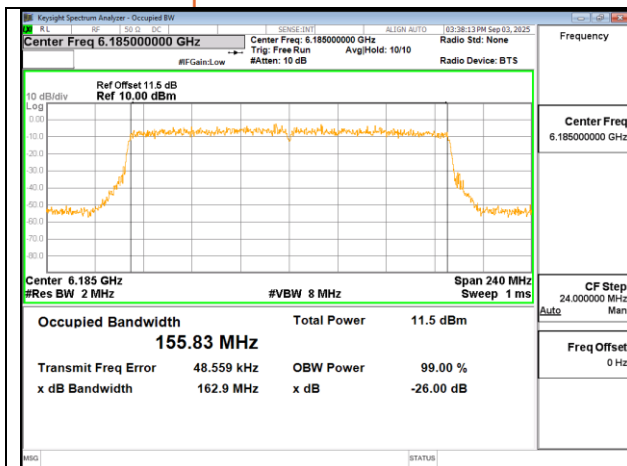
802.11ax 160MHz Chain0 6185MHz
