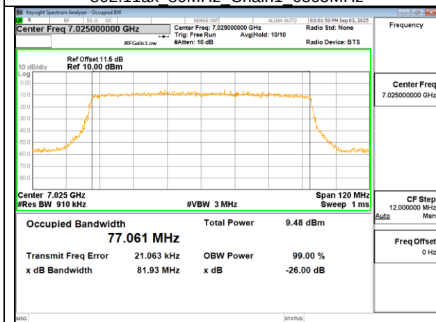
802.11ax 80MHz Chain1 7025MHz
