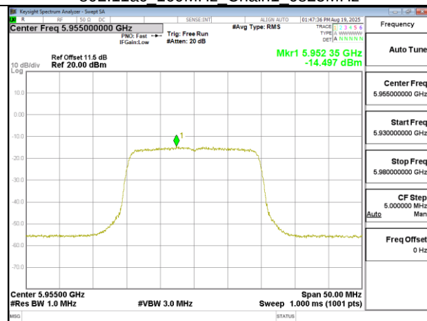
802.11ax 20MHz Chain0 5955MHz
