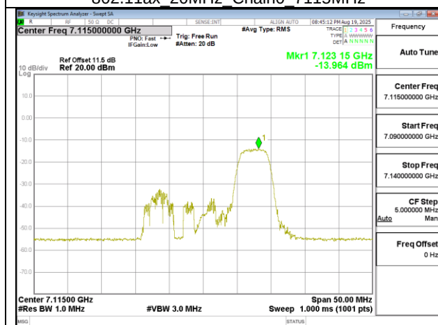
802.11ax 20MHz Chain0 7115MHz RU52 40
