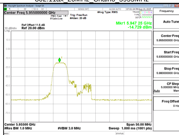
802.11ax 20MHz Chain0 5955MHz RU52 37
