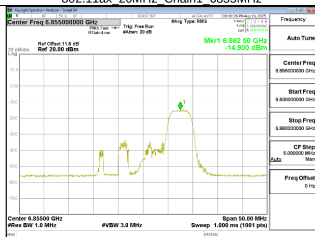
802.11ax 20MHz Chain1 6855MHz RU52 40
