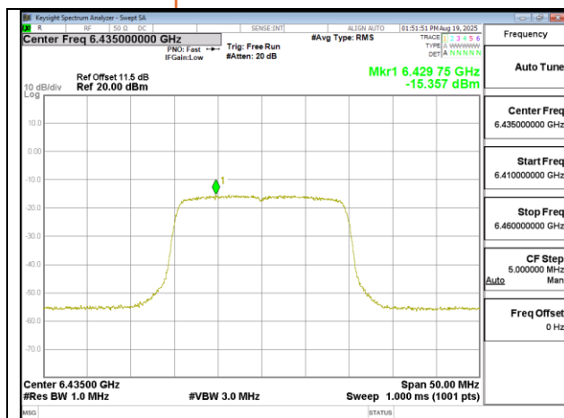
802.11ax 20MHz Chain0 6435MHz
