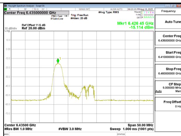
802.11ax 20MHz Chain0 6435MHz RU26 0
