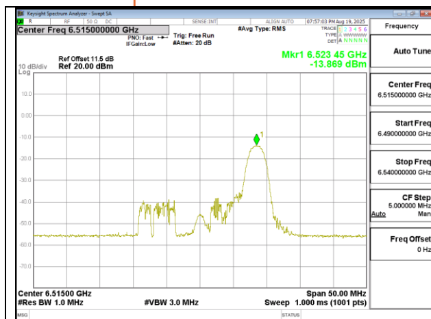
802.11ax 20MHz Chain0 6515MHz RU26 8
