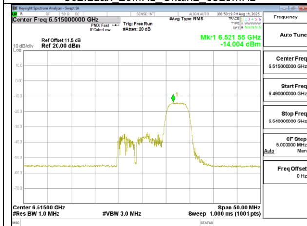
802.11ax 20MHz Chain1 6515MHz RU52 40
