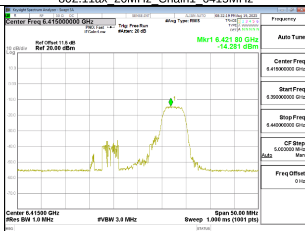
802.11ax 20MHz Chain1 6415MHz RU52 40
