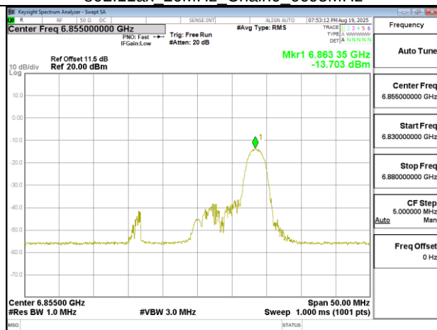
802.11ax 20MHz Chain0 6855MHz RU26 8
