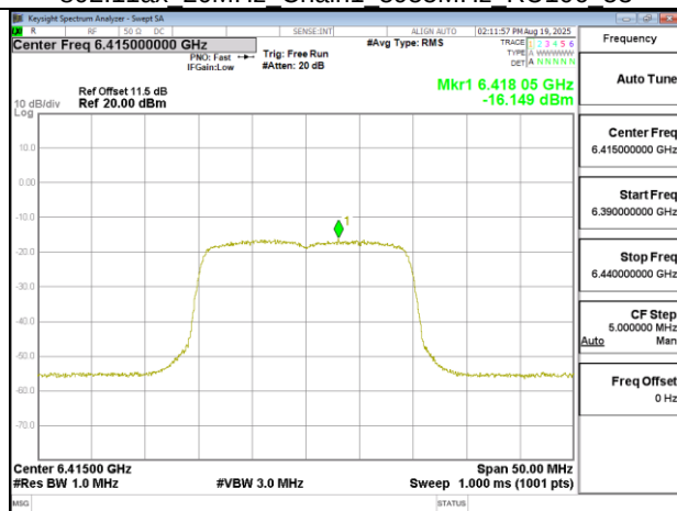
802.11ax 20MHz Chain1 6415MHz
