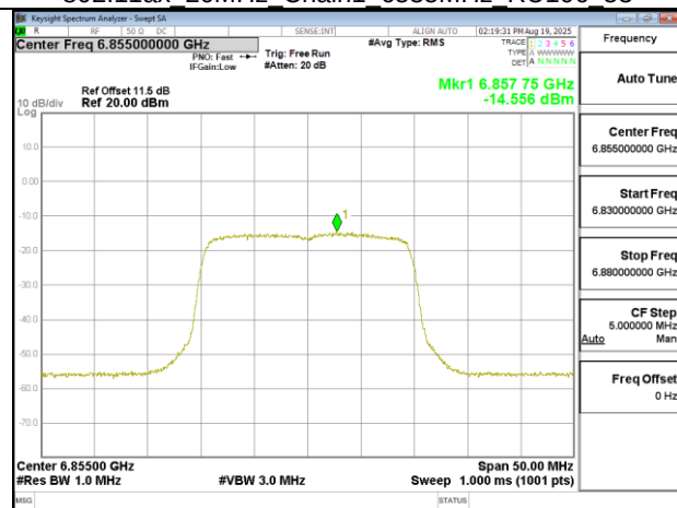
802.11ax 20MHz Chain1 6855MHz
