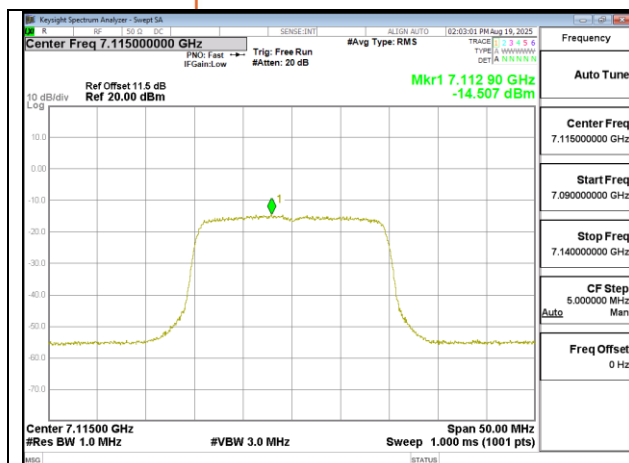
802.11ax 20MHz Chain0 7115MHz
