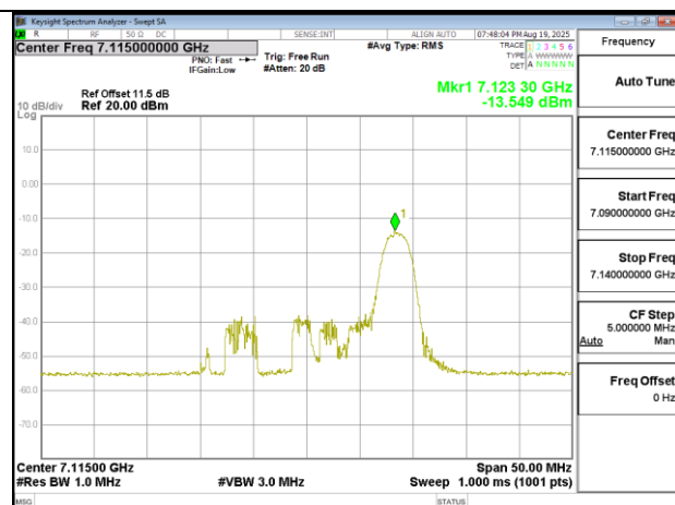
802.11ax 20MHz Chain0 7115MHz RU26 8
