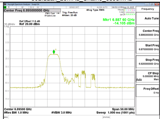
802.11ax 20MHz Chain0 6895MHz RU52 37
