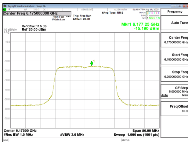
802.11ax 20MHz Chain0 6175MHz
