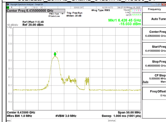
802.11ax 20MHz Chain1 6435MHz RU26 0
