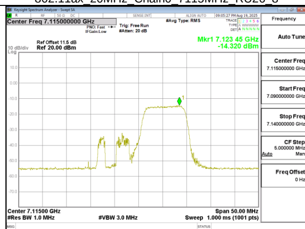
802.11ax 20MHz Chain0 7115MHz RU106 54
