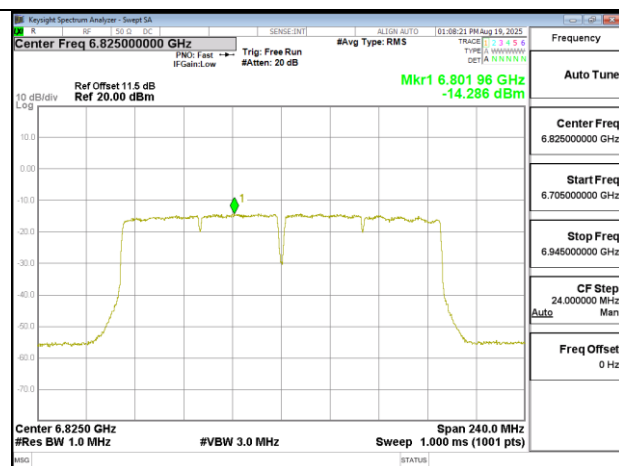
802.11ac 160MHz Chain1 6825MHz
