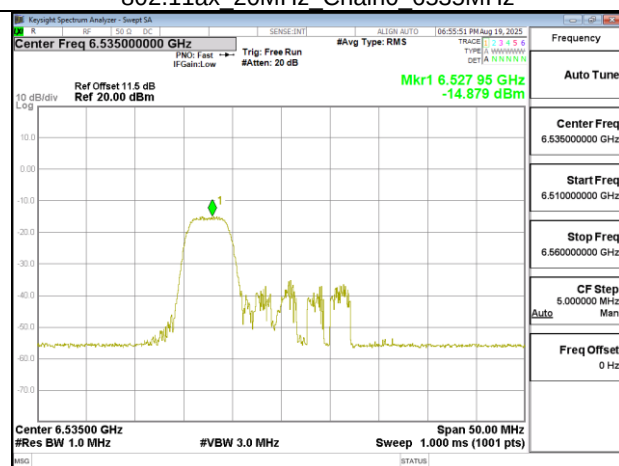
802.11ax 20MHz Chain0 6535MHz RU52 37
