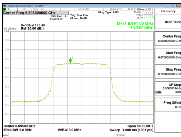
802.11ax 20MHz Chain0 6695MHz
