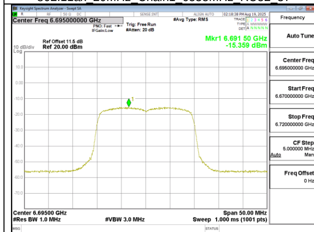
802.11ax 20MHz Chain1 6695MHz
