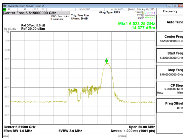
802.11ax 20MHz Chain1 6515MHz RU26 8
