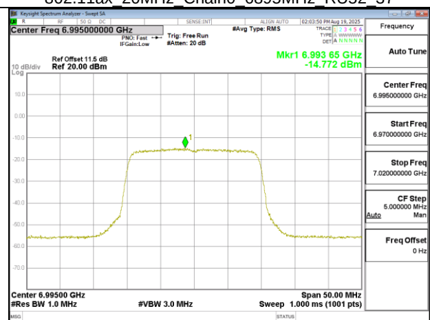
802.11ax 20MHz Chain0 6995MHz
