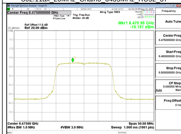
802.11ax 20MHz Chain0 6475MHz
