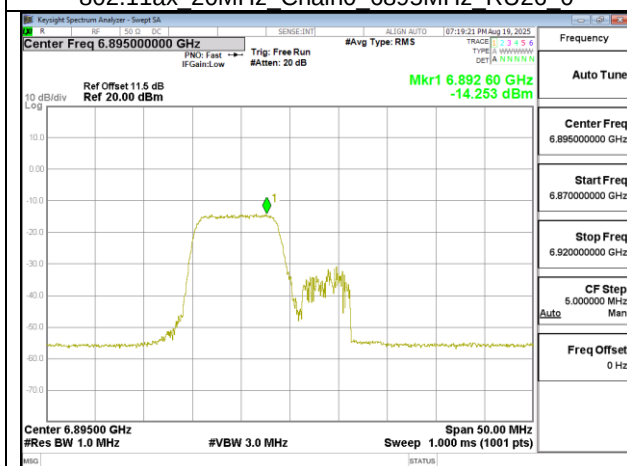
802.11ax 20MHz Chain0 6895MHz RU106 53
