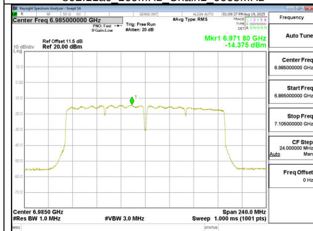
802.11ac 160MHz Chain1 6985MHz
