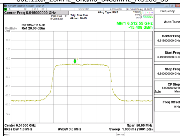
802.11ax 20MHz Chain0 6515MHz
