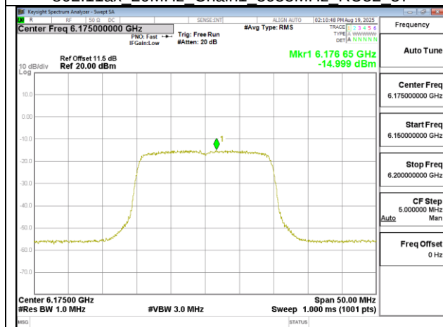
802.11ax 20MHz Chain1 6175MHz
