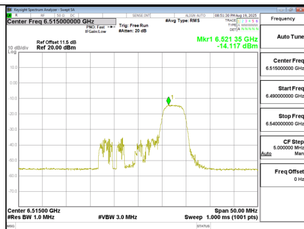
802.11ax 20MHz Chain0 6515MHz RU52 40
