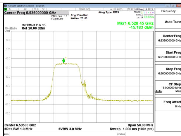
802.11ax 20MHz Chain1 6535MHz RU106 53
