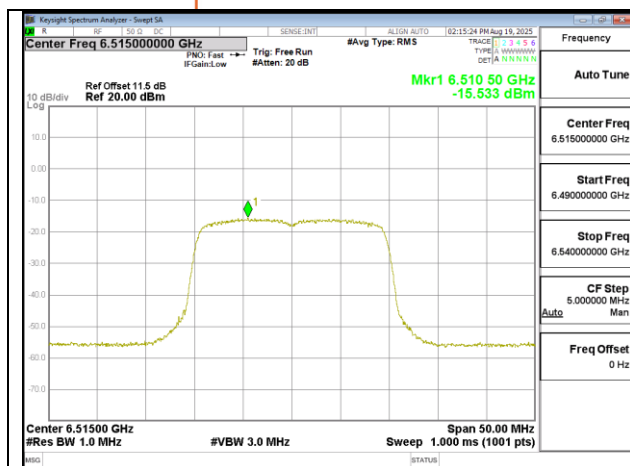
802.11ax 20MHz Chain1 6515MHz
