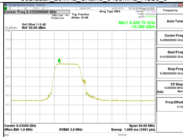
802.11ax 20MHz Chain0 6435MHz RU106 53
