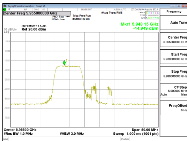
802.11ax 20MHz Chain1 5955MHz RU106 53
