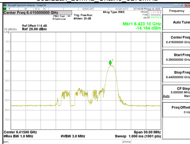
802.11ax 20MHz Chain0 6415MHz RU26 8
