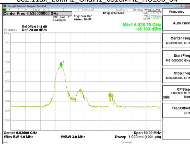
802.11ax 20MHz Chain1 6535MHz RU26 0
