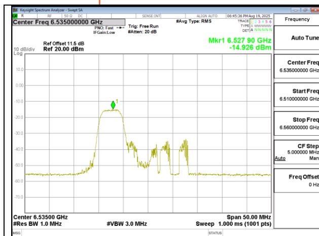
802.11ax 20MHz Chain1 6535MHz RU52 37
