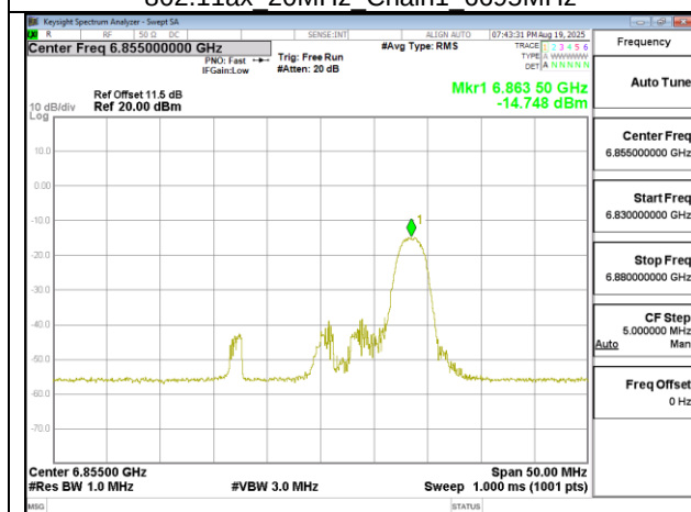
802.11ax 20MHz Chain1 6855MHz RU26 8
