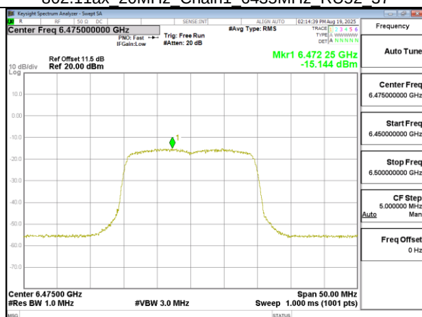
802.11ax 20MHz Chain1 6475MHz
