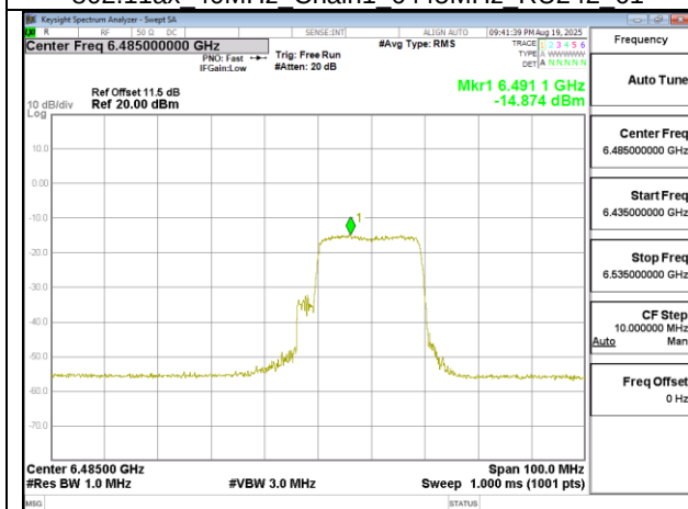
802.11ax 40MHz Chain1 6485MHz RU242 62
