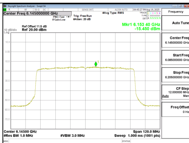
802.11ax 80MHz Chain0 6145MHz
