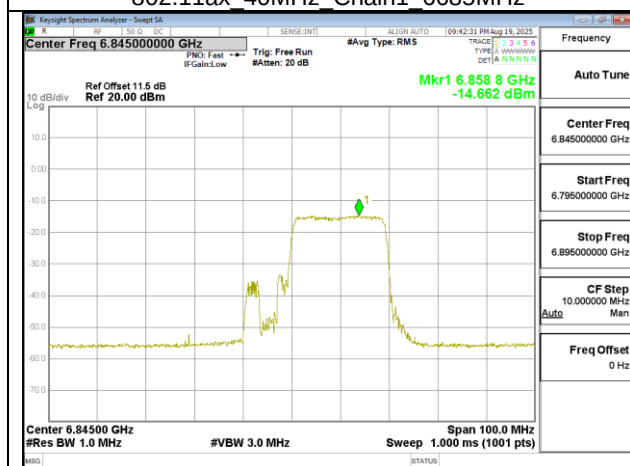
802.11ax 40MHz Chain1 6845MHz RU242 62
