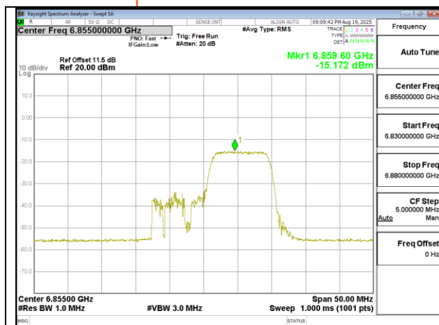
802.11ax 20MHz Chain1 6855MHz RU106 54
