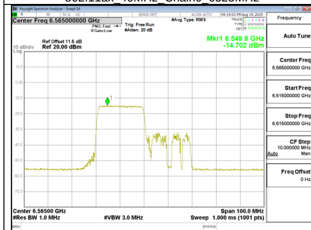
802.11ax 40MHz Chain0 6565MHz RU242 61
