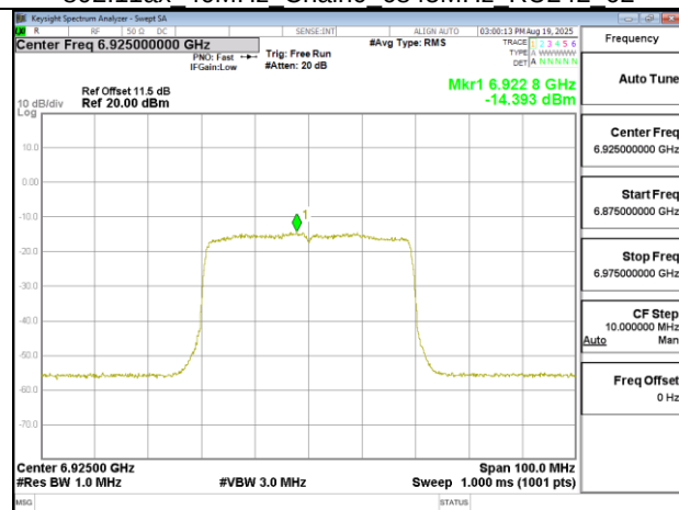
802.11ax 40MHz Chain0 6925MHz
