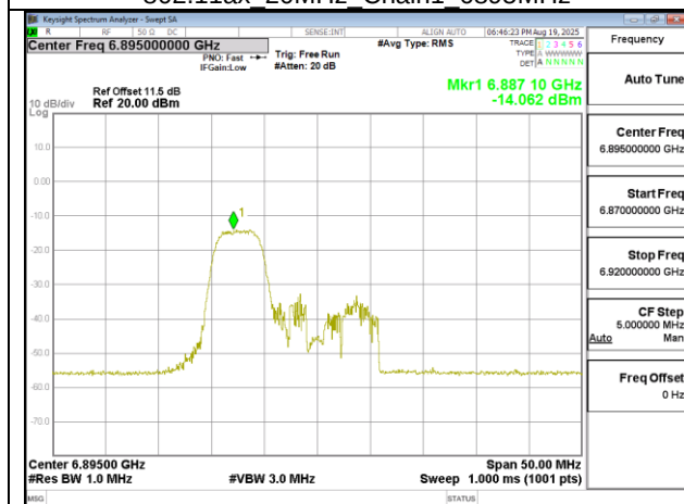
802.11ax 20MHz Chain1 6895MHz RU52 37
