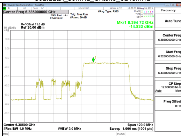
802.11ax 80MHz Chain0 6385MHz RU484 66
