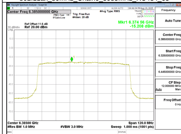
802.11ax 80MHz Chain0 6385MHz
