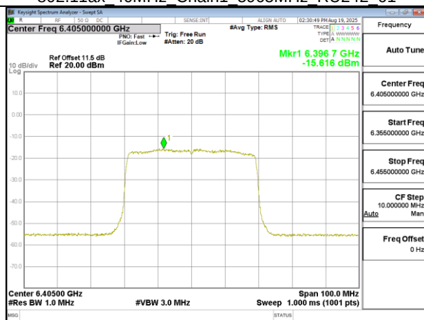
802.11ax 40MHz Chain1 6405MHz
