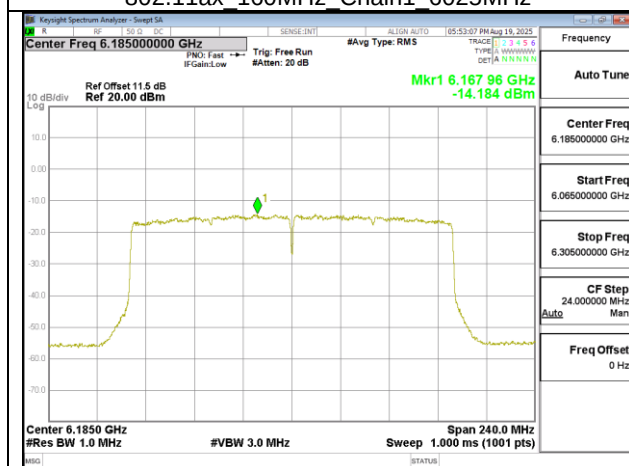
802.11ax 160MHz Chain1 6185MHz
