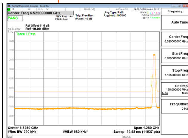
802.11a 20MHz Chain1 7115MHz
