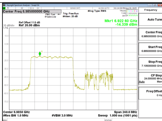
802.11ax 160MHz Chain1 6985MHz RU996_67
