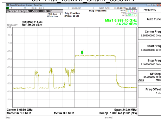
802.11ax 160MHz Chain1 6985MHz RU996_S67
