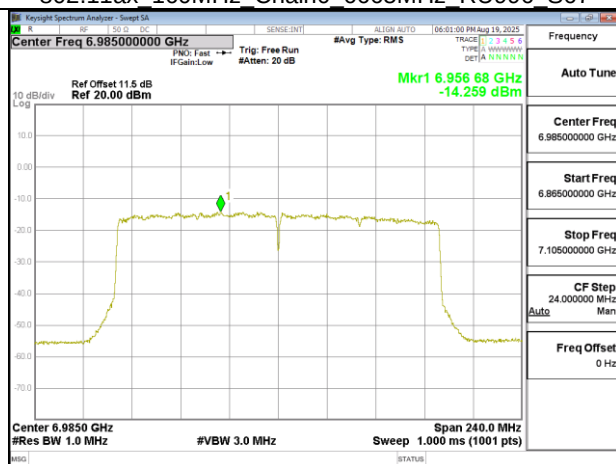
802.11ax 160MHz Chain0 6985MHz
