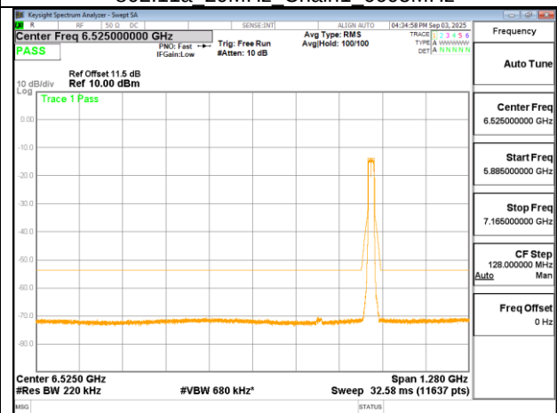
802.11a 20MHz Chain1 6875MHz
