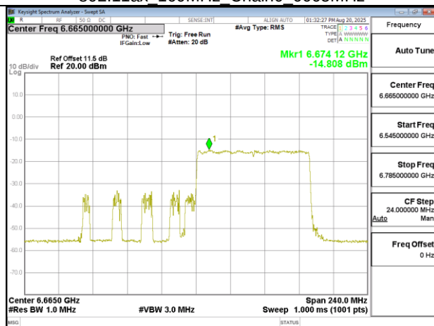
802.11ax 160MHz Chain0 6665MHz RU996 S67
