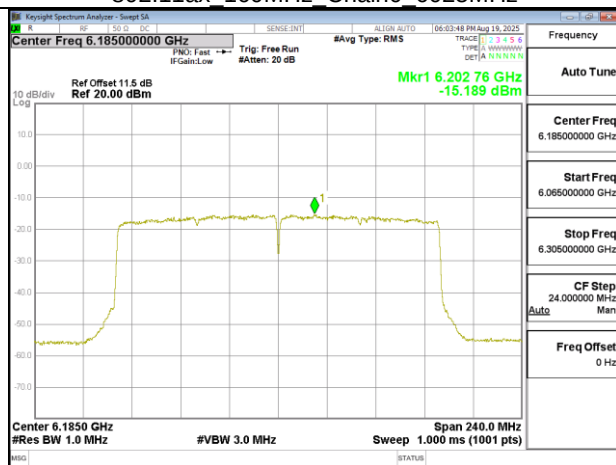
802.11ax 160MHz Chain0 6185MHz
