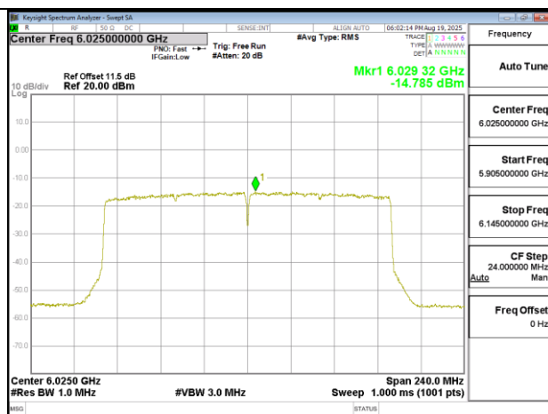
802.11ax 160MHz Chain0 6025MHz
