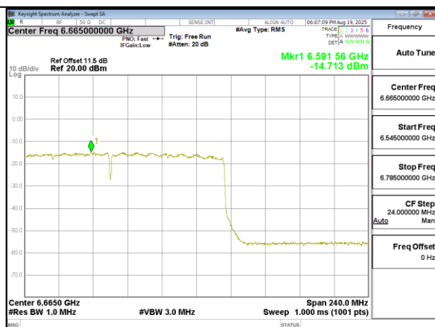
802.11ax 160MHz Chain0 6665MHz
