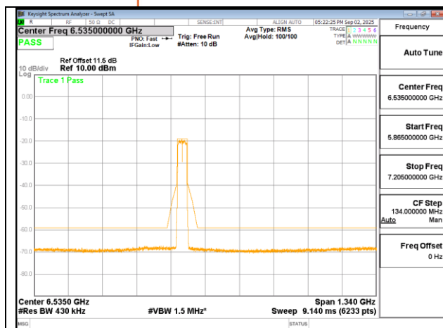
802.11n 40MHz Chain0 6445MHz
