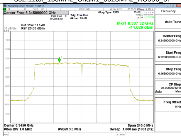
802.11ax 160MHz Chain1 6345MHz
