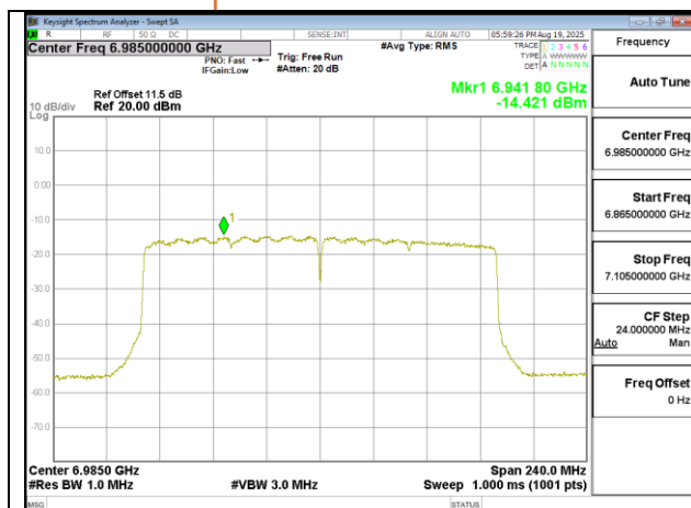
802.11ax 160MHz Chain1 6985MHz
