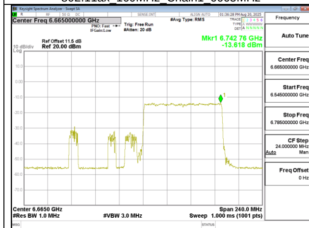
802.11ax 160MHz Chain1 6665MHz RU996_S67
