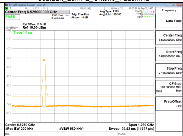
802.11n 20MHz Chain1 6175MHz
