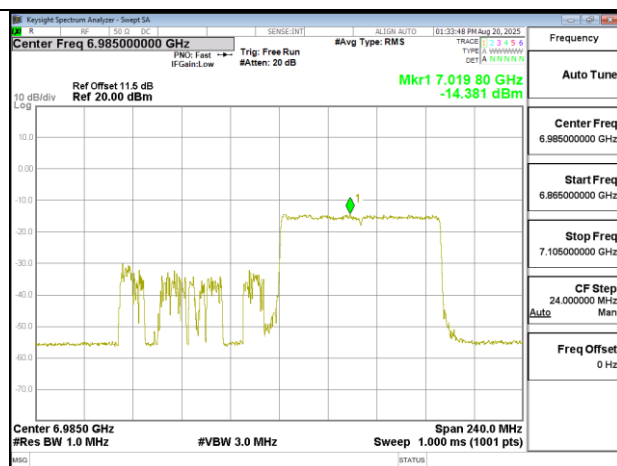
802.11ax 160MHz Chain0 6985MHz RU996 S67
