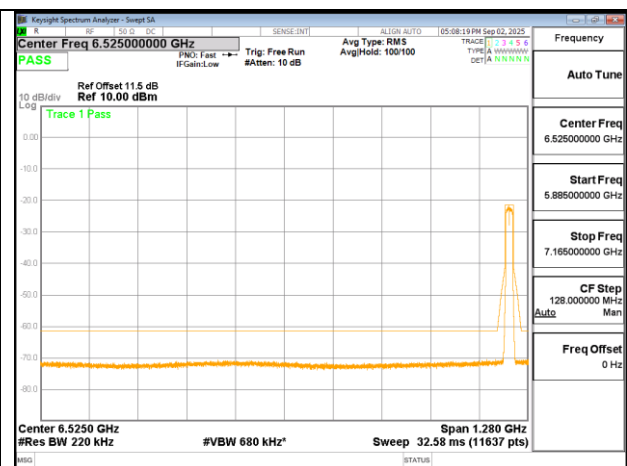
802.11n 20MHz Chain0 7115MHz
