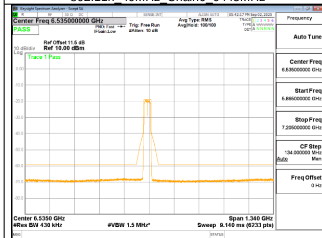
802.11n 40MHz Chain0 6525MHz
