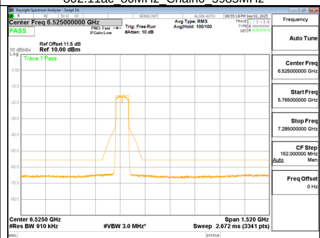
802.11ac 80MHz Chain0 6385MHz
