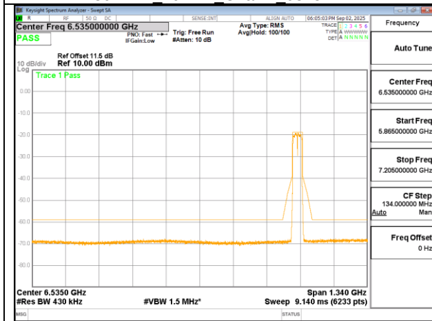
802.11n 40MHz Chain1 6925MHz
