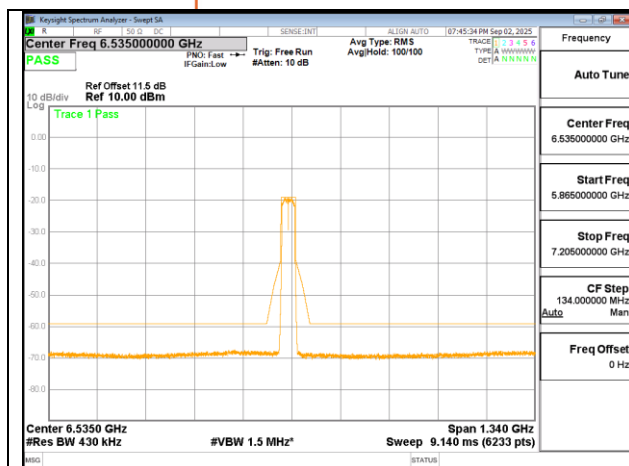
802.11ac 40MHz Chain0 6525MHz
