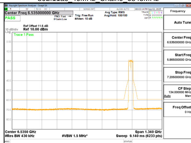
802.11ac 40MHz Chain0 6865MHz
