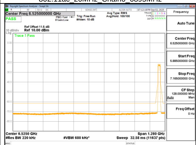
802.11ac 20MHz Chain0 7115MHz
