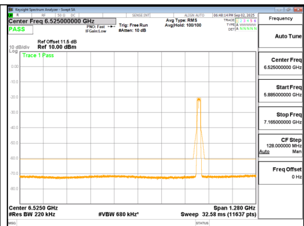
802.11ac 20MHz Chain0 6855MHz
