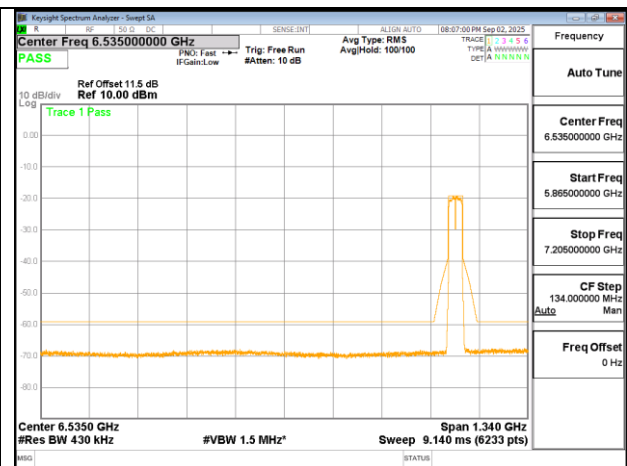
802.11ac 40MHz Chain1 7005MHz
