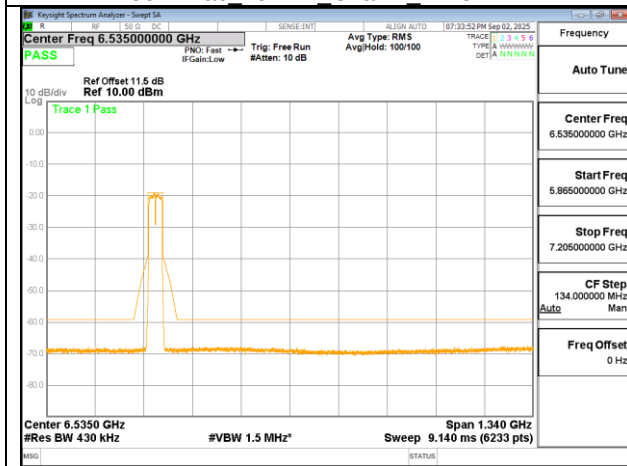
802.11ac 40MHz Chain0 6165MHz
