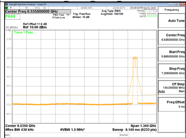
802.11n 40MHz Chain1 7005MHz
