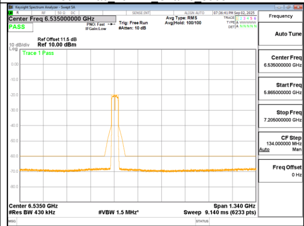
802.11ac 40MHz Chain0 6405MHz
