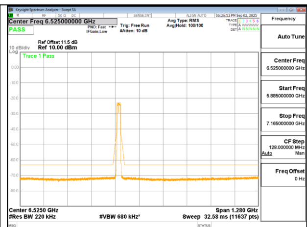
802.11ac 20MHz Chain0 6415MHz
