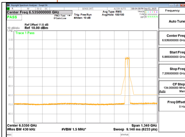
802.11ac 40MHz Chain1 6925MHz
