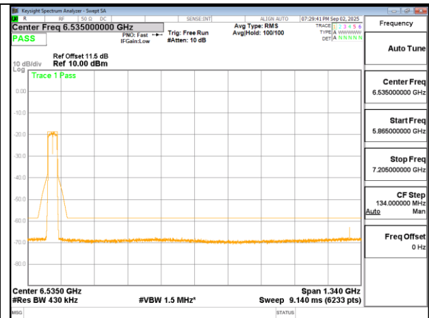
802.11ac 40MHz Chain0 5965MHz
