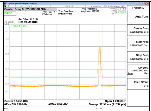
802.11ac 20MHz Chain1 6875MHz
