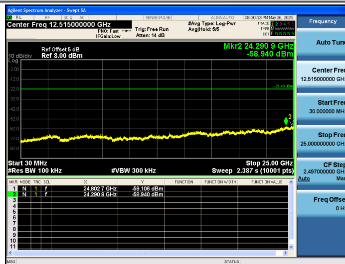
BLE_2480_30~25000
