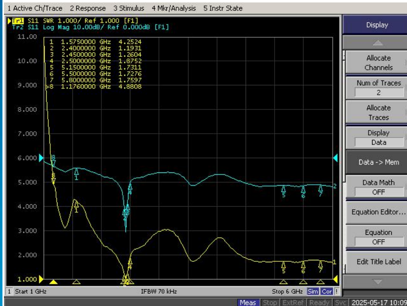
驻波图
