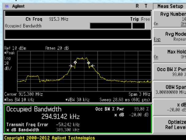
915.3MHz
