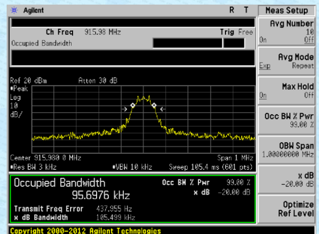
915.98MHz
