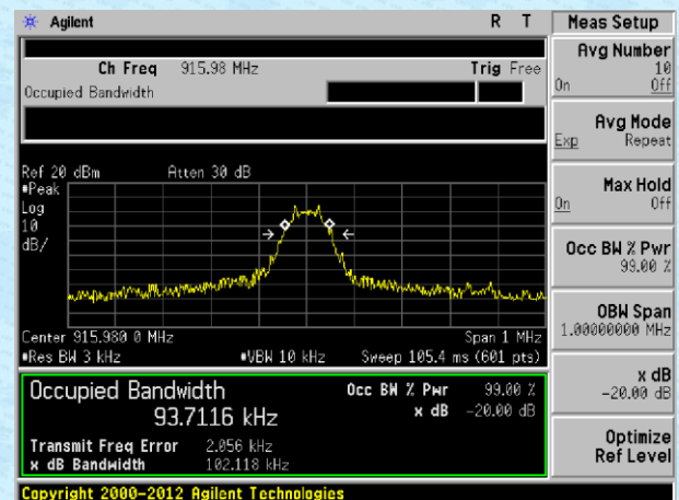
915.98MHz
