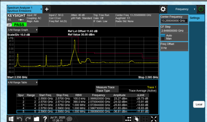
Band7-20MHz-QPSK-21350-1RB#99-PASS
