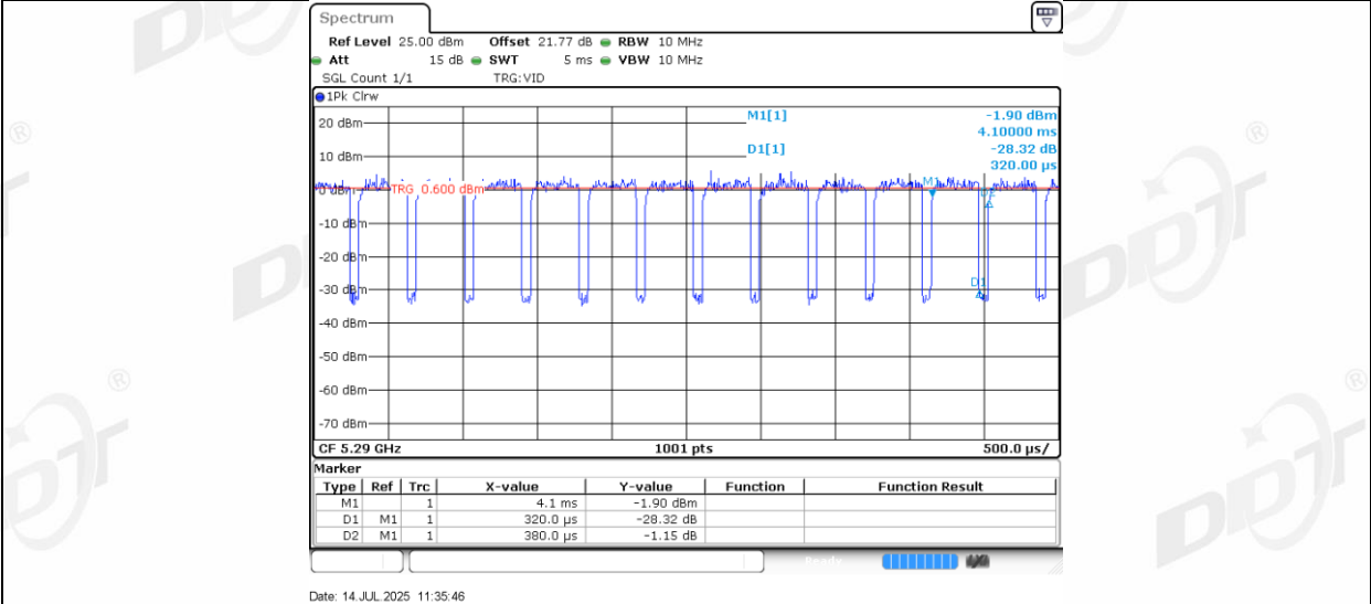
11AC80MIMO_Ant2_5290
