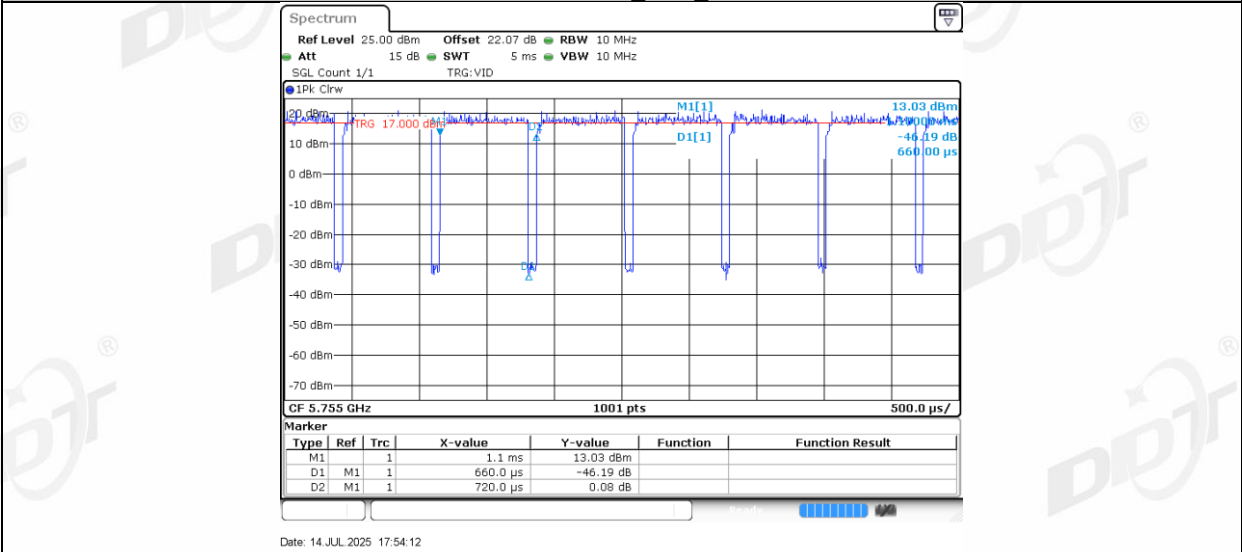
11AC40MIMO_Ant2_5755
