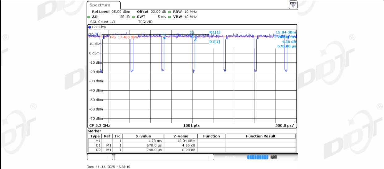
11N20MIMO_Ant2_5200
