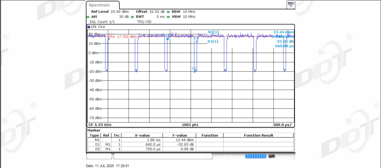
11AC40MIMO_Ant2_5230
