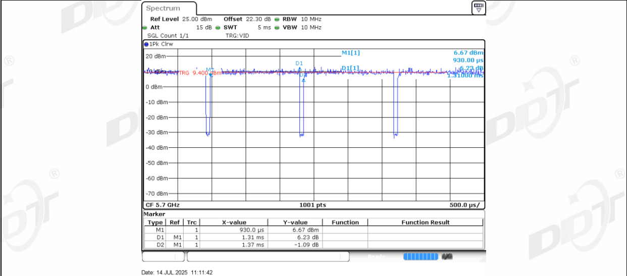
11AC20MIMO_Ant1_5745
