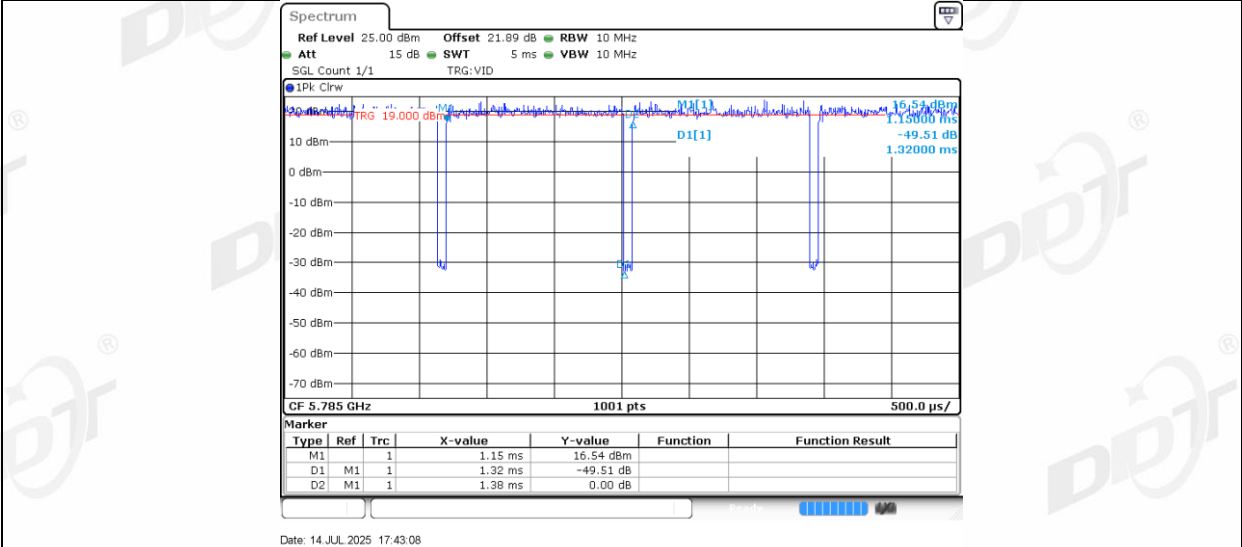
11AC20MIMO_Ant2_5785
