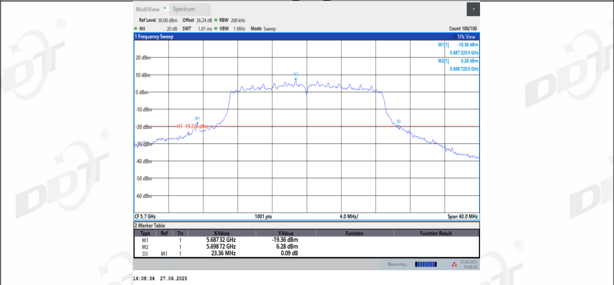
11N20_Ant3_5700
