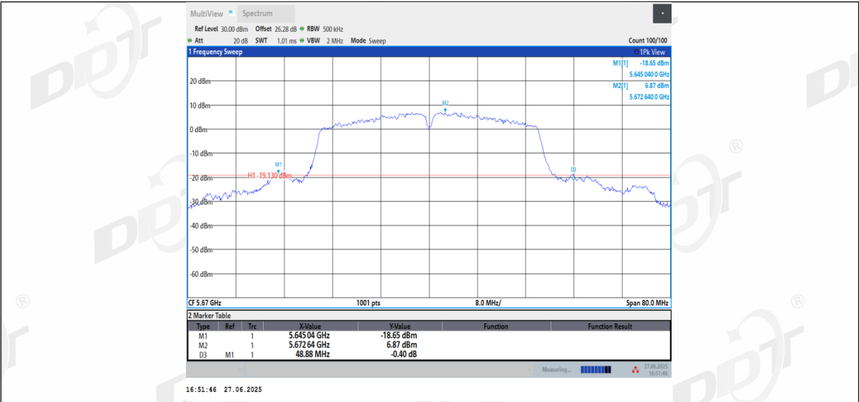
11N40_Ant2_5670
