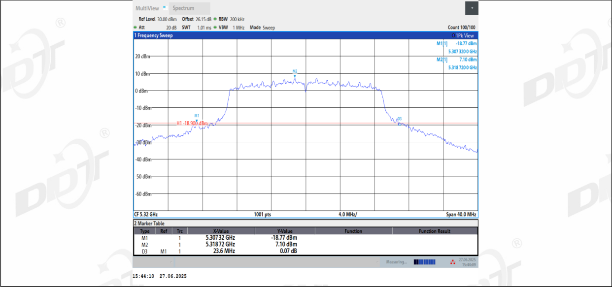
11N20_Ant3_5320
