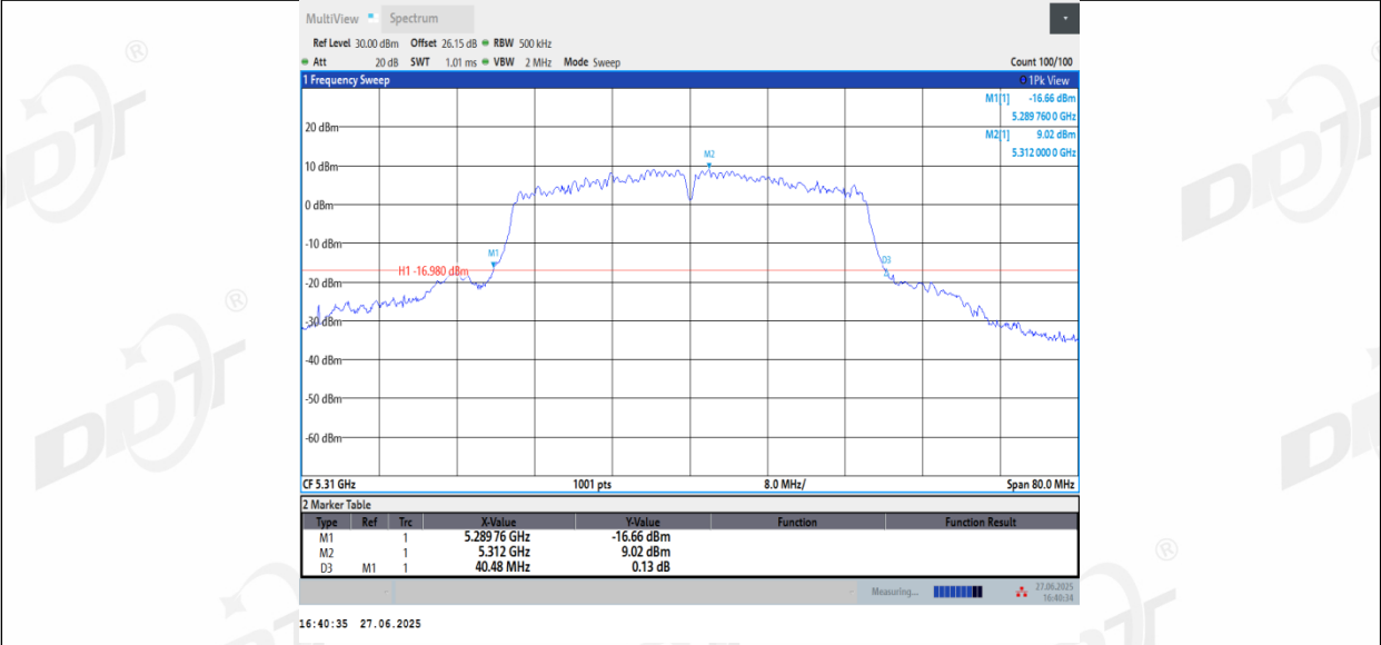
11N40_Ant3_5310
