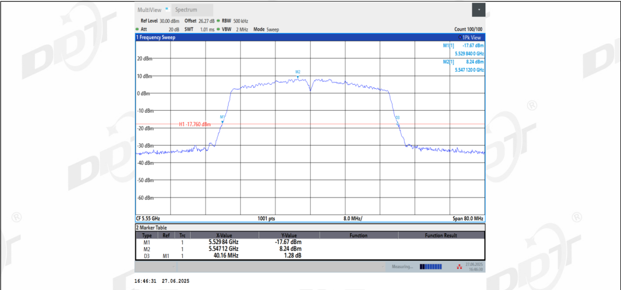
11N40_Ant2_5550
