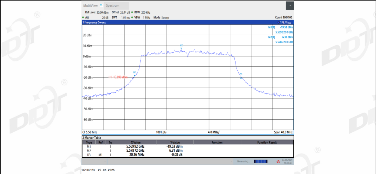
11N20_Ant3_5580
