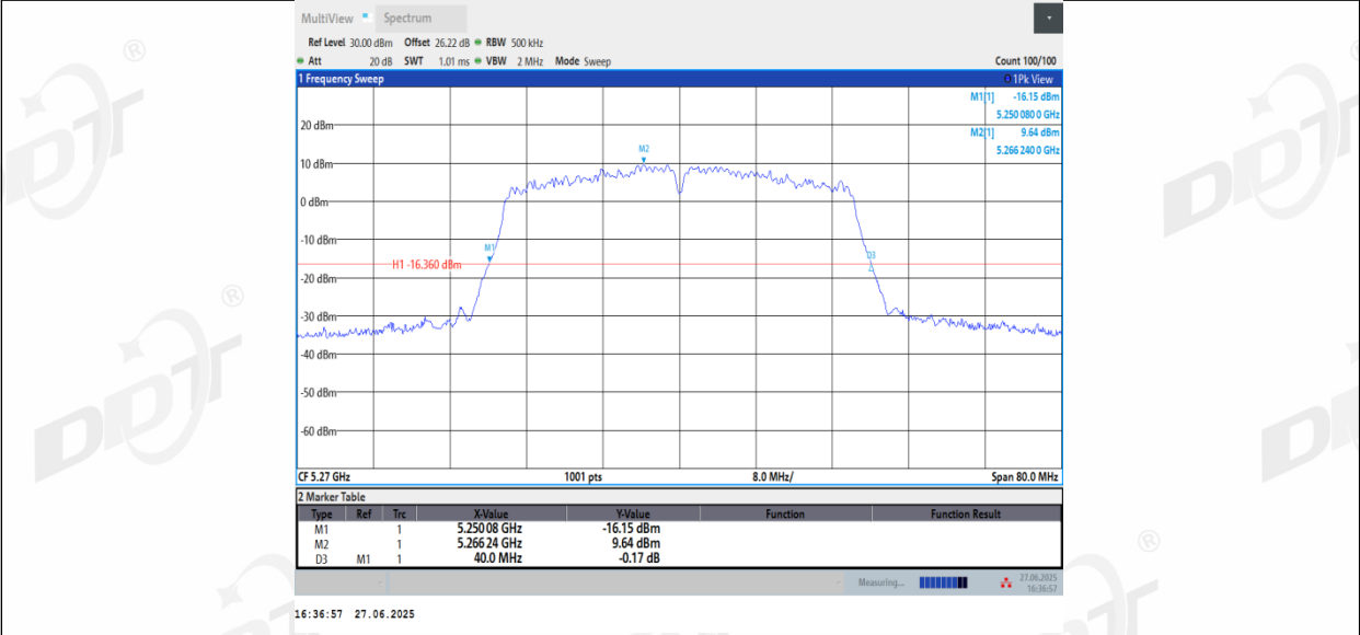
11N40_Ant3_5270
