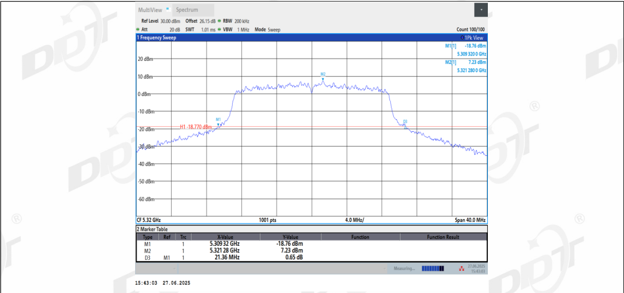
11N20_Ant2_5320
