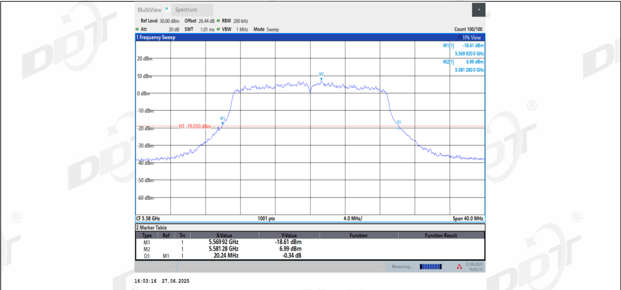
11N20_Ant2_5580
