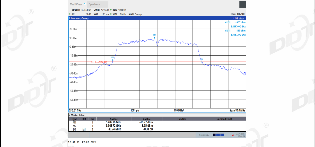
11N40_Ant3_5510
