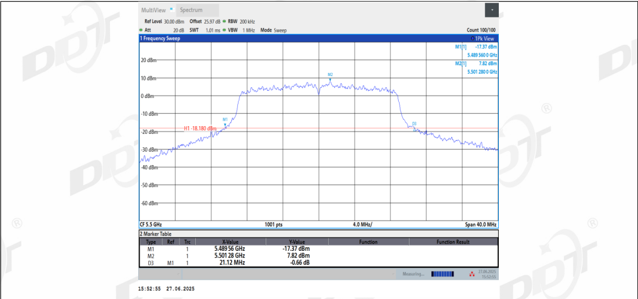
11N20_Ant2_5500
