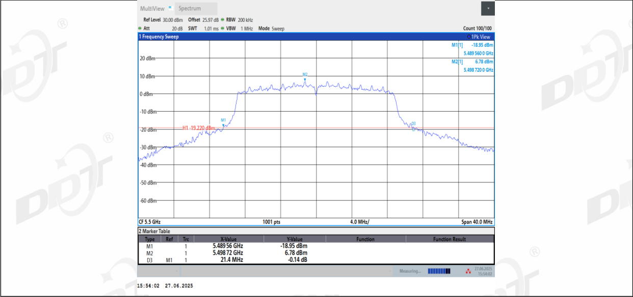
11N20_Ant3_5500
