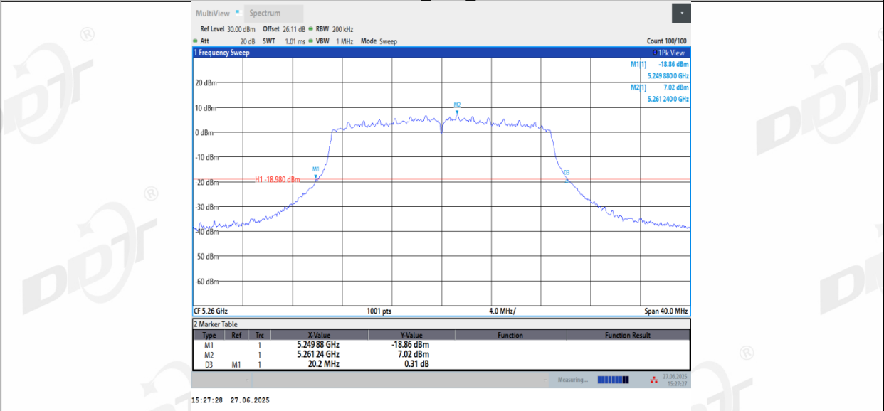
11N20_Ant3_5260
