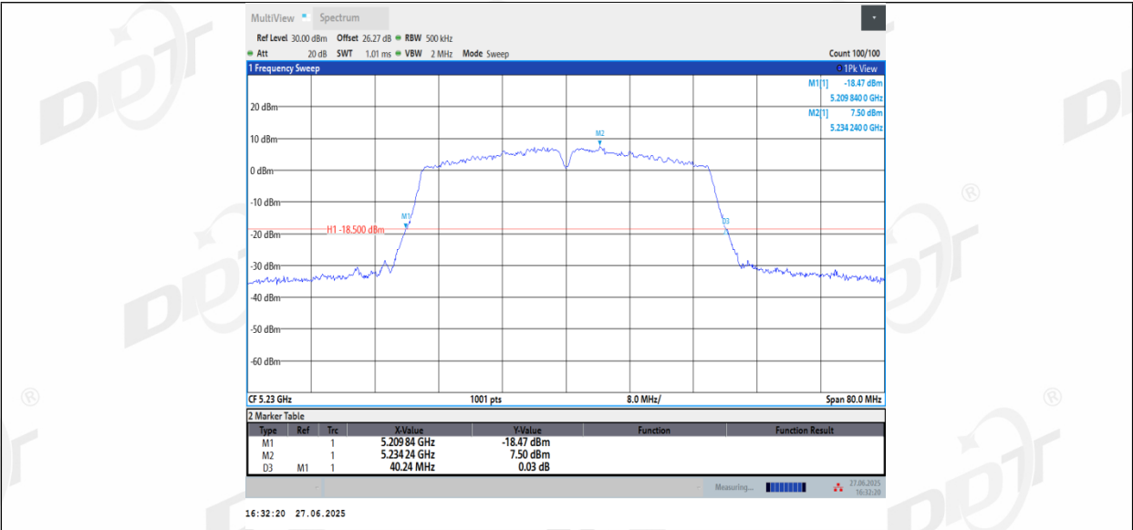
11N40_Ant2_5230
