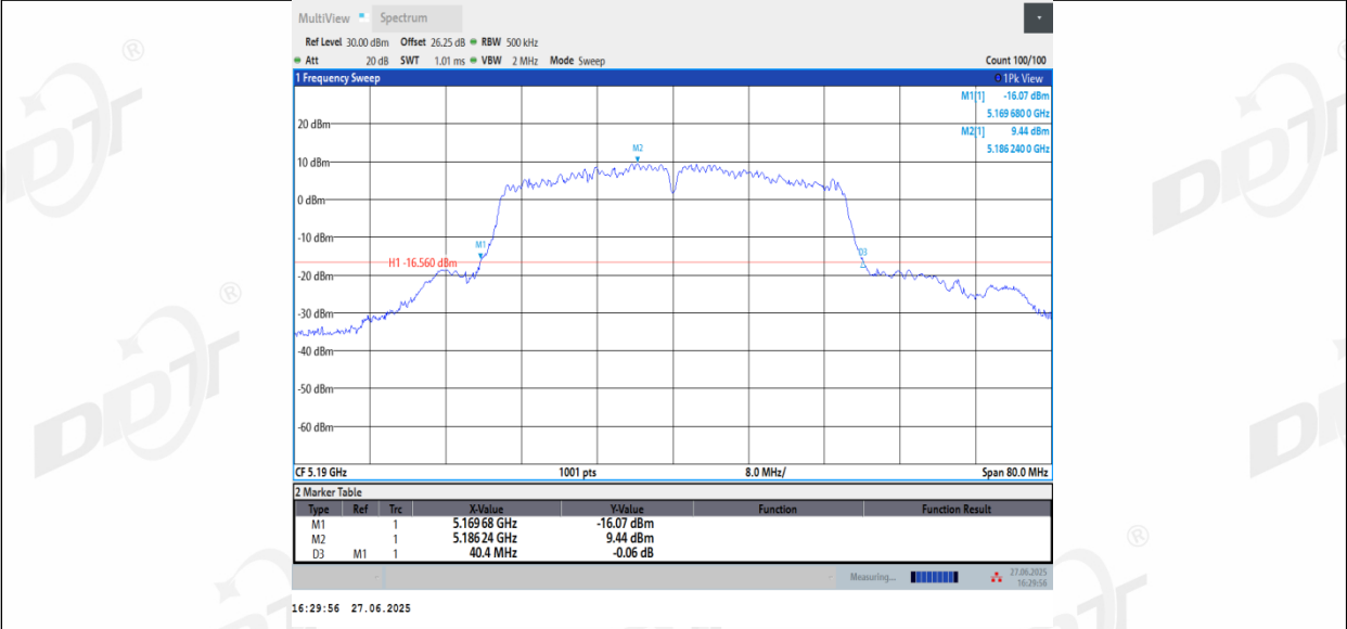
11N40_Ant3_5190
