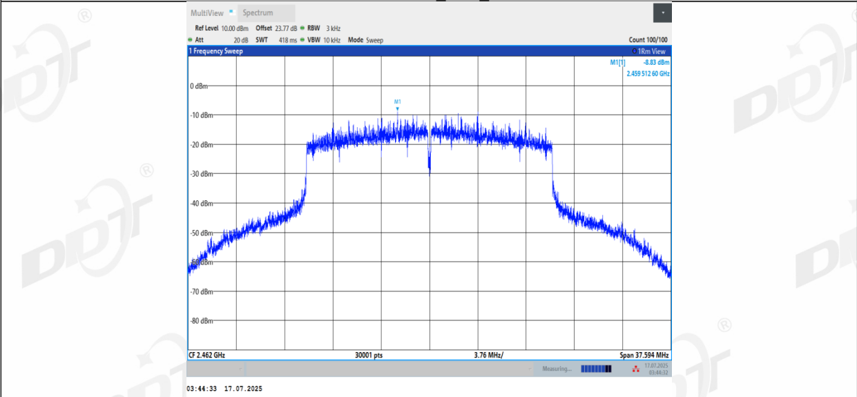
11AX20MIMO_Ant2_2462
