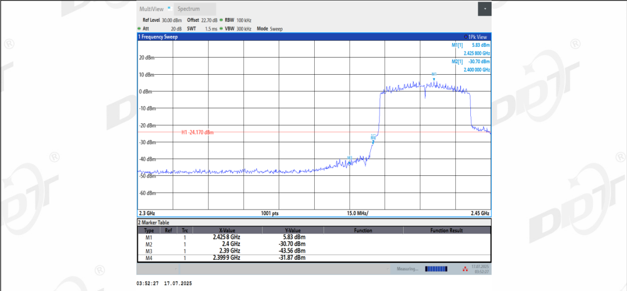
11AX40_Ant2_Low_2422
