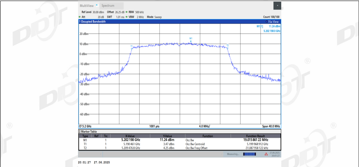
11AX20_Ant2_5200
