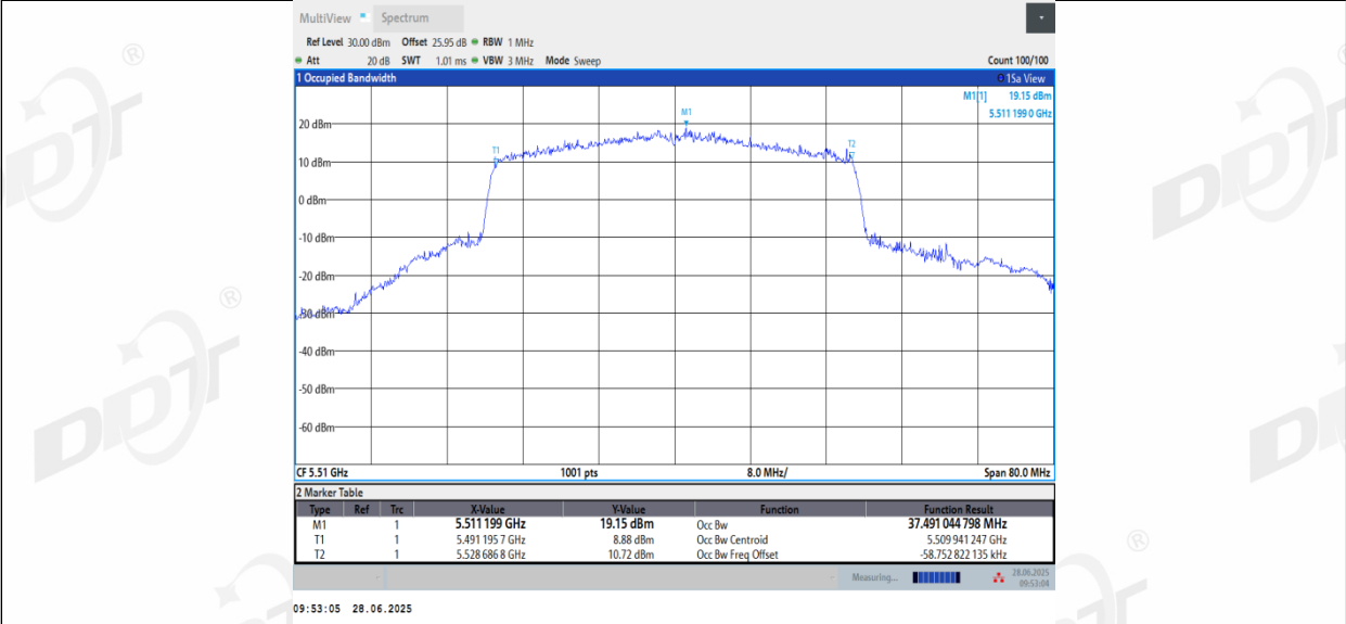
11AX40_Ant3_5510
