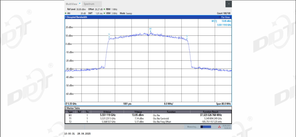
11AX40_Ant3_5550
