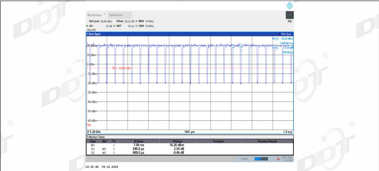
11AX20MIMO_Ant2_5280
