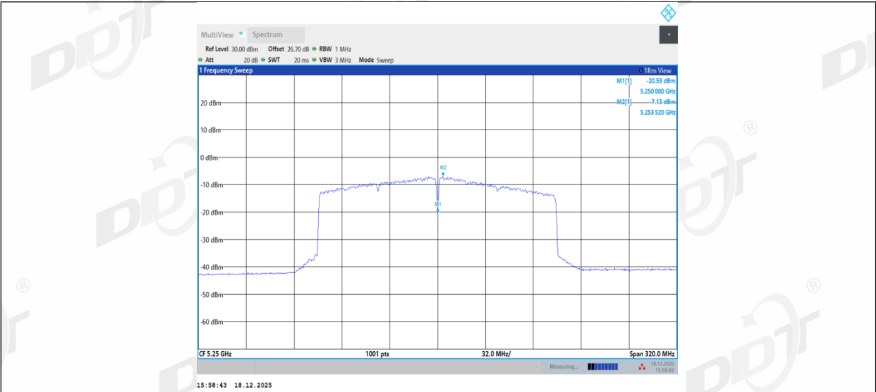
11AX160MIMO_Ant2_5250_UNII-2A
