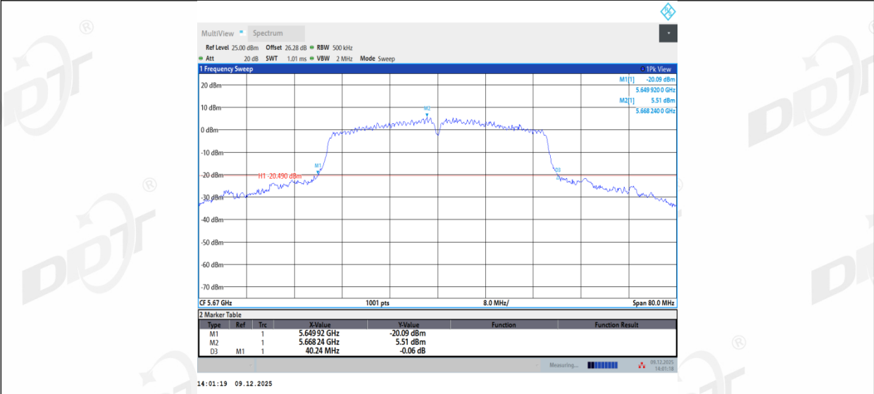
11AC40MIMO_Ant3_5670
