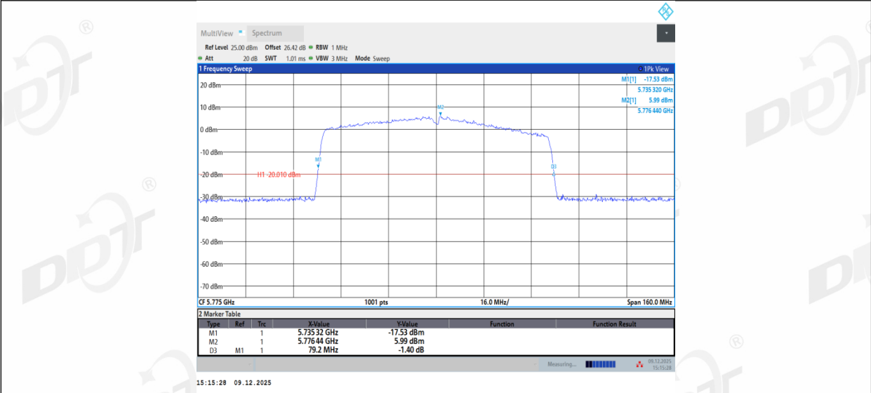
11AC80MIMO_Ant3_5775
