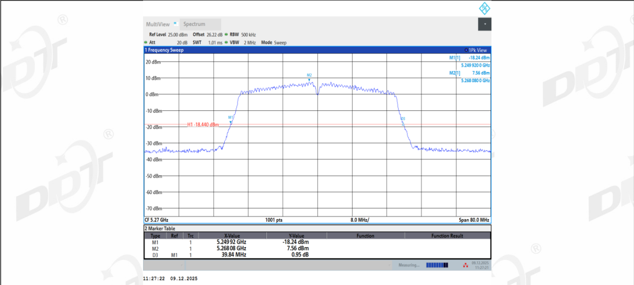
11AC40MIMO_Ant3_5270
