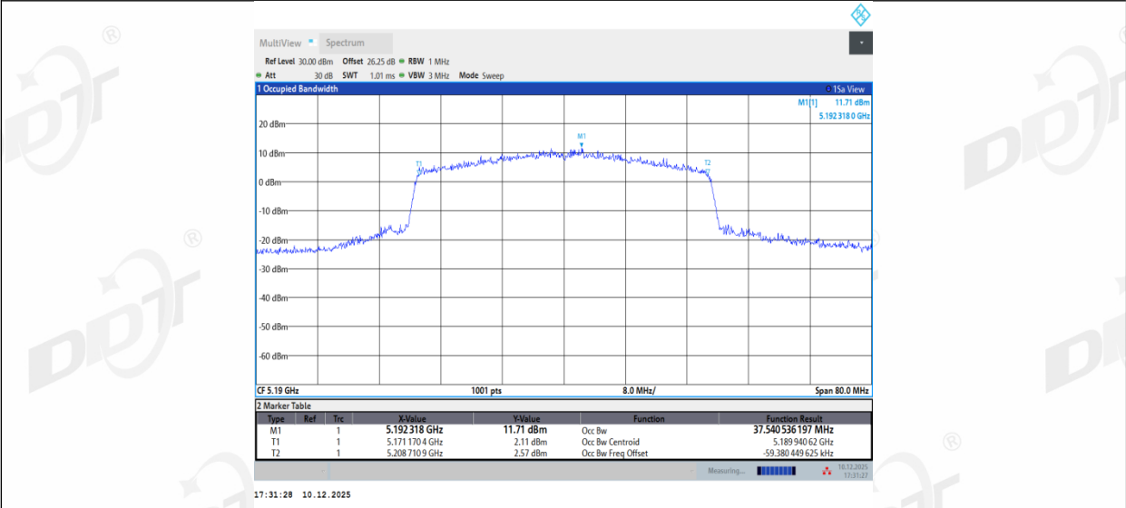
11AX40MIMO_Ant3_5190
