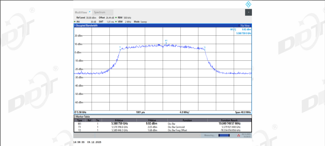
11AX20MIMO_Ant3_5580
