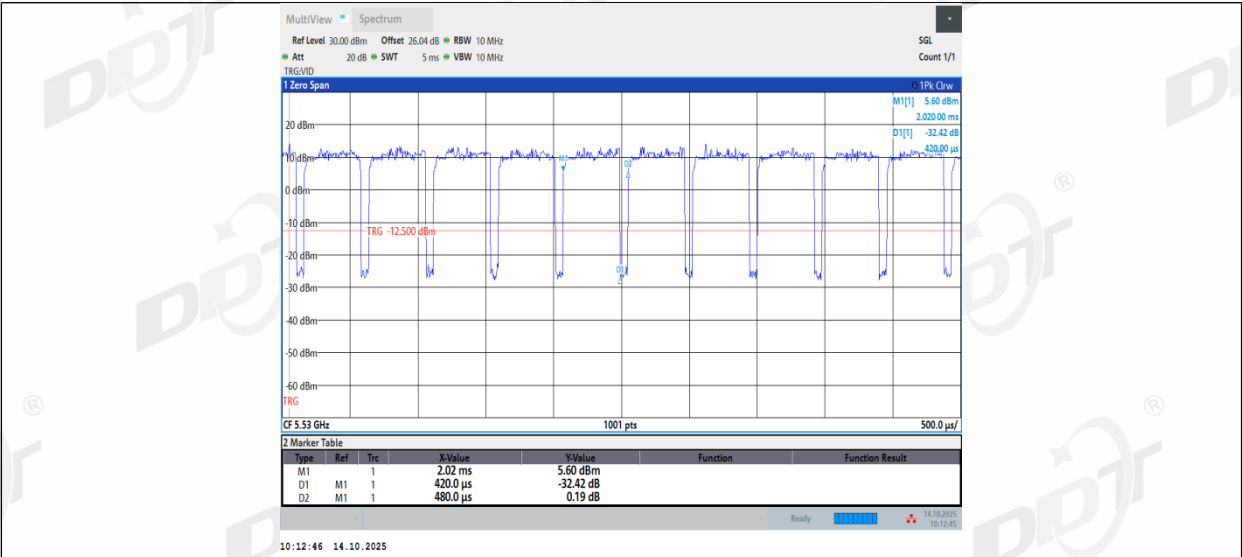
11AX80MIMO_Ant2_5530
