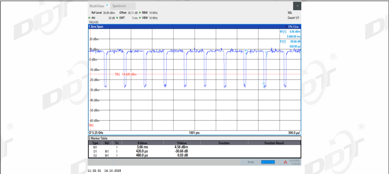
11AX160MIMO_Ant2_5250
