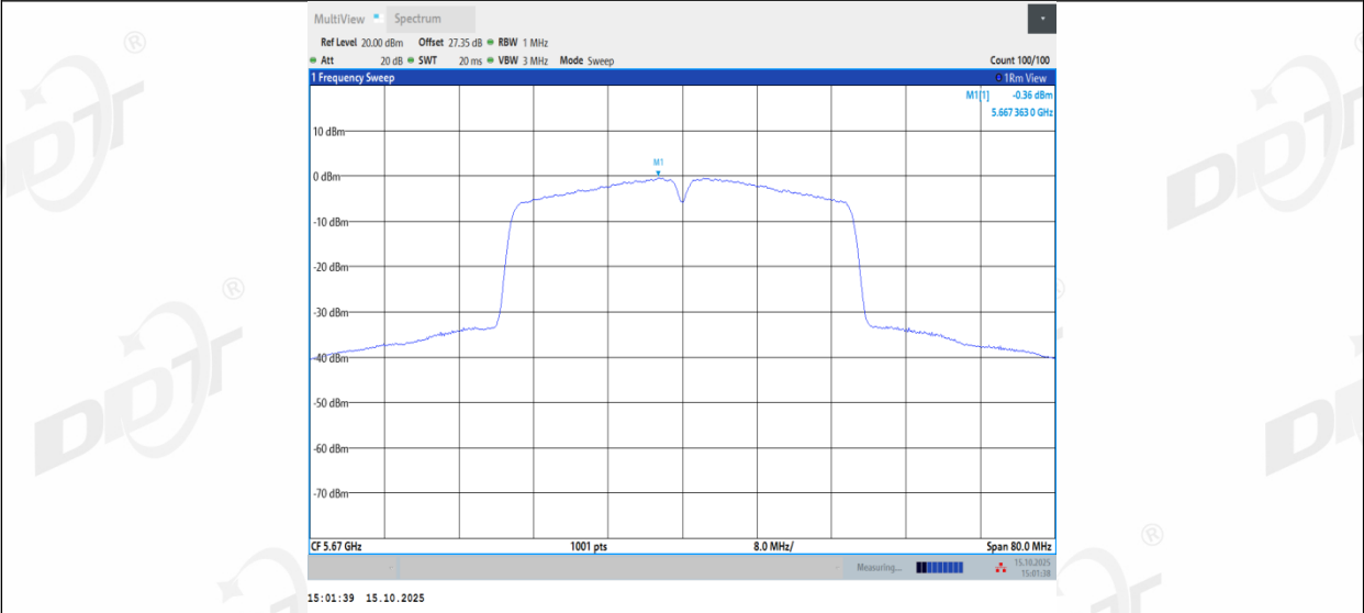
11N40MIMO_Ant3_5670
