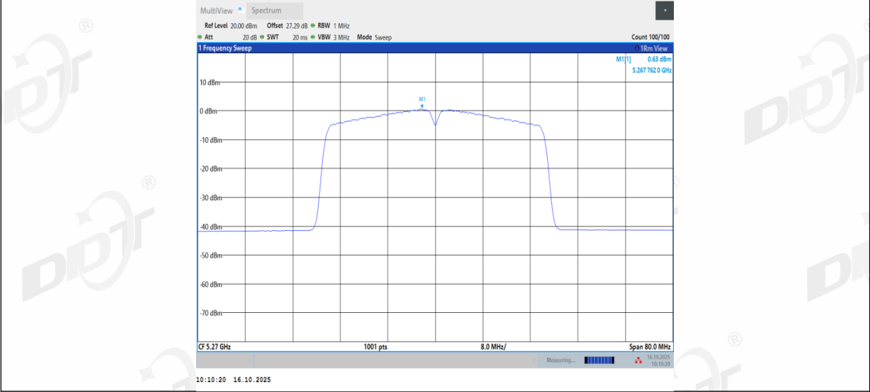
11AC40MIMO_Ant3_5270
