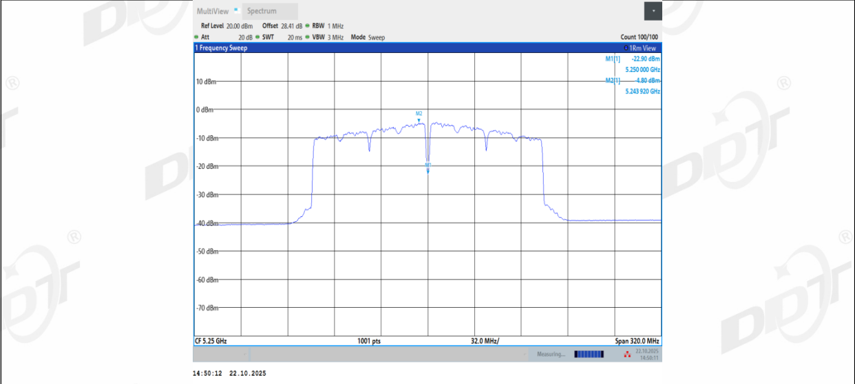
11AC160MIMO_Ant1_5250_UNII-2A
