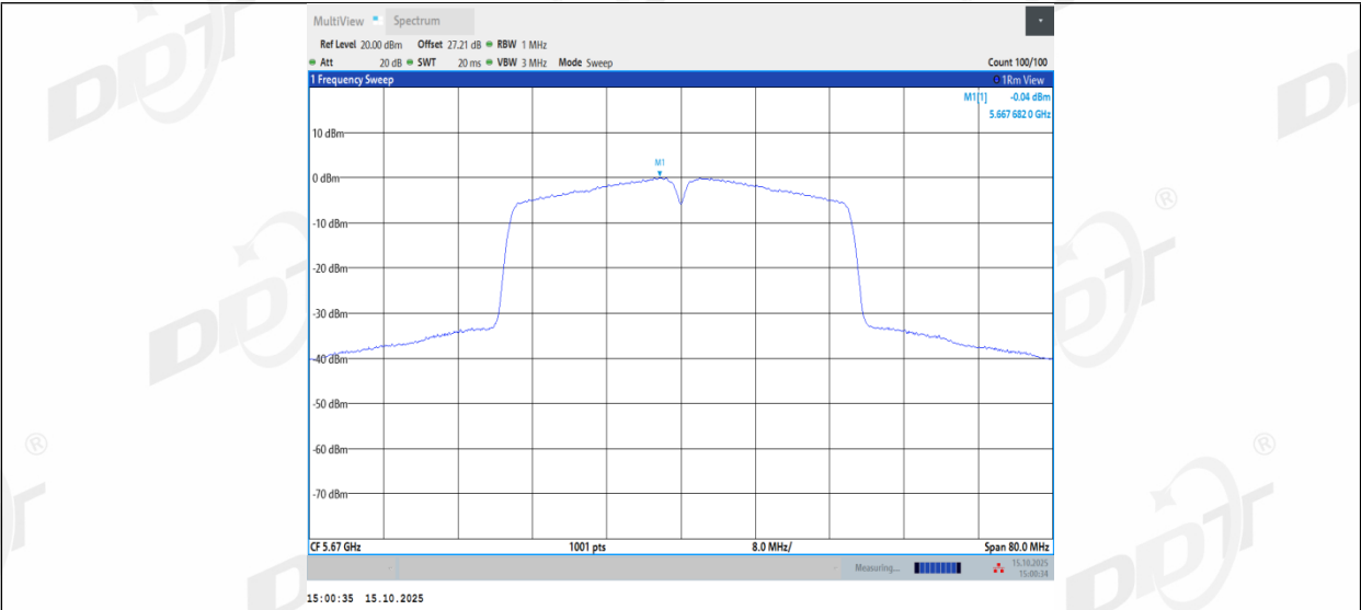
11N40MIMO_Ant2_5670
