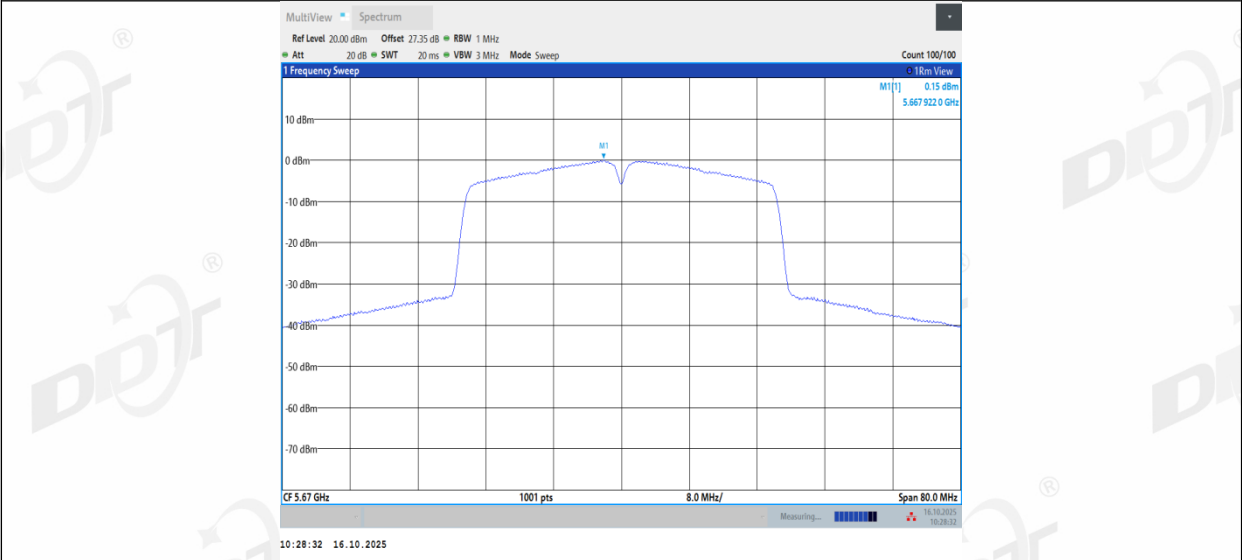
11AC40MIMO_Ant3_5670
