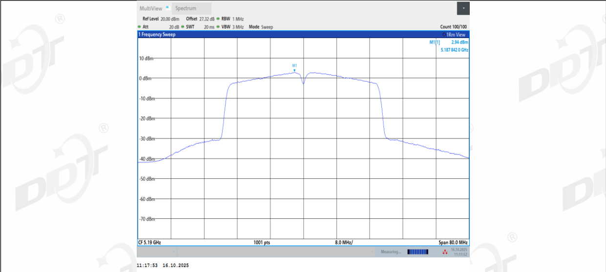
11AC40MIMO_Ant3_5190
