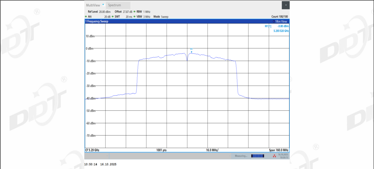
11AC80MIMO_Ant3_5290
