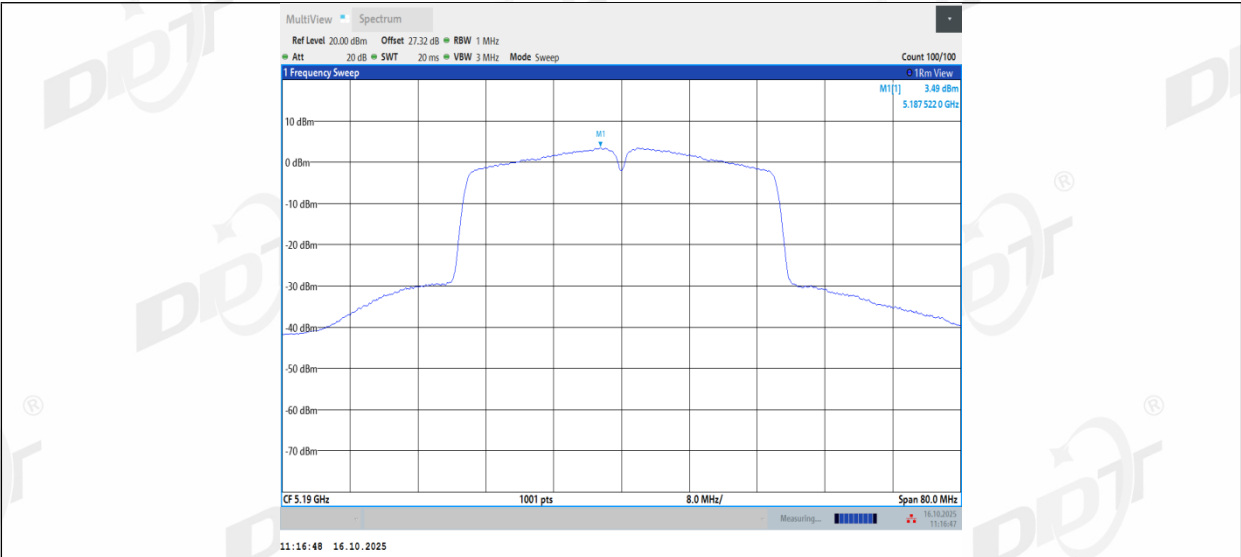
11AC40MIMO_Ant2_5190
