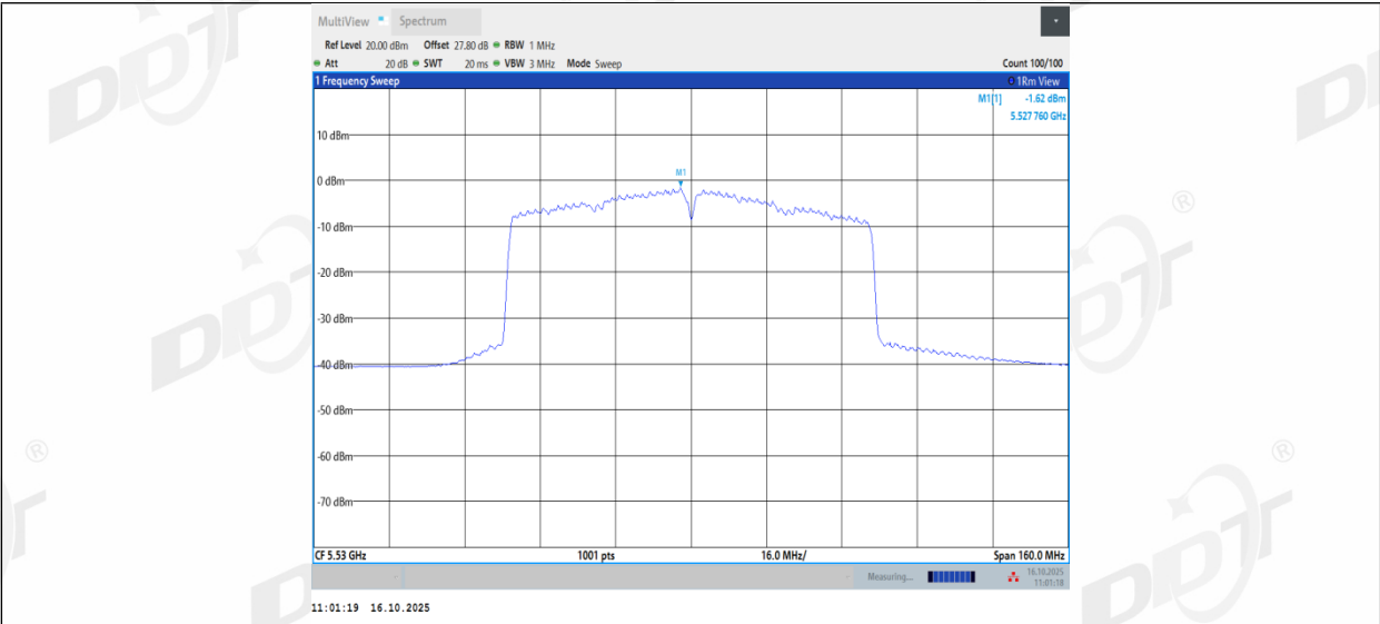
11AC80MIMO_Ant2_5530
