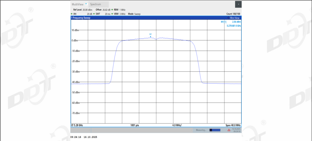
11AC20MIMO_Ant3_5280
