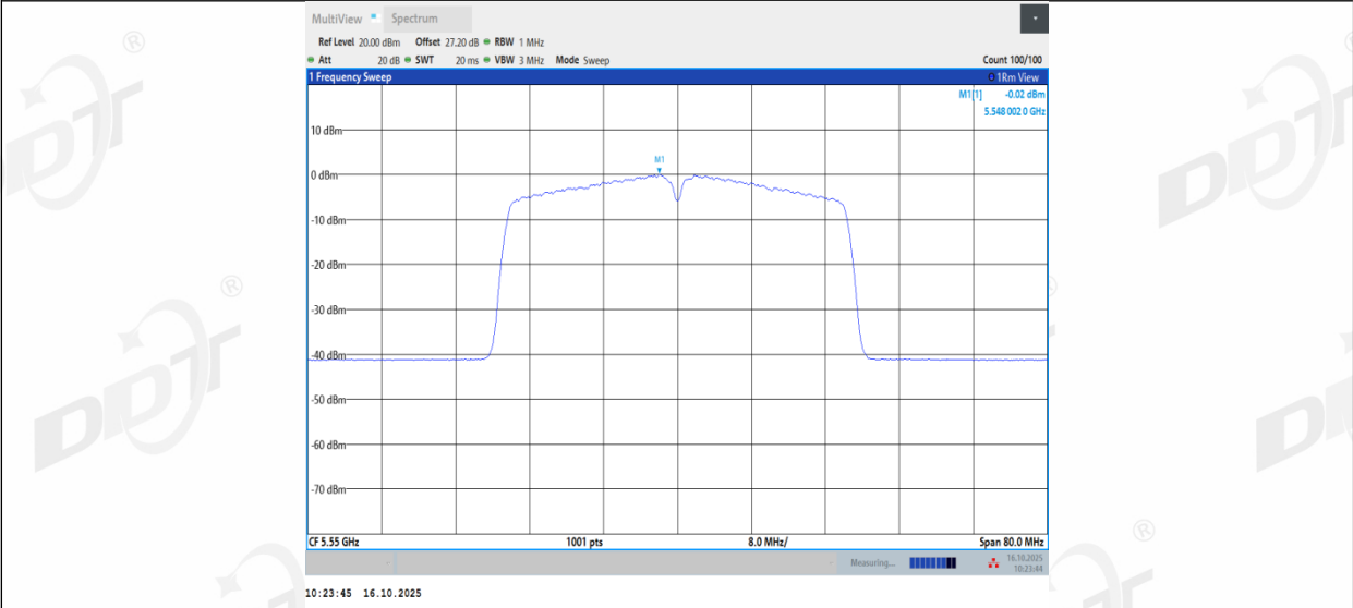
11AC40MIMO_Ant3_5550
