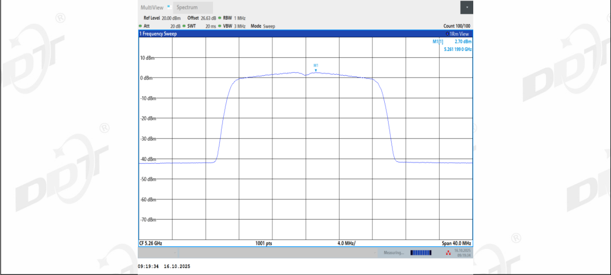
11AC20MIMO_Ant3_5260
