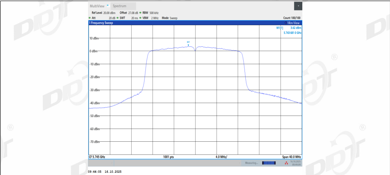
11AC20MIMO_Ant2_5745
