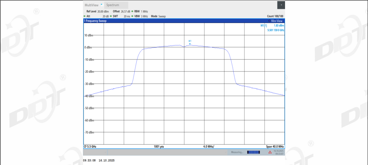
11AC20MIMO_Ant3_5500
