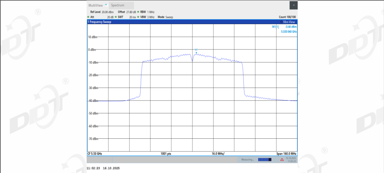
11AC80MIMO_Ant3_5530
