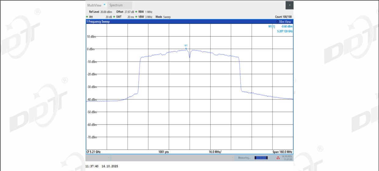
11AC80MIMO_Ant3_5210
