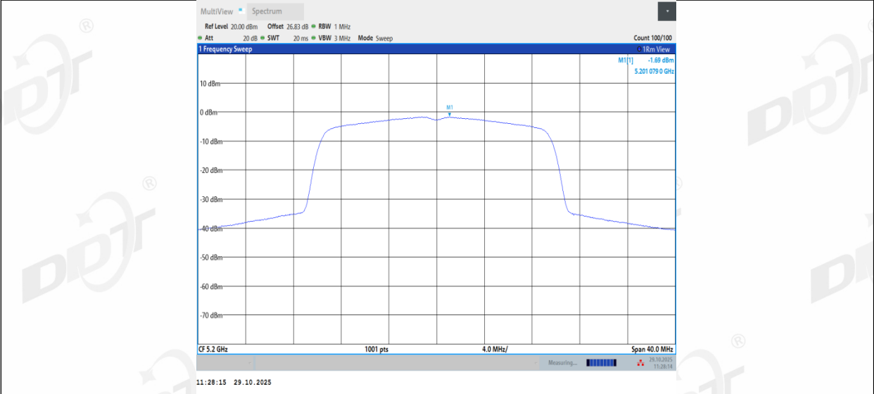
11AX20MIMO_Ant3_5200
