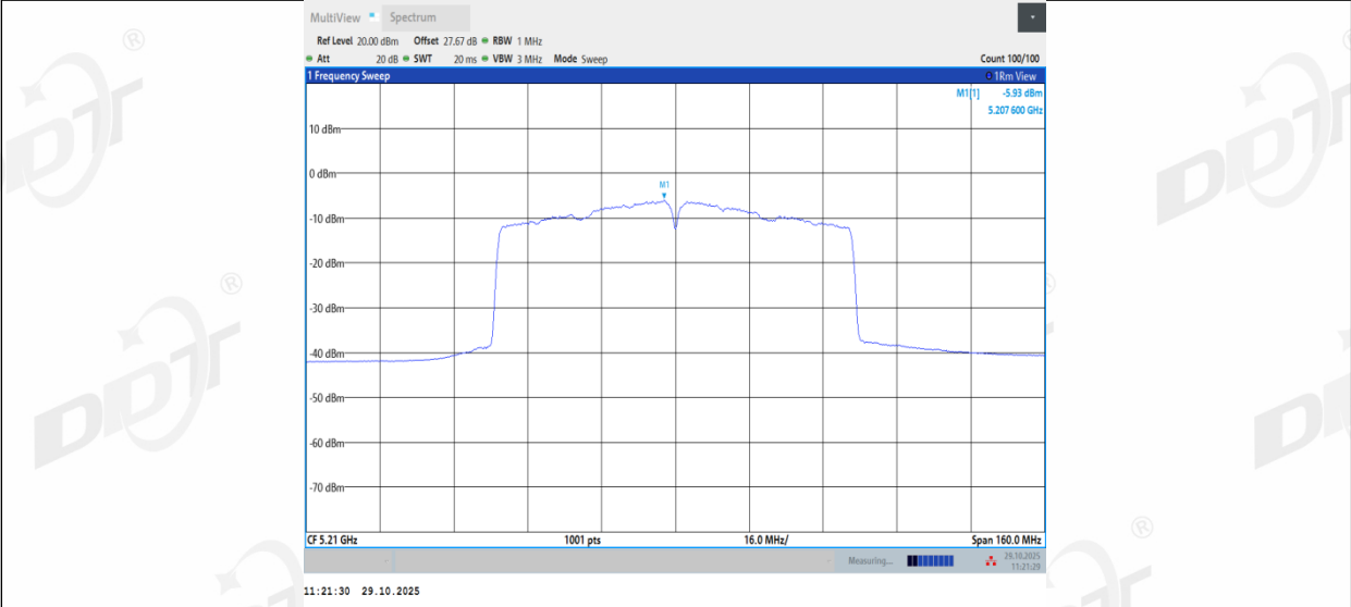
11AC80MIMO_Ant3_5210
