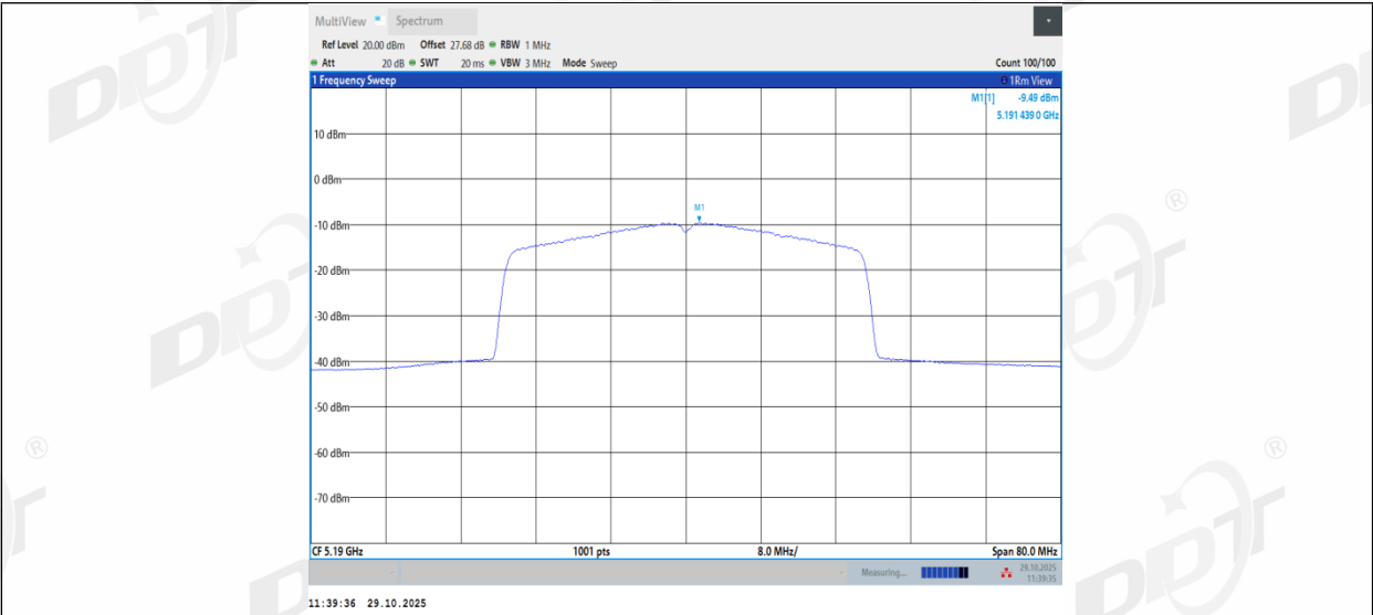
11AX40MIMO_Ant2_5190
