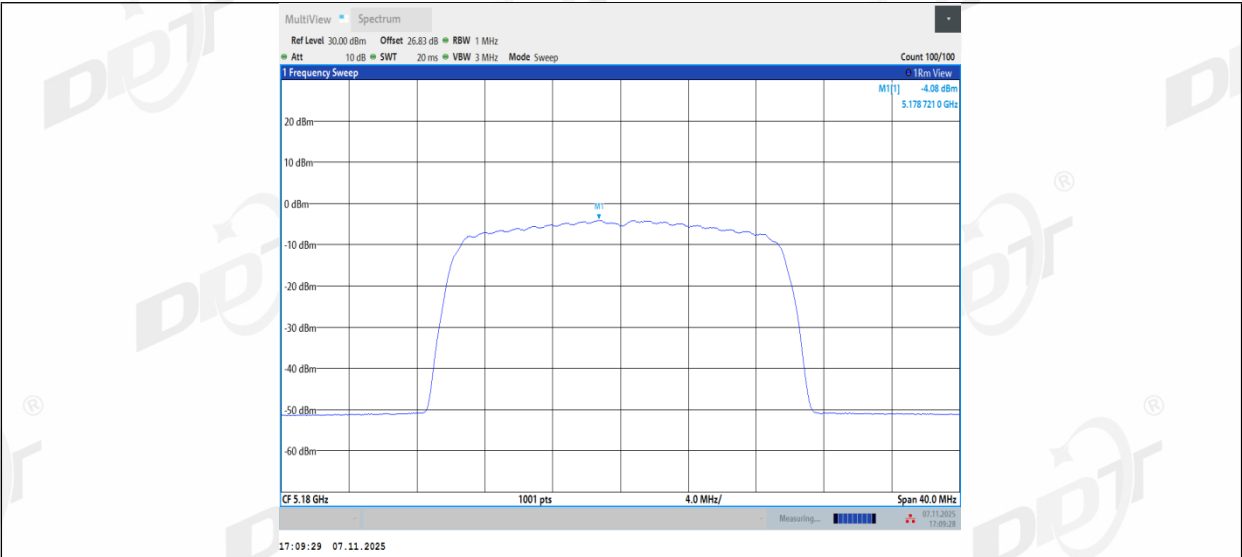
11BE20MIMO_Ant2_5180
