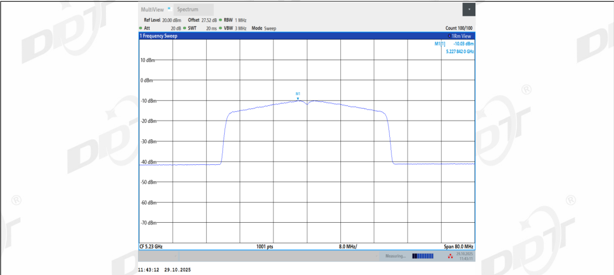
11AX40MIMO_Ant2_5230
