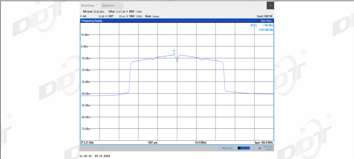
11AC80MIMO_Ant2_5210
