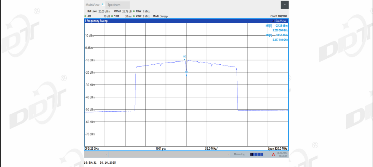
11BE160MIMO_Ant3_5250_UNII-1
