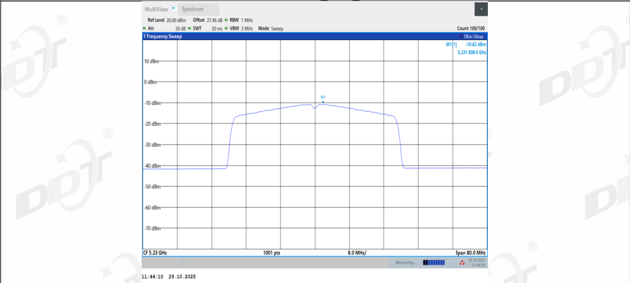
11AX40MIMO_Ant3_5230
