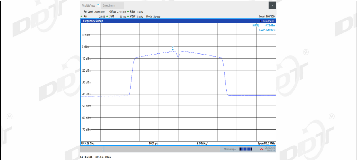
11AC40MIMO_Ant2_5230
