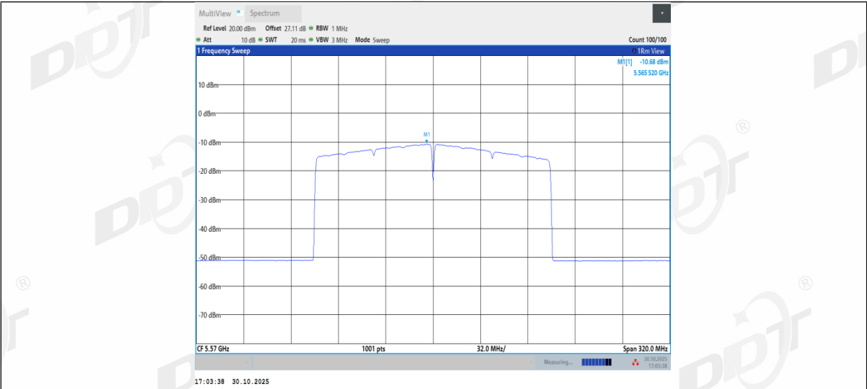
11BE160MIMO_Ant2_5570
