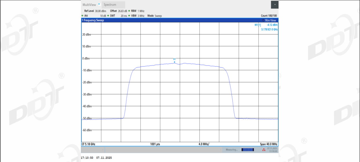
11BE20MIMO_Ant3_5180
