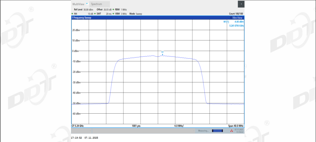
11BE20MIMO_Ant3_5240
