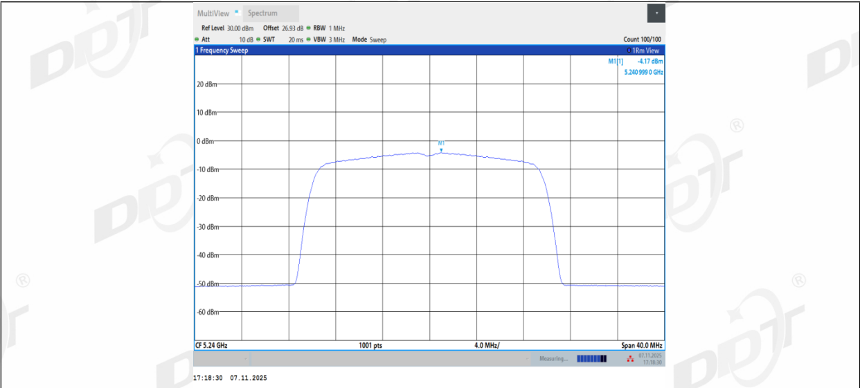
11BE20MIMO_Ant2_5240
