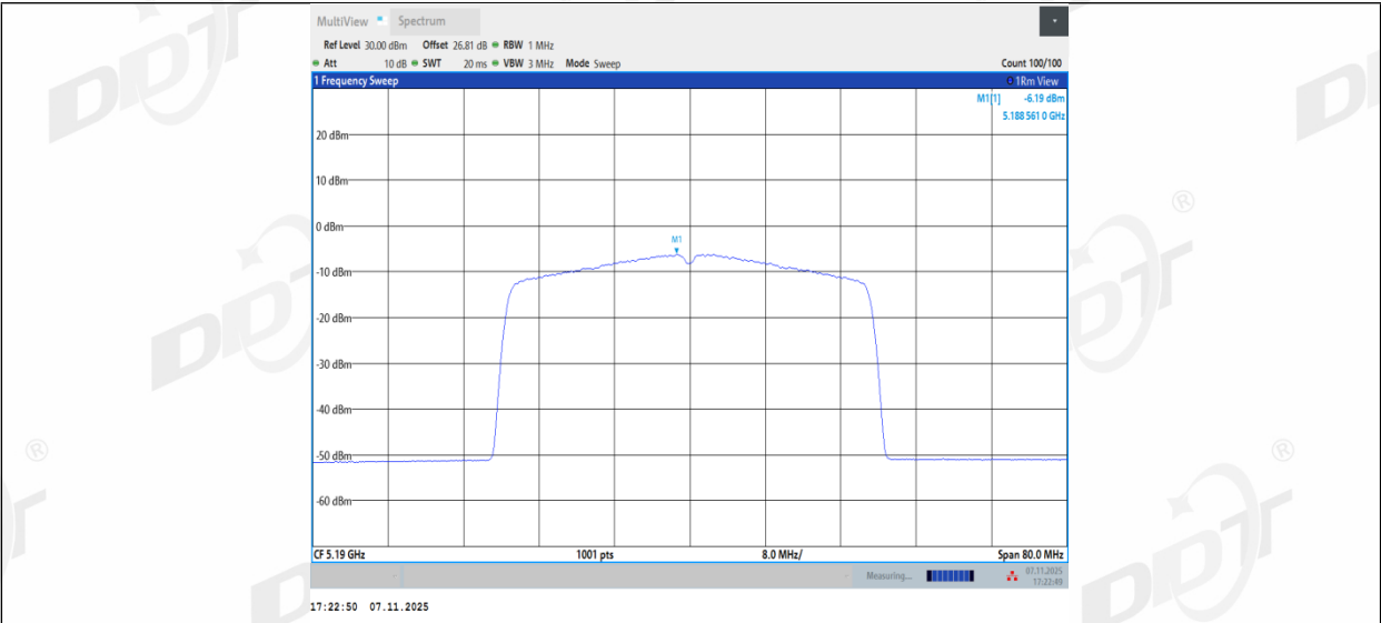
11BE40MIMO_Ant2_5190
