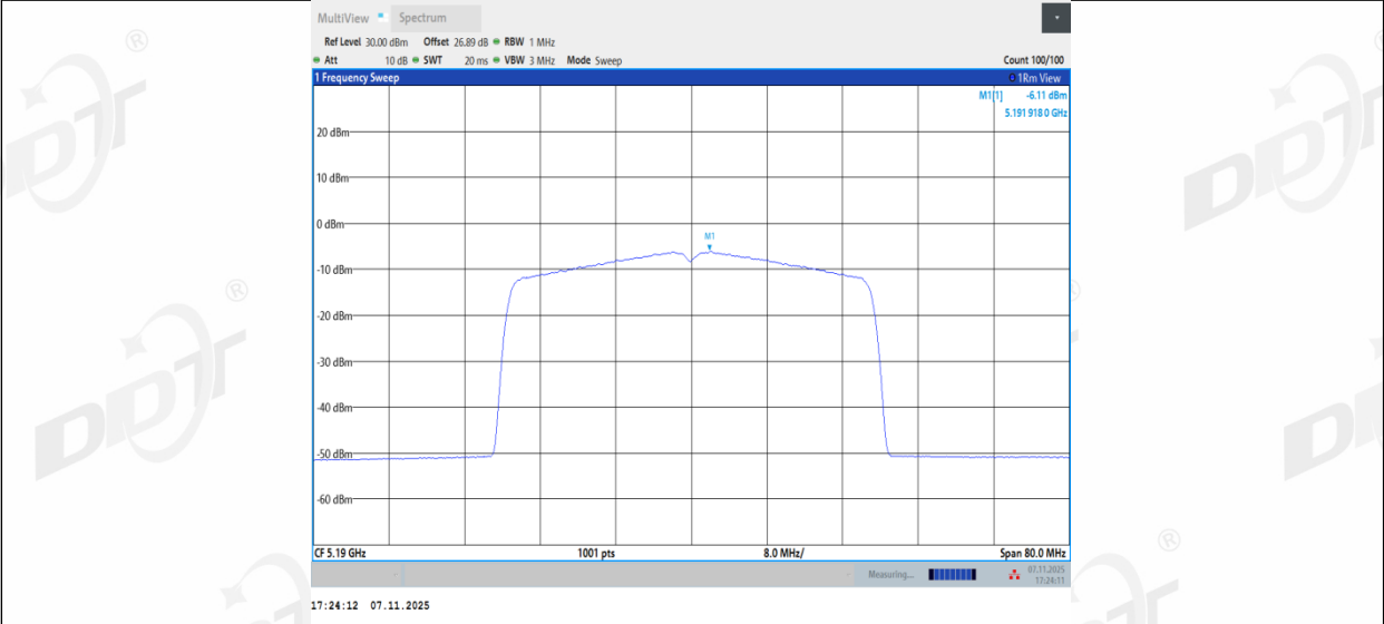
11BE40MIMO_Ant3_5190
