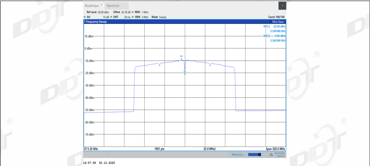
11BE160MIMO_Ant2_5250_UNII-1
