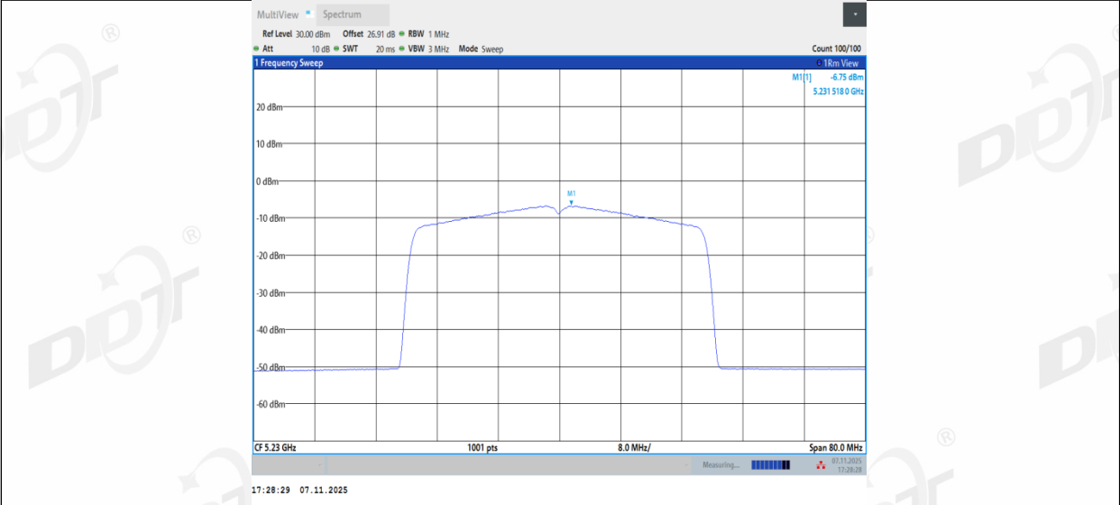
11BE40MIMO_Ant3_5230
