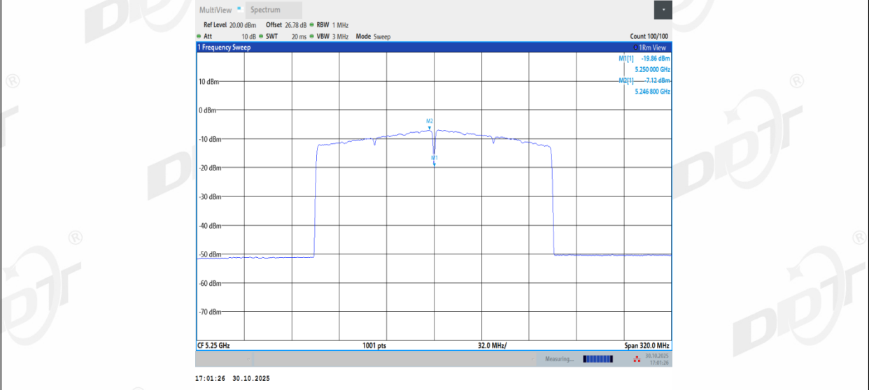
11BE160MIMO_Ant1_5250_UNII-2A
