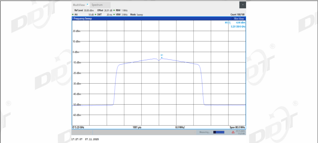
11BE40MIMO_Ant2_5230
