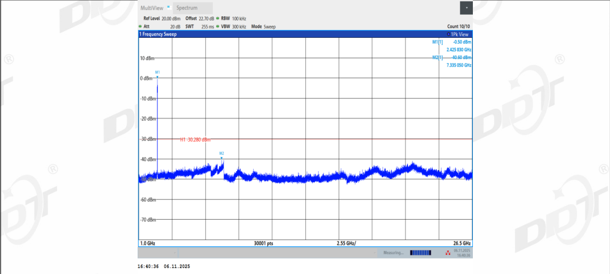
11N40MIMO_Ant2_2422_0~Reference
