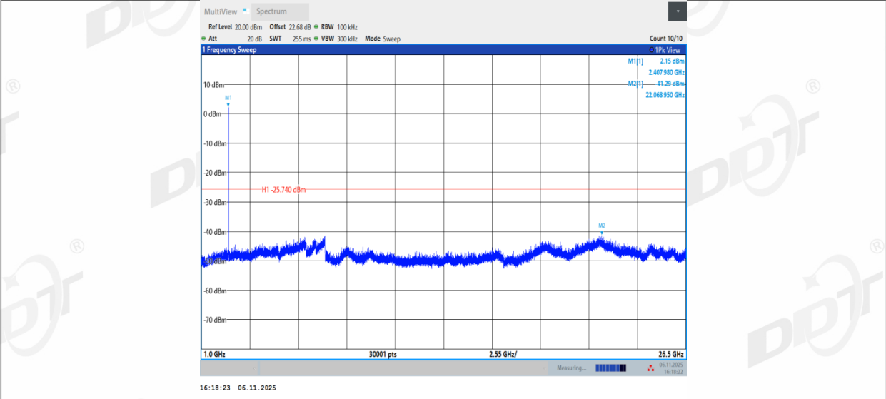
11N20MIMO_Ant2_2412_0~Reference
