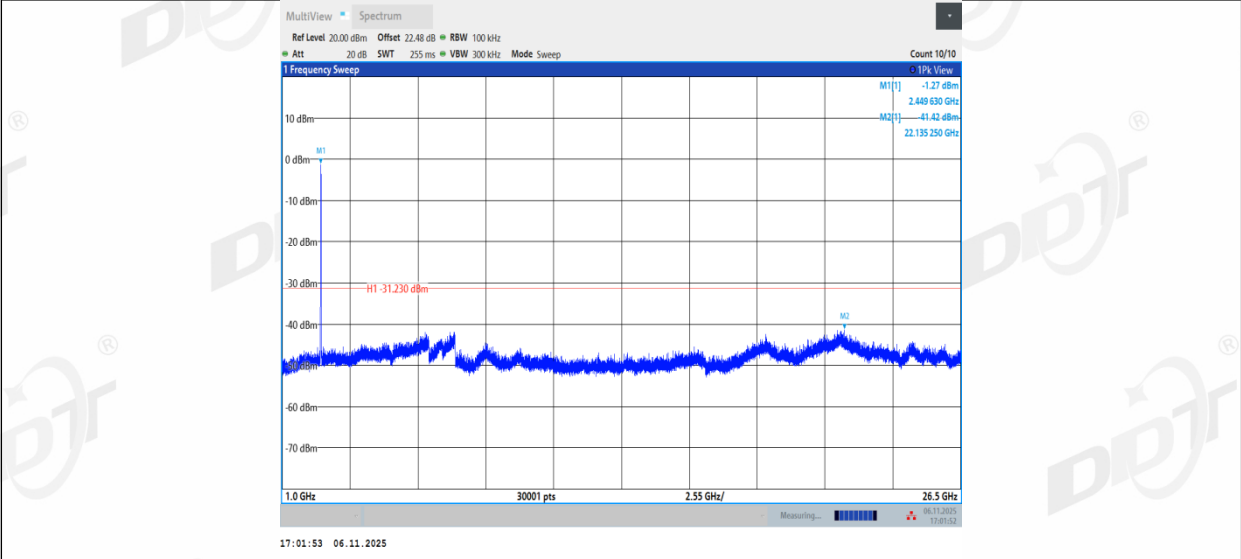
11AX20MIMO_Ant1_2412_0~Reference
