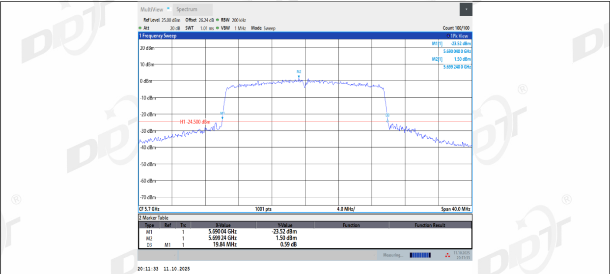
11AX20MIMO_Ant2_5700
