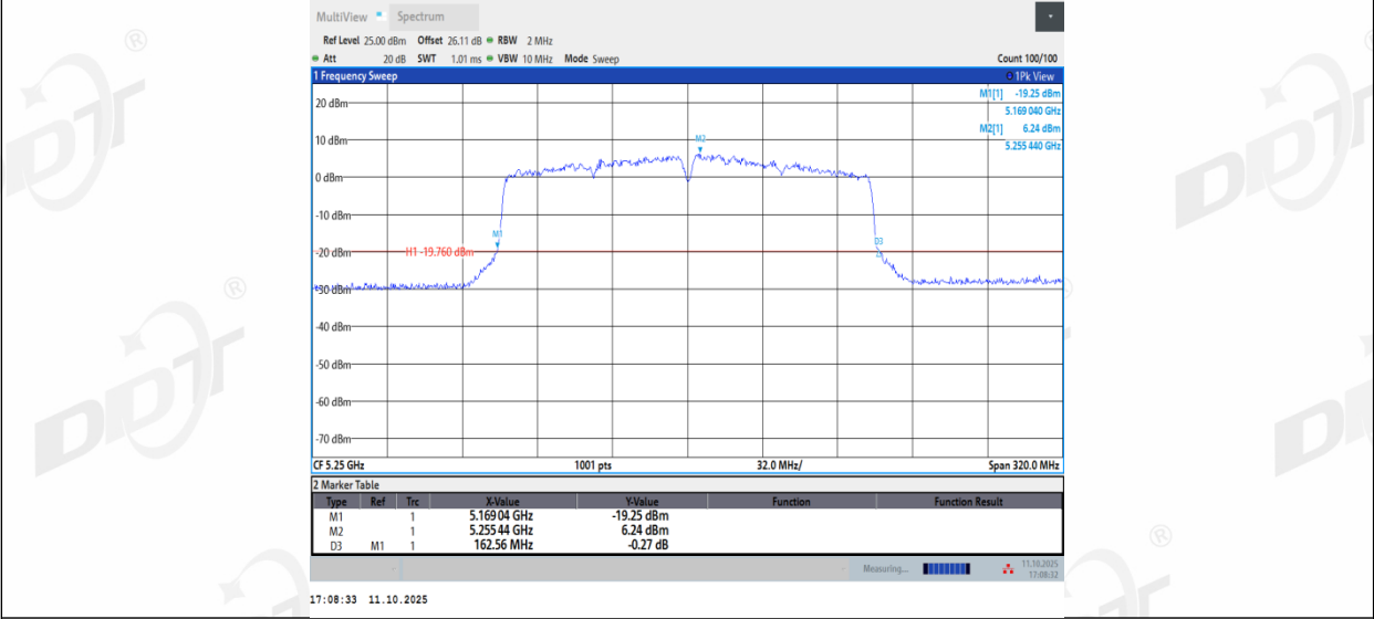
11AC160MIMO_Ant3_5250
