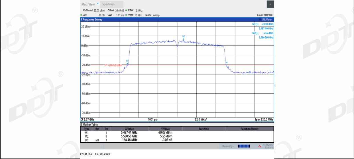
11AC160MIMO_Ant3_5570
