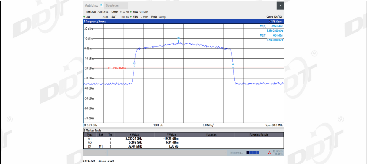
11AX40MIMO_Ant2_5270
