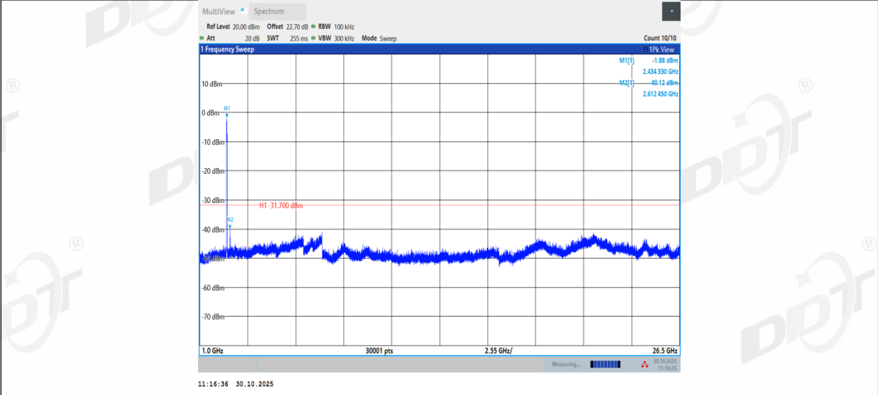
11BE40MIMO_Ant2_2437_0~Reference
