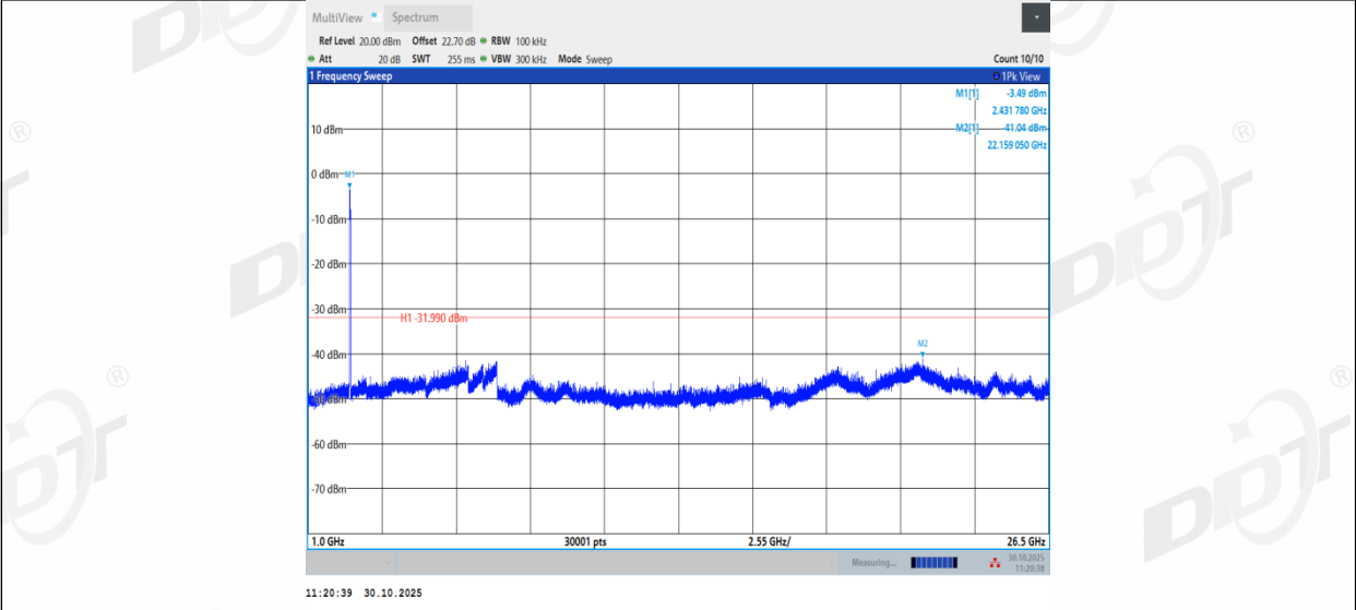
11BE40MIMO_Ant1_2452_0~Reference
