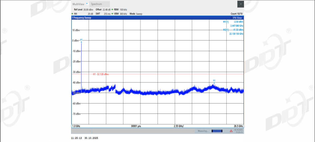
11BE40MIMO_Ant2_2452_0~Reference
