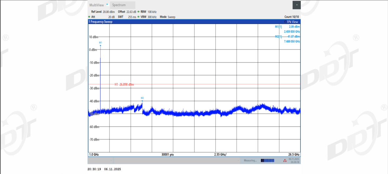
11AX20MIMO_Ant2_2462_0~Reference
