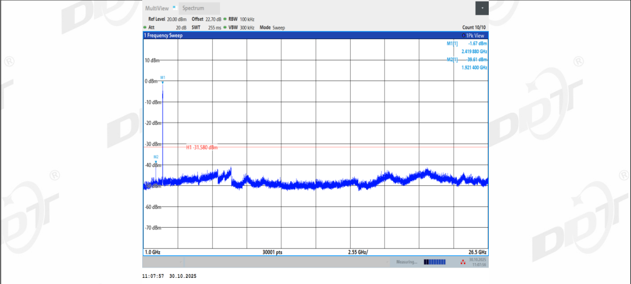
11BE40MIMO_Ant2_2422_0~Reference
