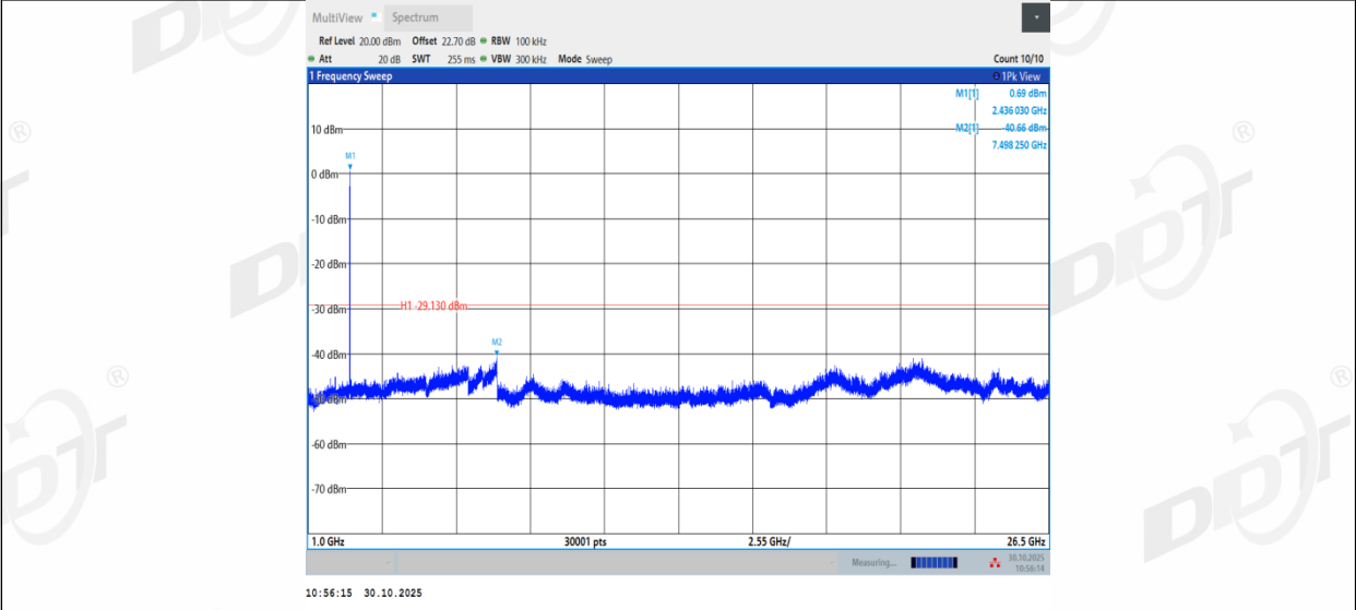
11BE20MIMO_Ant1_2462_0~Reference
