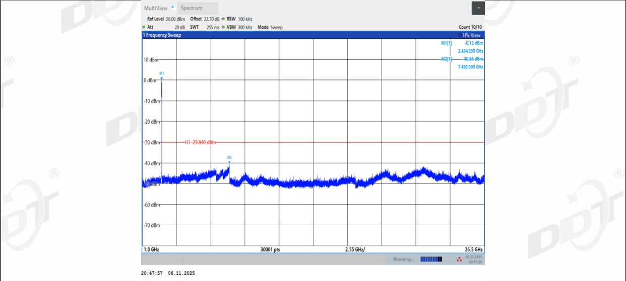
11AX40MIMO_Ant2_2437_0~Reference
