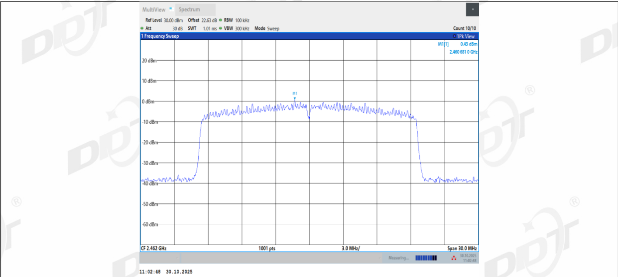
11BE20MIMO_Ant2_2462_30-1000
