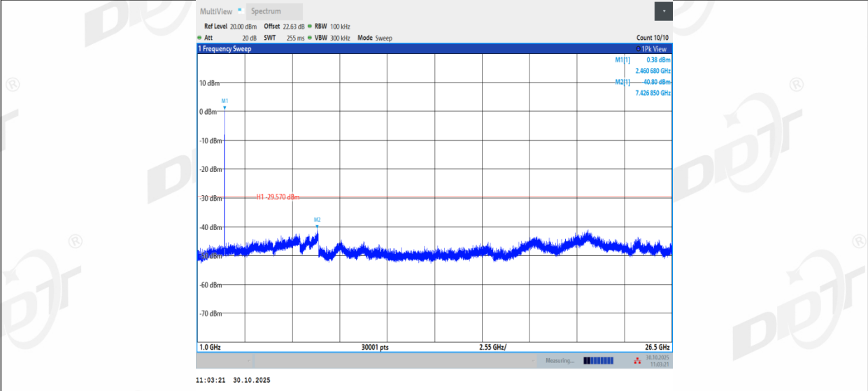
11BE40MIMO_Ant1_2422_0-Reference
