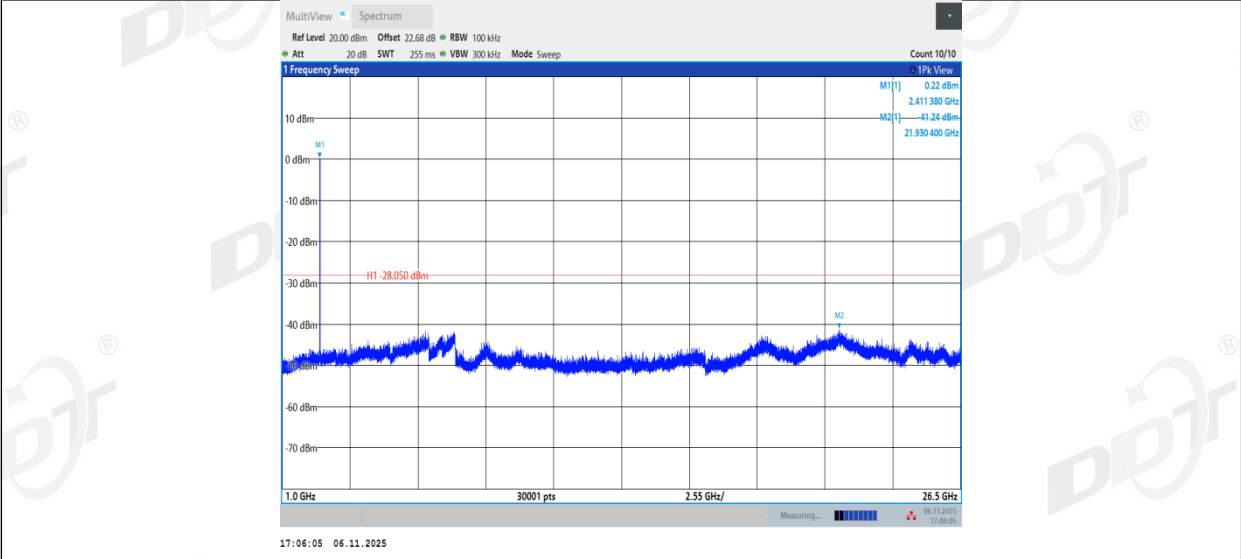
11AX20MIMO_Ant2_2412_0-Reference
