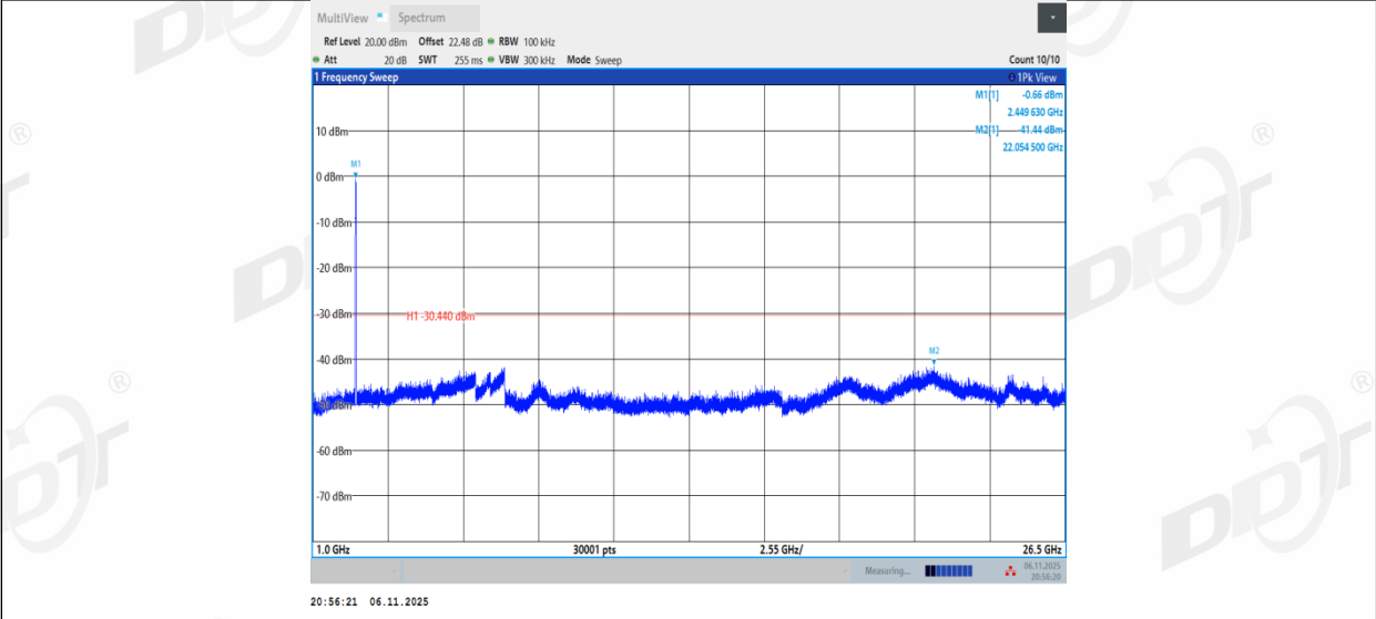
11AX40MIMO_Ant2_2452_0~Reference
