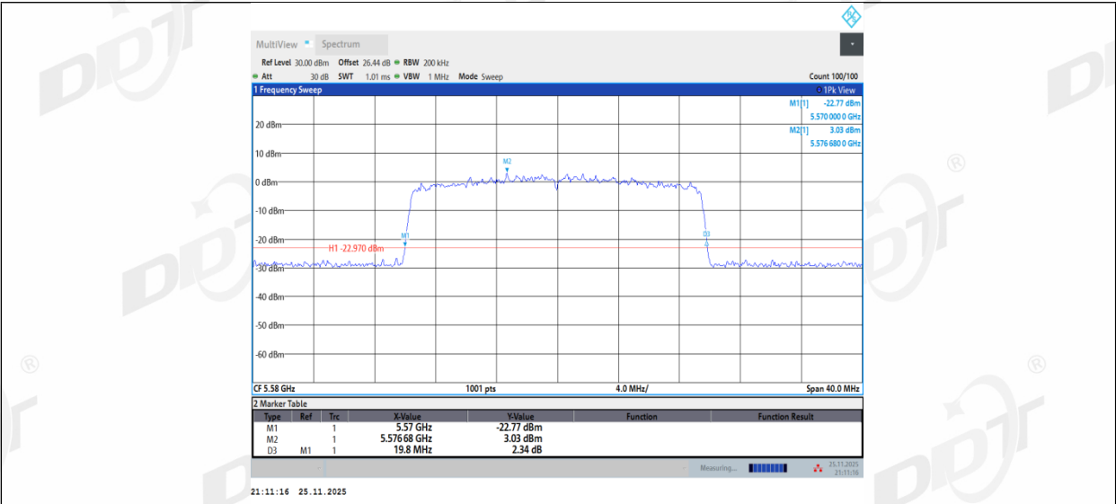
11BE20MIMO_Ant2_5580
