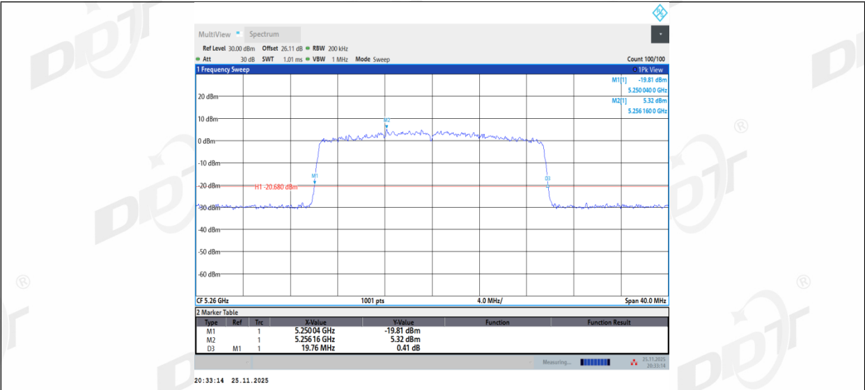
11BE20MIMO_Ant2_5260
