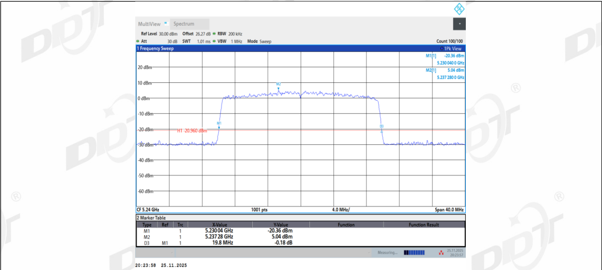
11BE20MIMO_Ant2_5240
