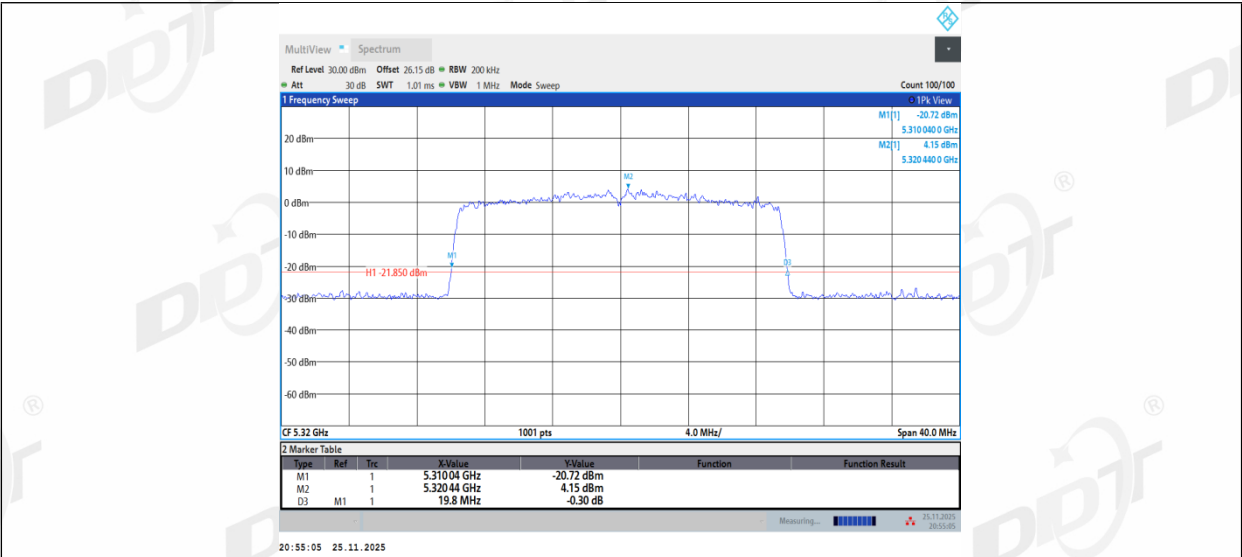
11BE20MIMO_Ant2_5320
