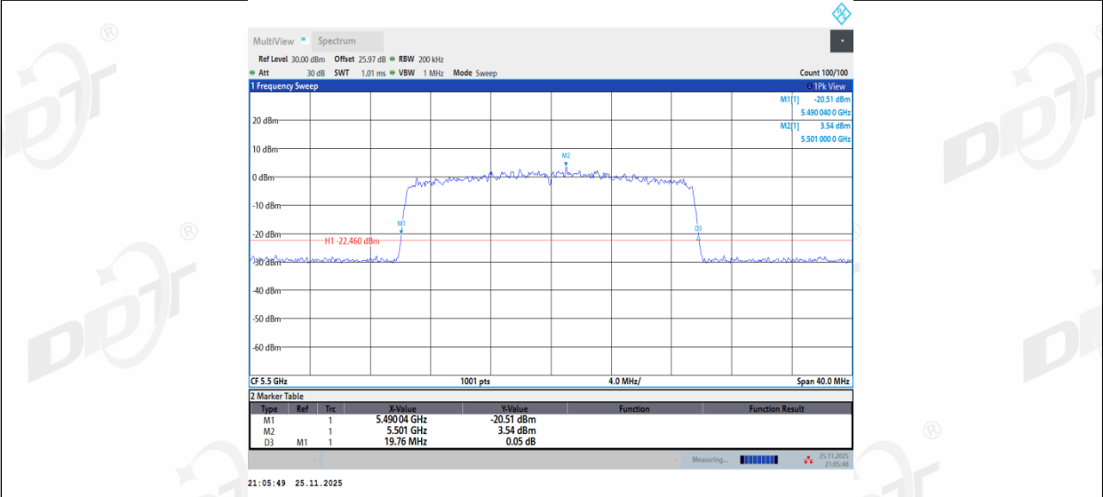
11BE20MIMO_Ant3_5500
