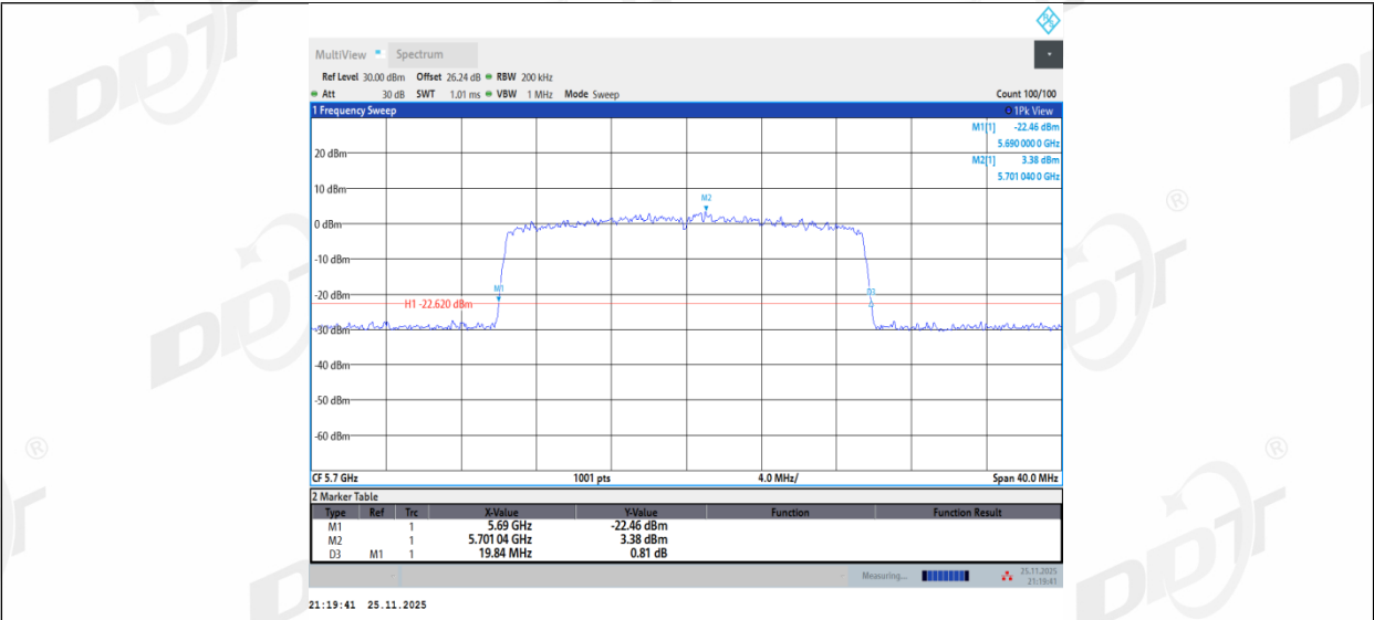
11BE20MIMO_Ant2_5700
