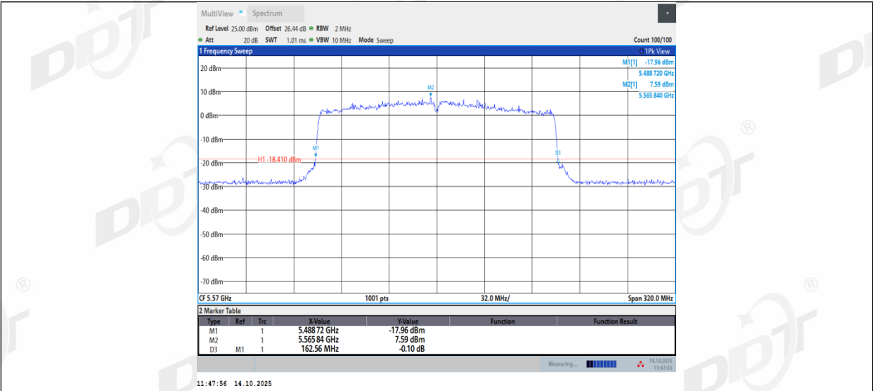
11AX160MIMO_Ant2_5570
