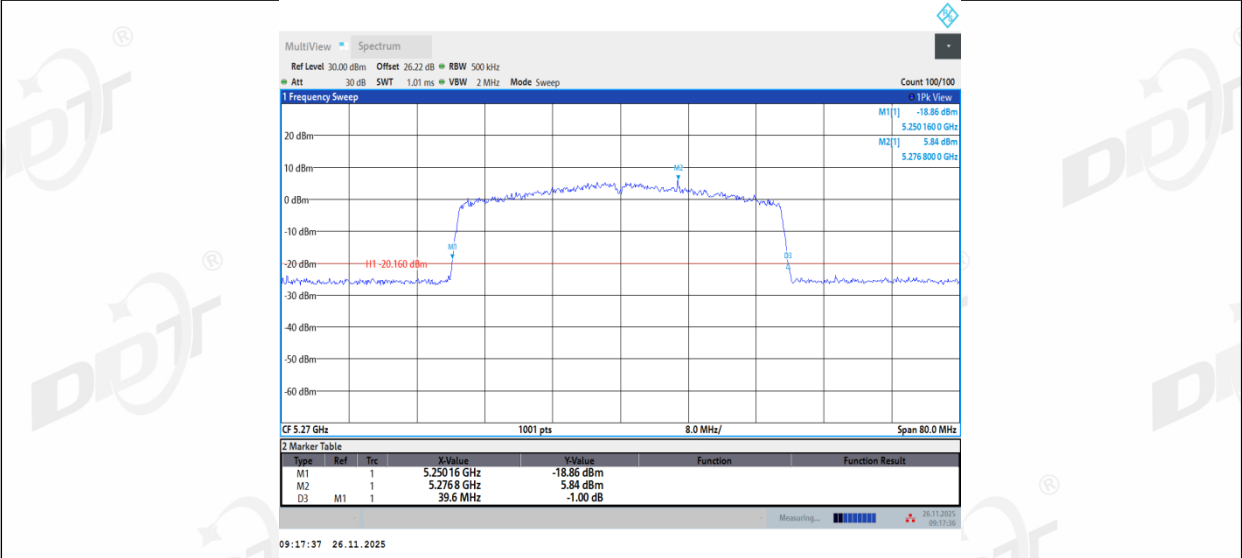
11BE40MIMO_Ant3_5270
