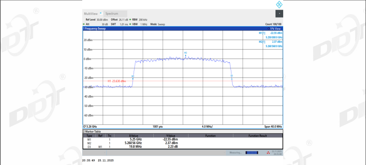
11BE20MIMO_Ant3_5260
