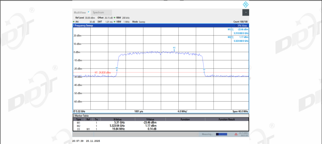
11BE20MIMO_Ant3_5320
