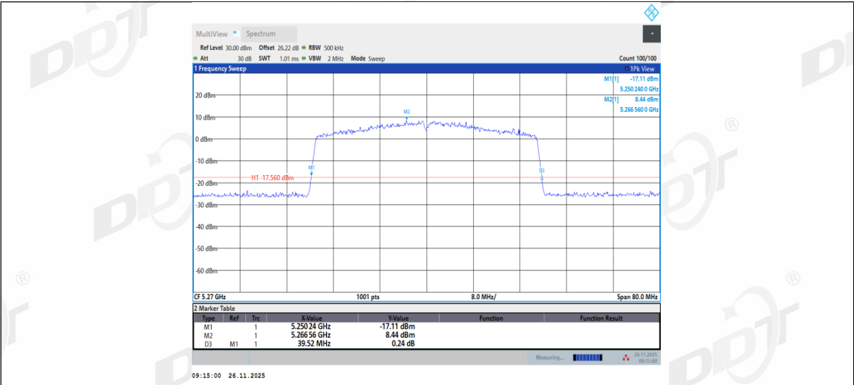
11BE40MIMO_Ant2_5270
