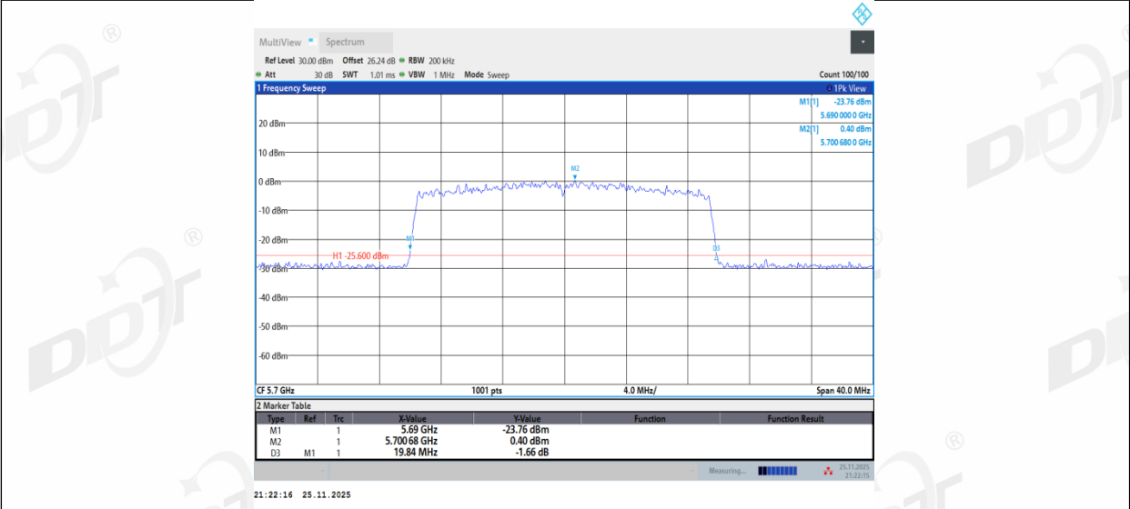
11BE20MIMO_Ant3_5700
