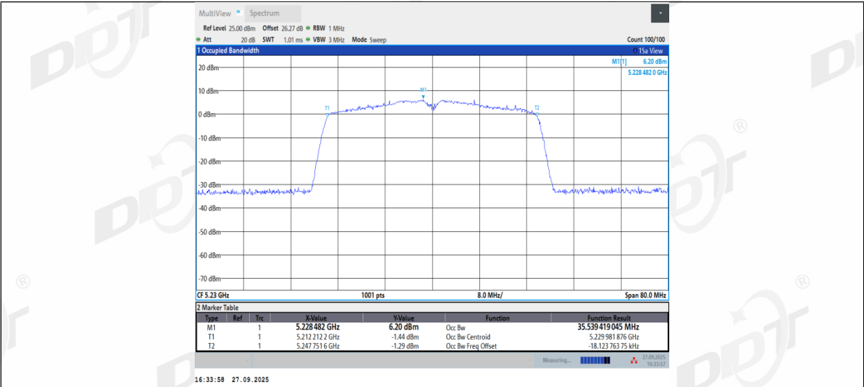
11N40MIMO_Ant2_5230
