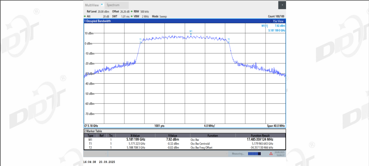
11N20MIMO_Ant3_5180
