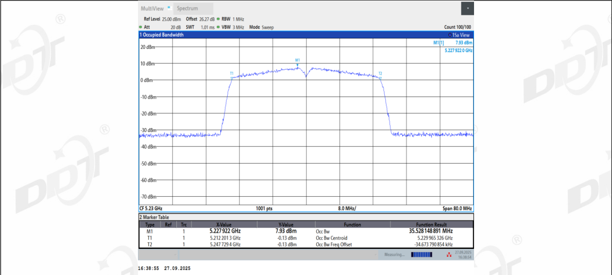
11N40MIMO_Ant3_5230
