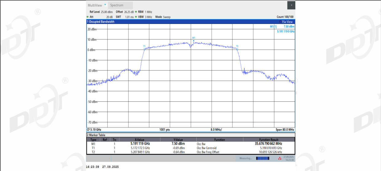
11N40MIMO_Ant3_5190
