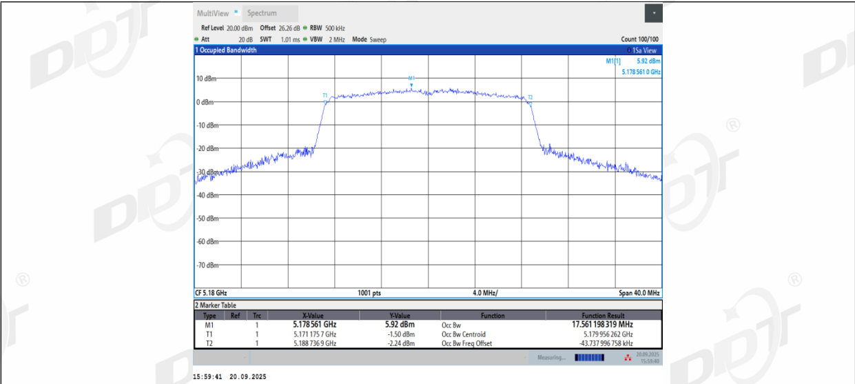
11N20MIMO_Ant2_5180
