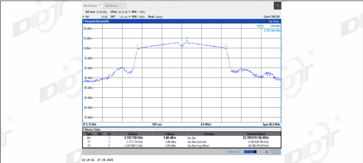
11N40MIMO_Ant2_5190
