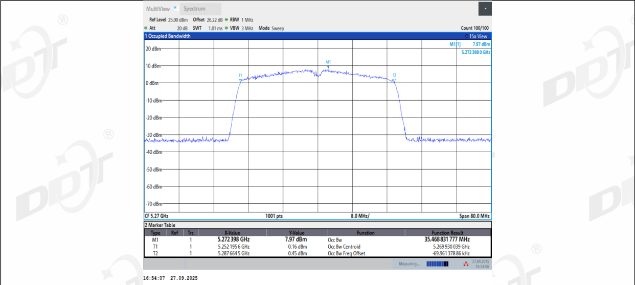
11N40MIMO_Ant3_5270
