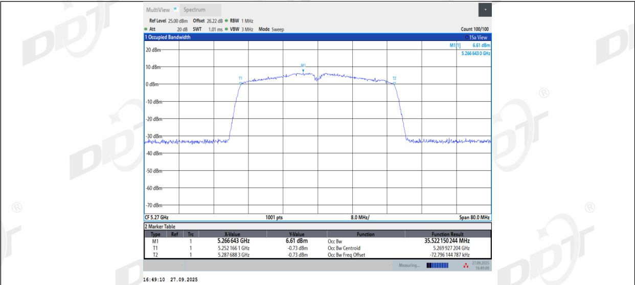
11N40MIMO_Ant2_5270
