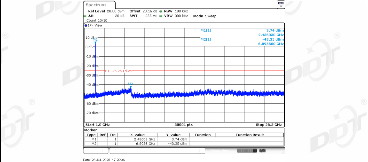
11BE20MIMO_Ant2_2437_0~Reference
