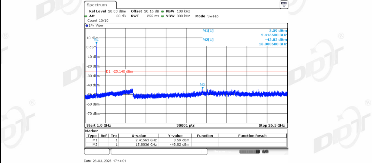
11BE20MIMO_Ant2_2412_0~Reference
