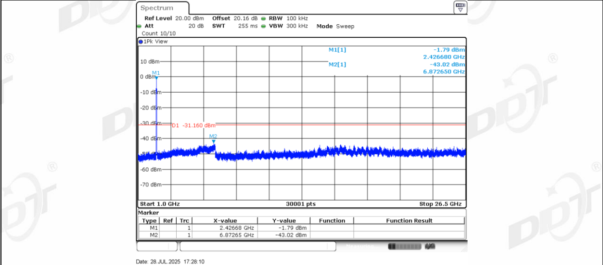
11BE40MIMO_Ant2_2422_0~Reference
