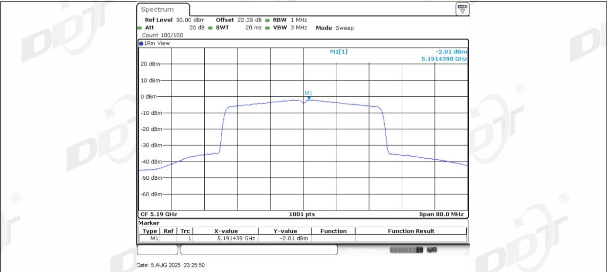
11BE40MIMO_Ant2_5190
