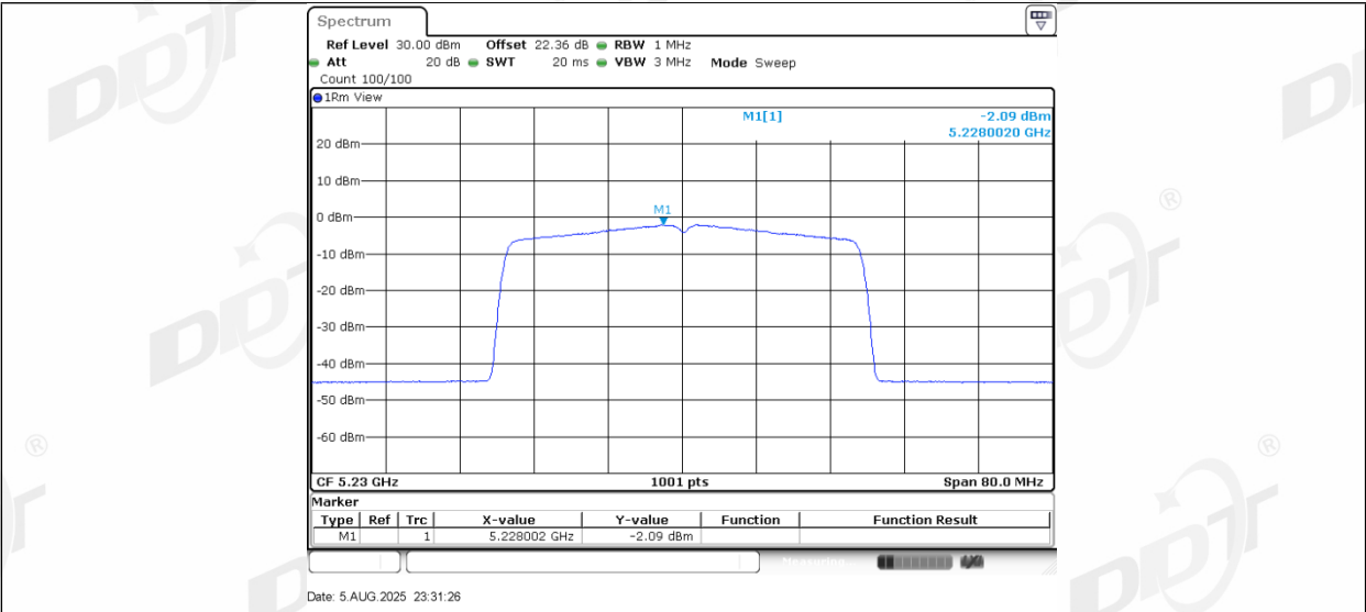
11BE40MIMO_Ant2_5230
