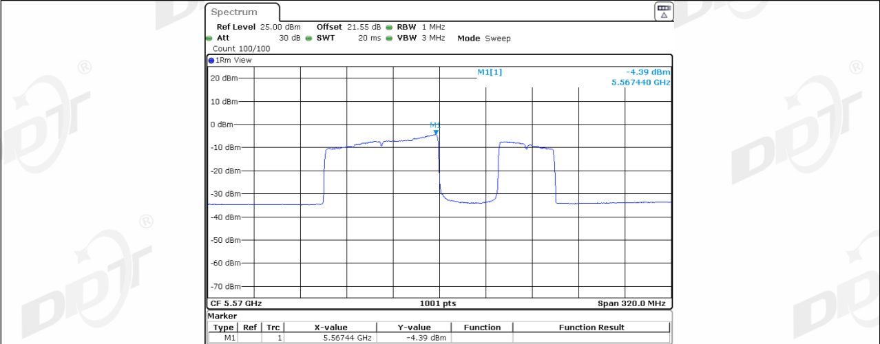
11BE160MIMO_Ant3_5570_996+484_4
