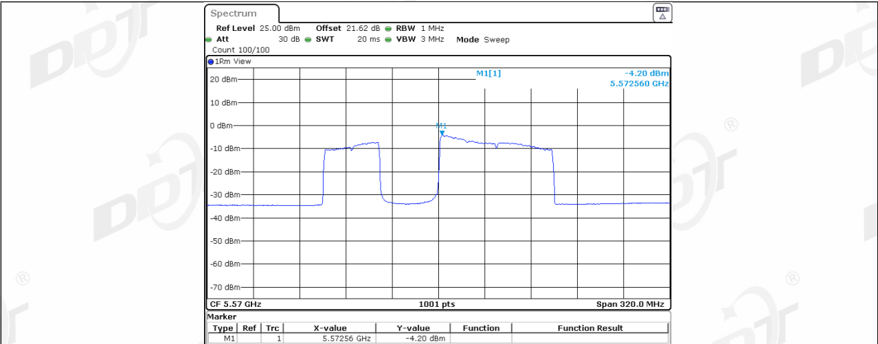
11BE160MIMO_Ant3_5570_996+484_3
