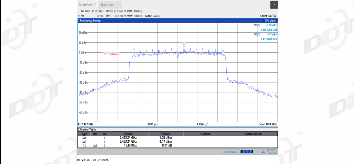
11BE20MIMO Ant2 2462
