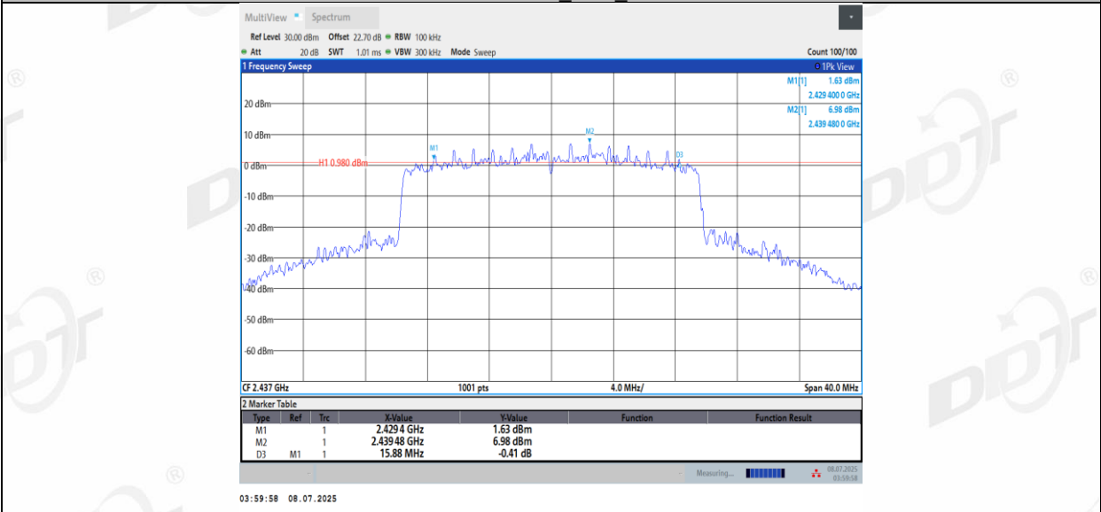
11BE20MIMO Ant2 2437
