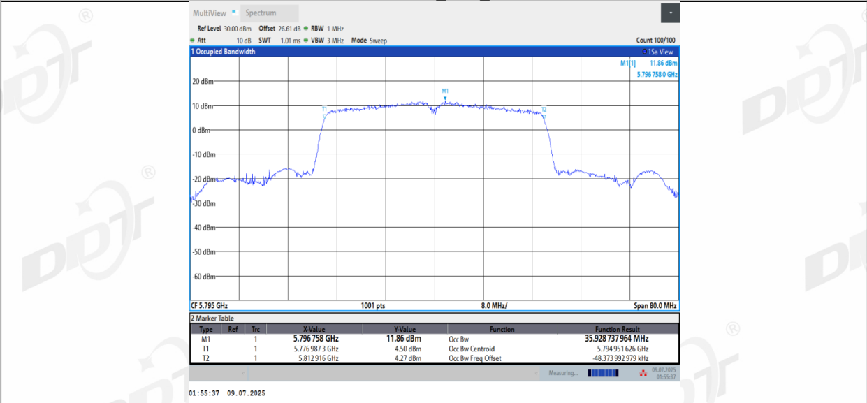
11N40MIMO_Ant3_5795
