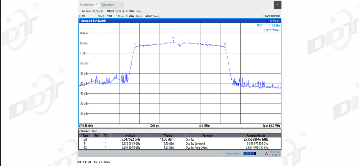
11N40MIMO_Ant3_5550
