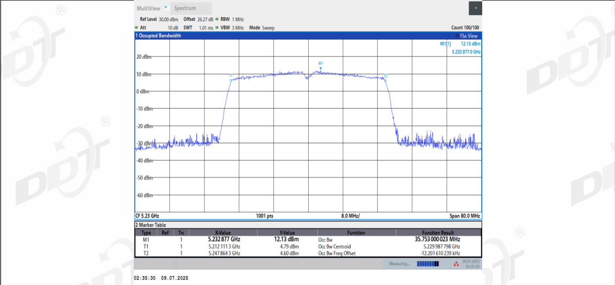
11AC40MIMO_Ant3_5230
