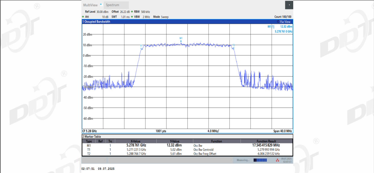
11AC20MIMO_Ant3_5280
