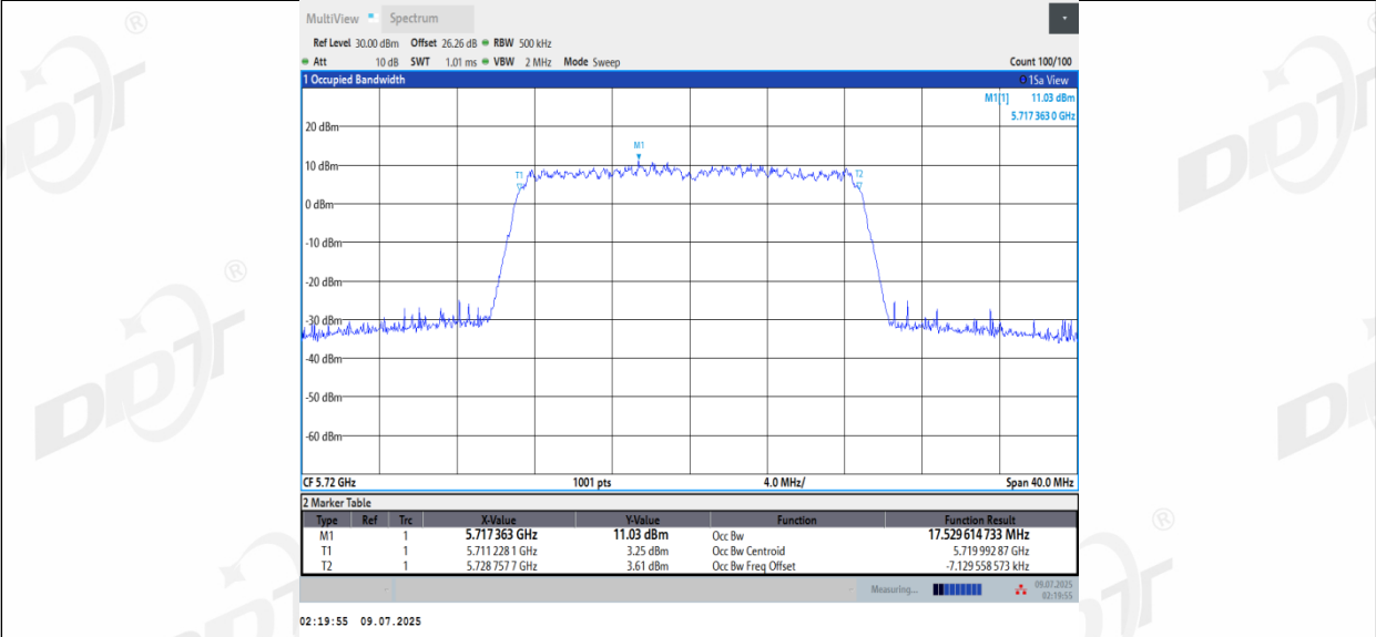
11AC20MIMO_Ant3_5720
