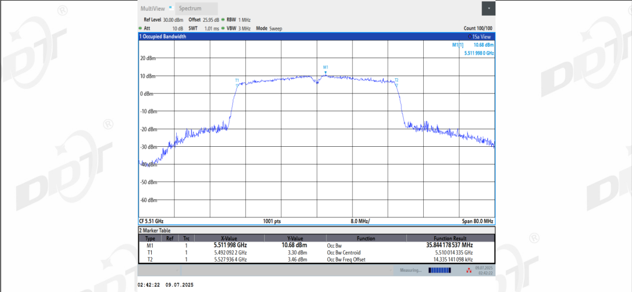
11AC40MIMO_Ant3_5510
