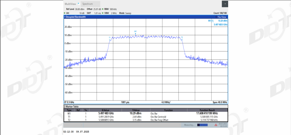
11AC20MIMO_Ant3_5500
