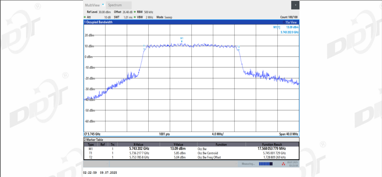
11AC20MIMO_Ant3_5745
