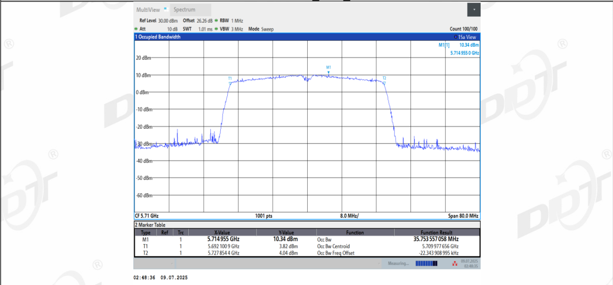
11AC40MIMO_Ant2_5710
