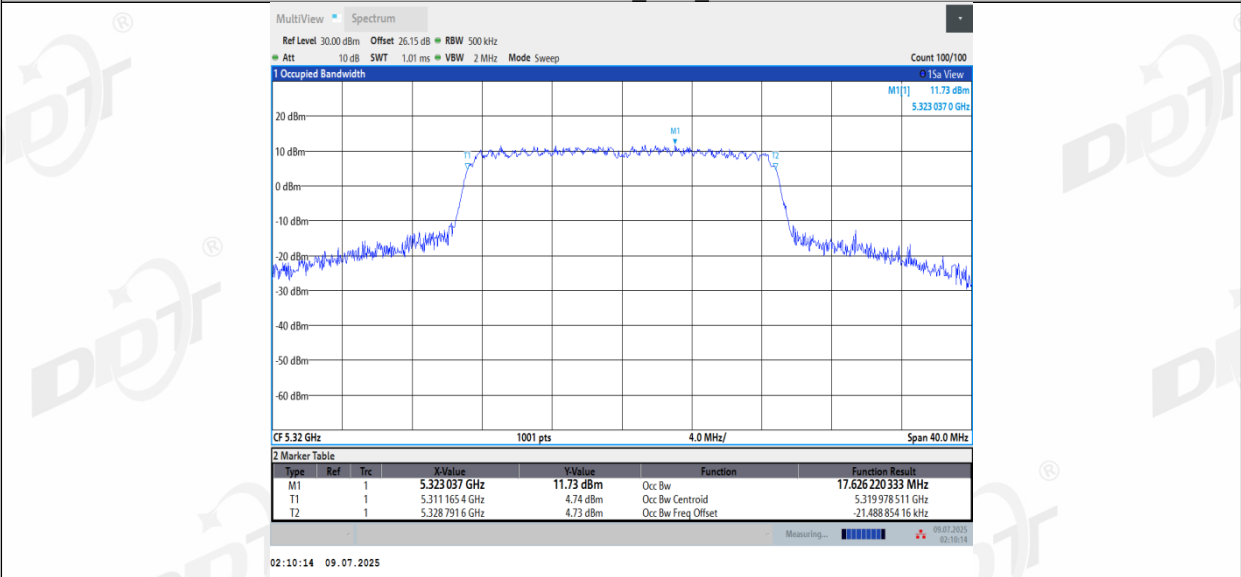
11AC20MIMO_Ant3_5320
