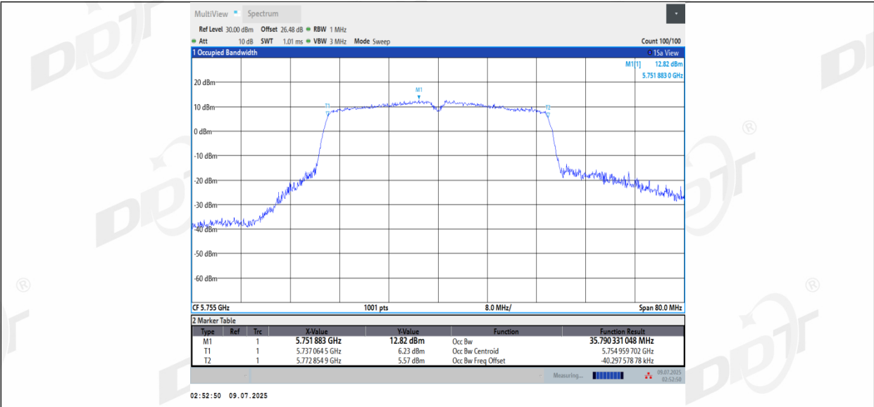
11AC40MIMO_Ant3_5755
