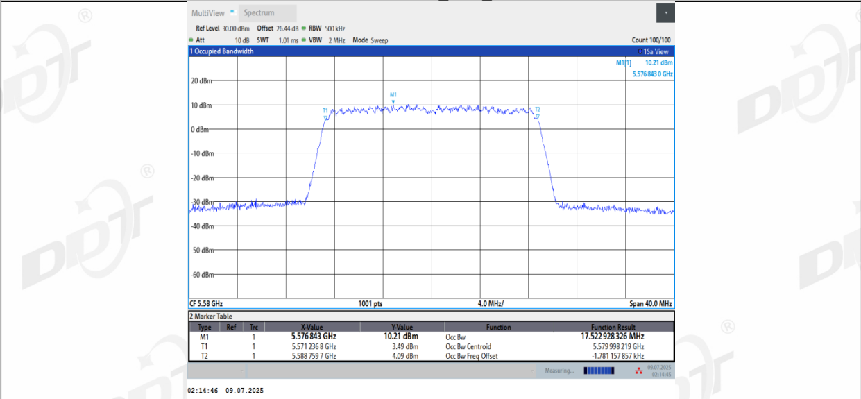
11AC20MIMO_Ant3_5580
