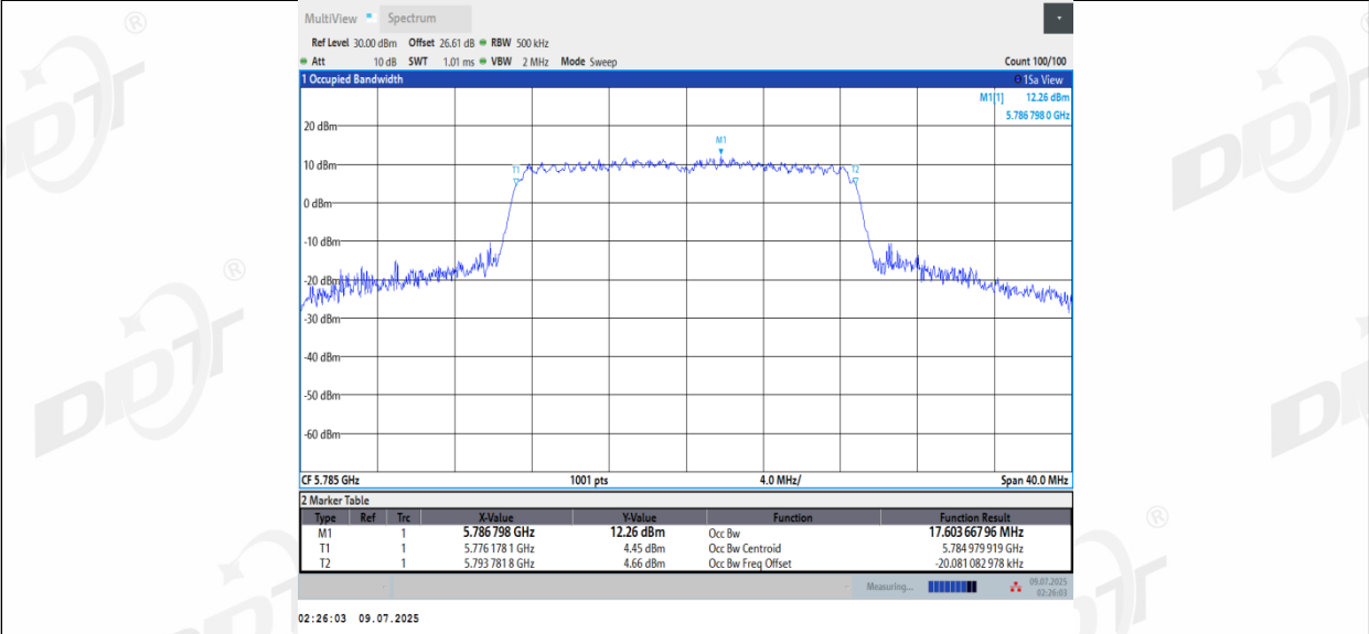
11AC20MIMO_Ant3_5785
