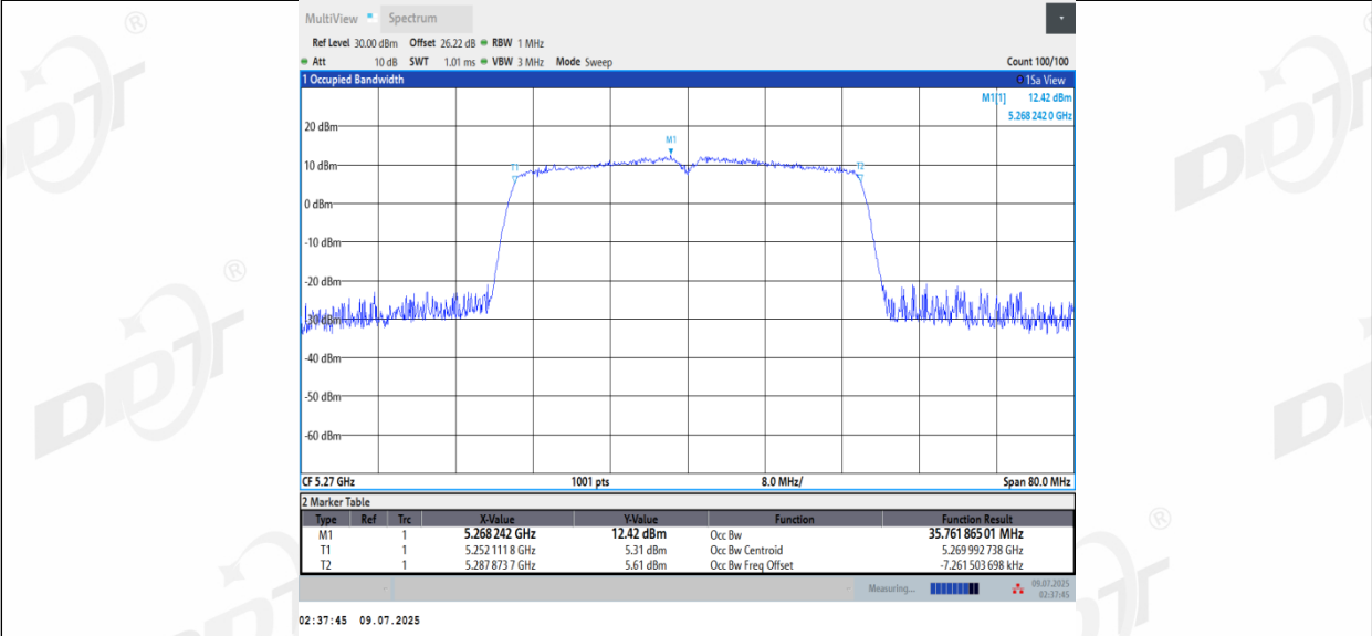
11AC40MIMO_Ant3_5270
