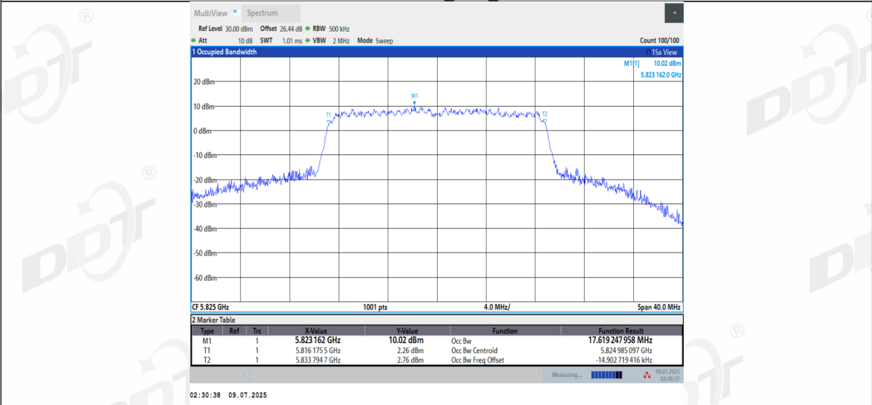
11AC20MIMO_Ant3_5825
