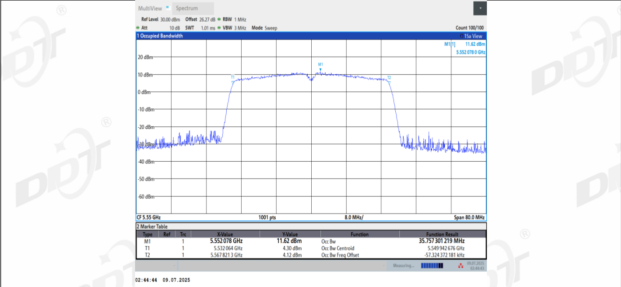
11AC40MIMO_Ant3_5550
