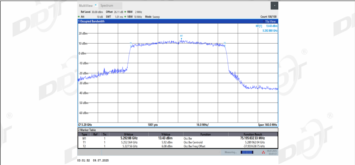
11AC80MIMO_Ant3_5290
