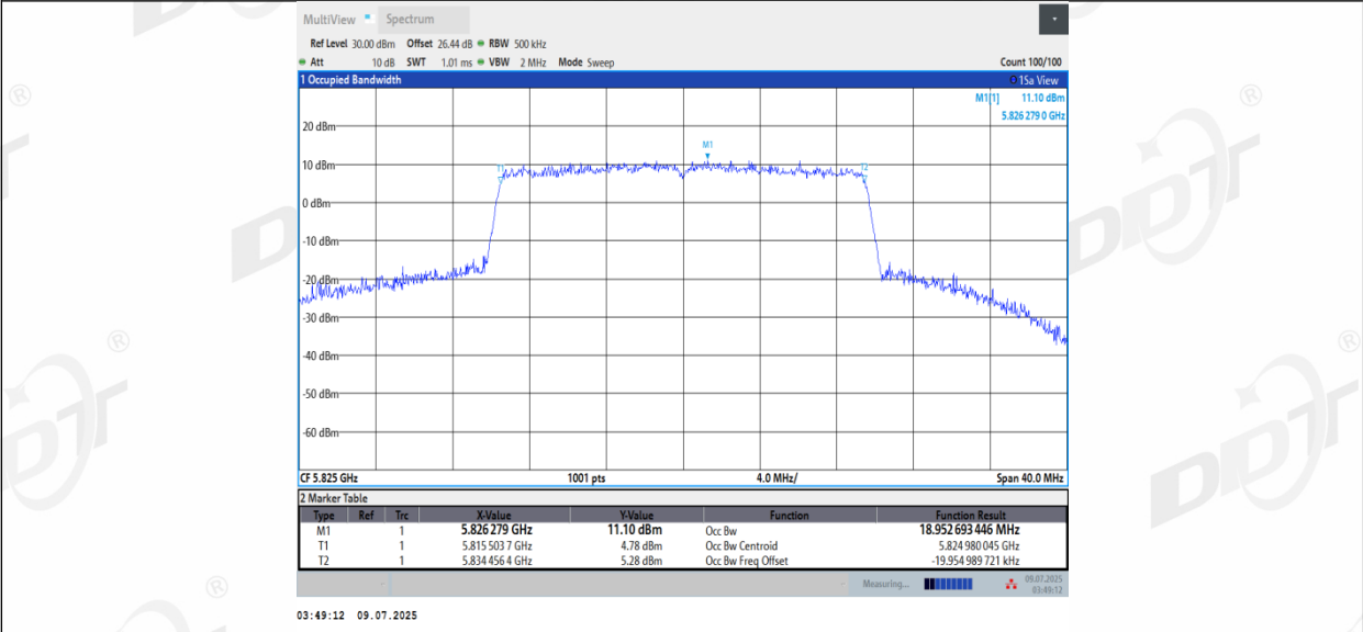
11AX20MIMO_Ant2_5825
