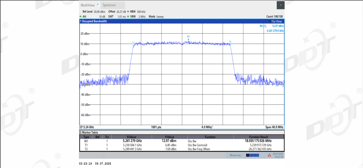
11AX20MIMO_Ant2_5240
