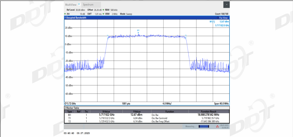
11AX20MIMO_Ant3_5720
