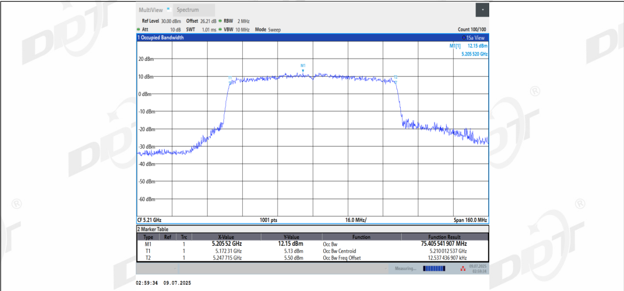
11AC80MIMO_Ant3_5210
