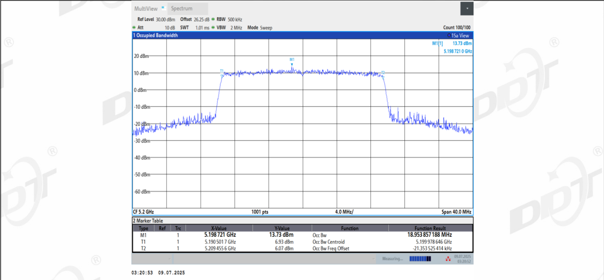
11AX20MIMO_Ant2_5200
