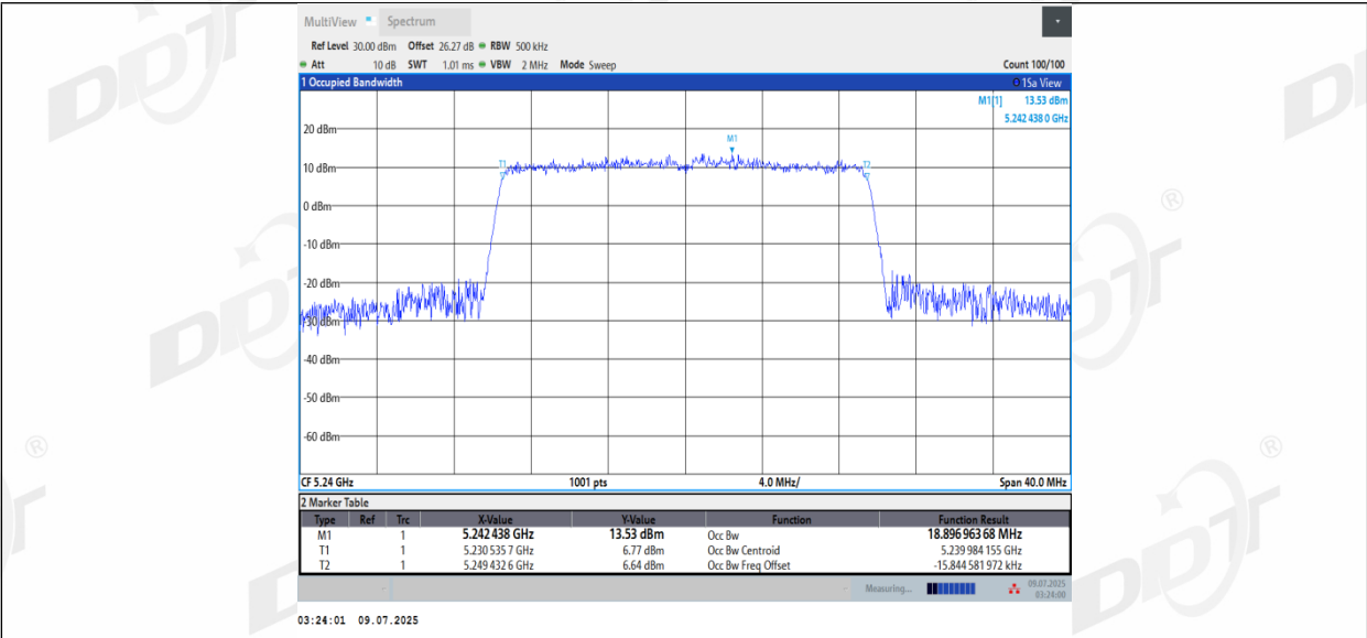
11AX20MIMO_Ant3_5240
