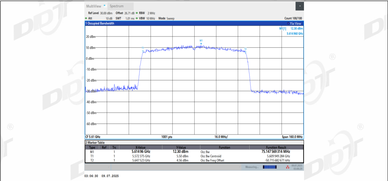
11AC80MIMO_Ant3_5610
