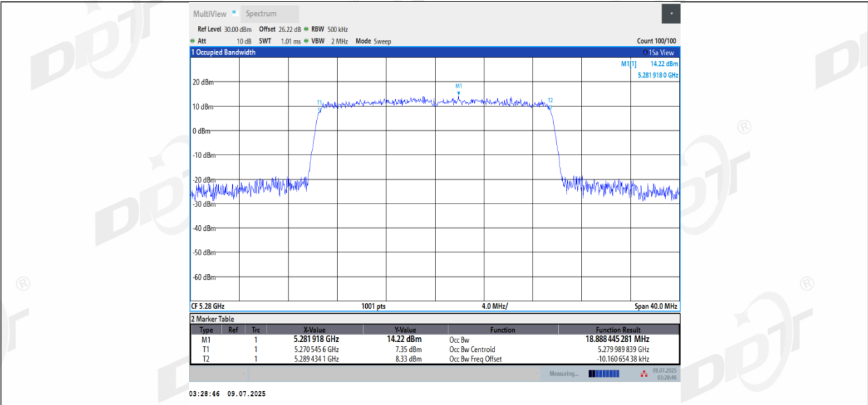
11AX20MIMO_Ant3_5280
