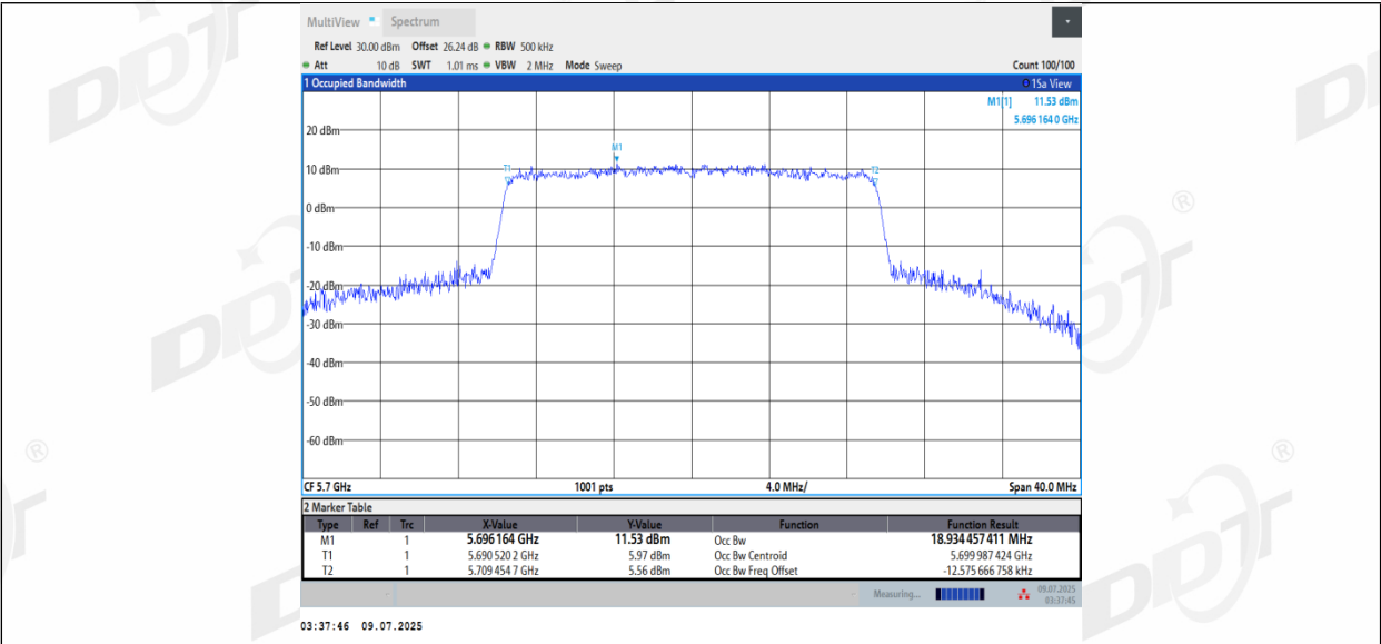
11AX20MIMO_Ant3_5700
