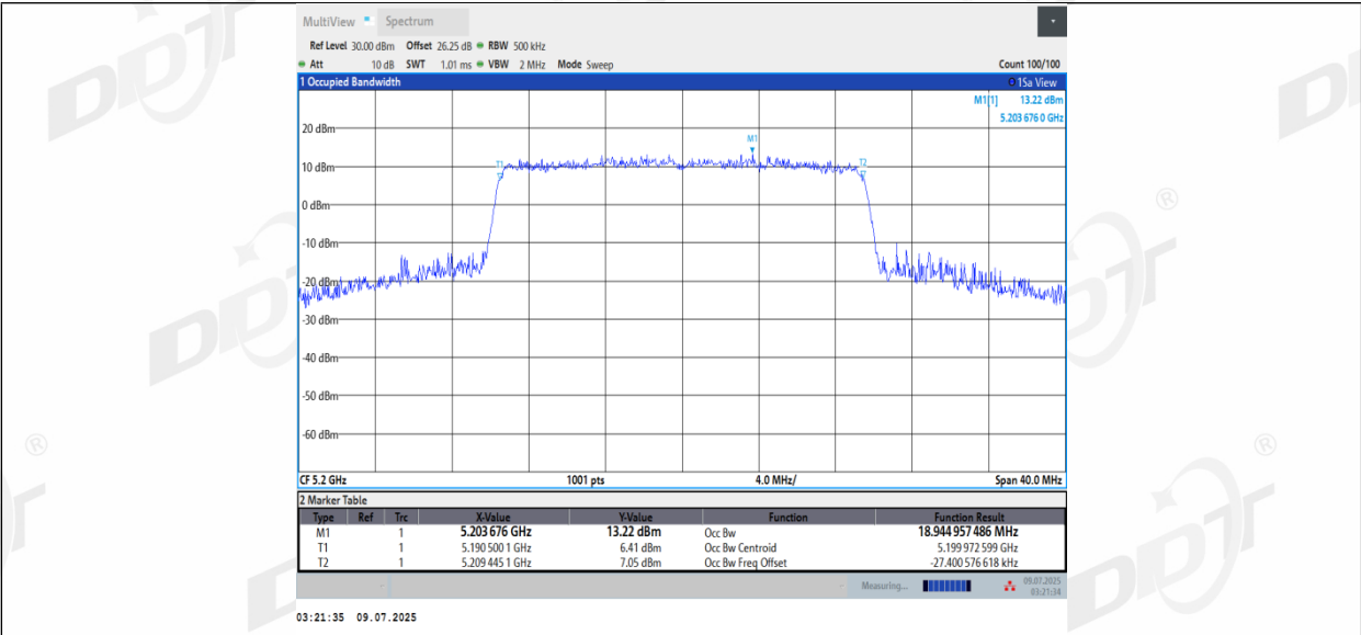
11AX20MIMO_Ant3_5200
