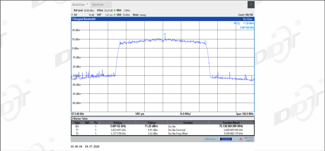
11AC80MIMO_Ant2_5690
