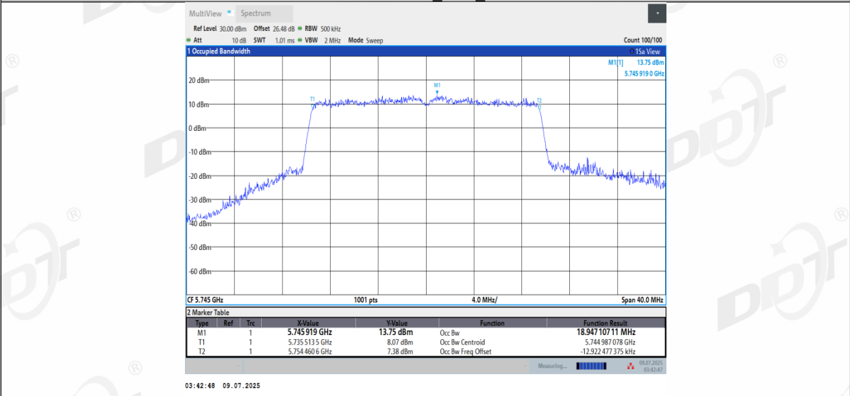
11AX20MIMO_Ant2_5745
