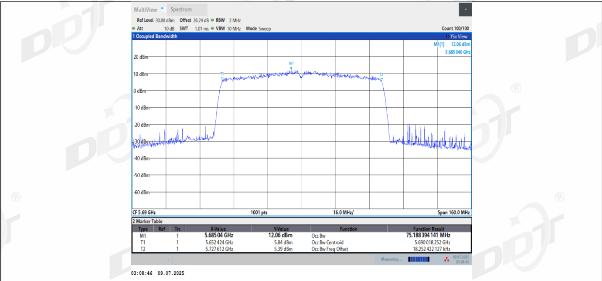
11AC80MIMO_Ant3_5690
