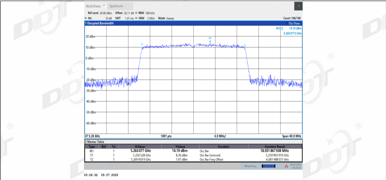
11AX20MIMO_Ant3_5260
