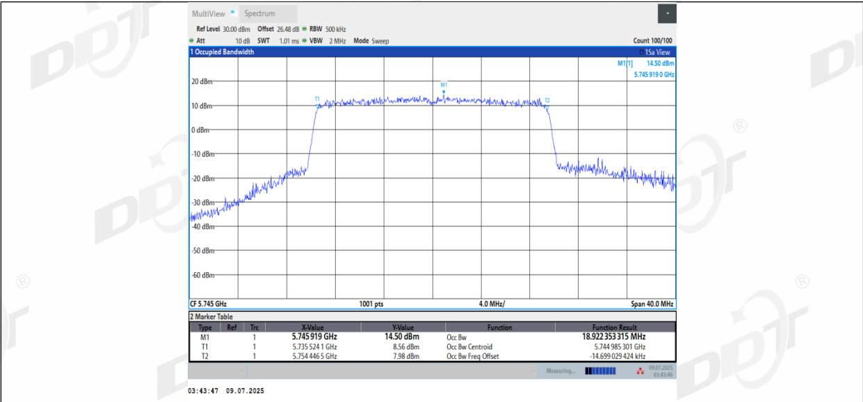
11AX20MIMO_Ant3_5745
