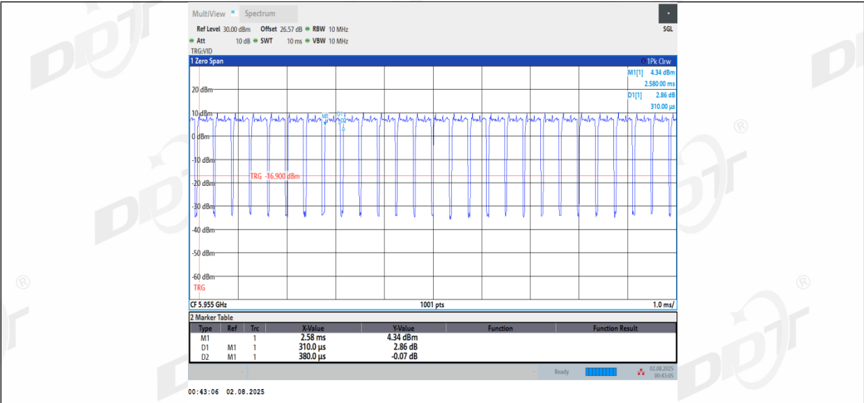
11BE20MIMO_Ant2_5955
