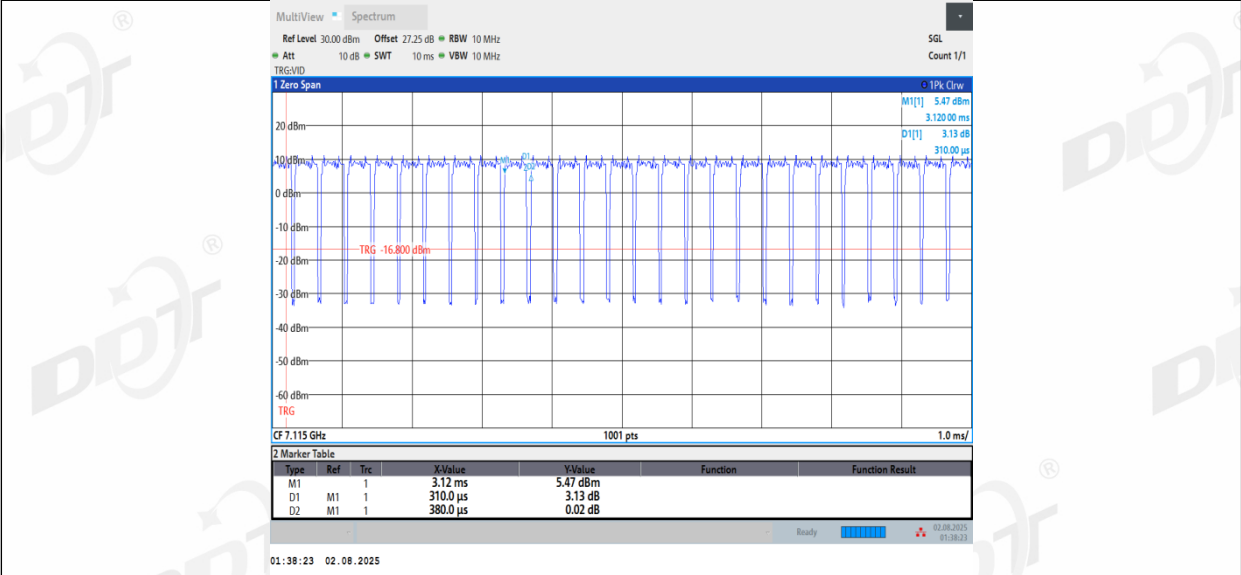
11BE20MIMO_Ant3_7115
