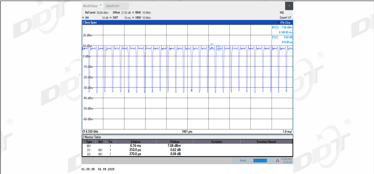
11BE20MIMO_Ant2_6535
