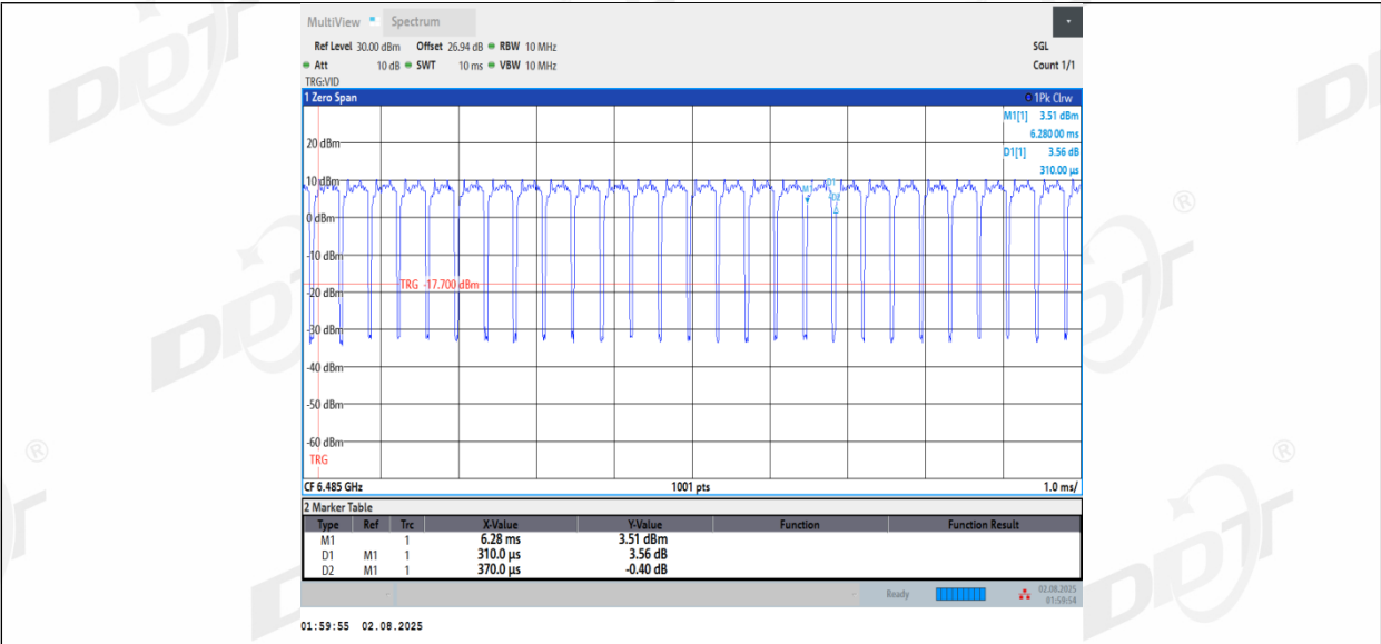
11BE40MIMO_Ant2_6485
