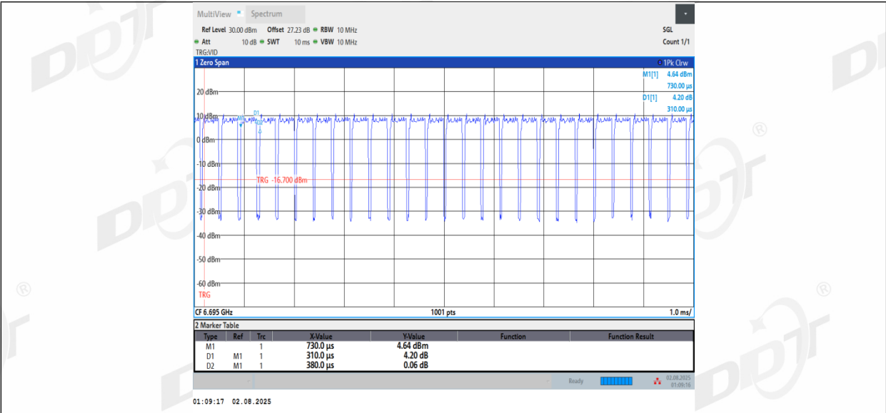
11BE20MIMO_Ant2_6695
