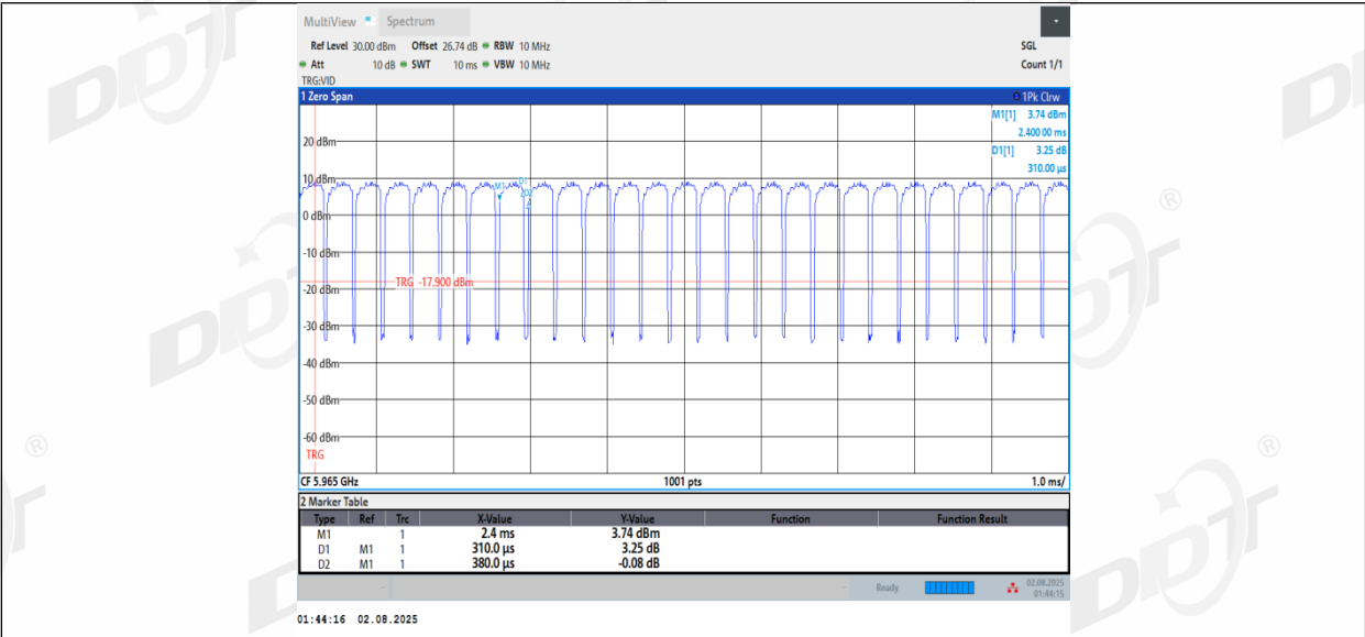
11BE40MIMO_Ant2_5965
