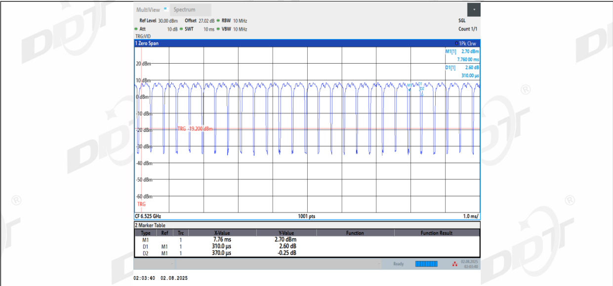
11BE40MIMO_Ant2_6525
