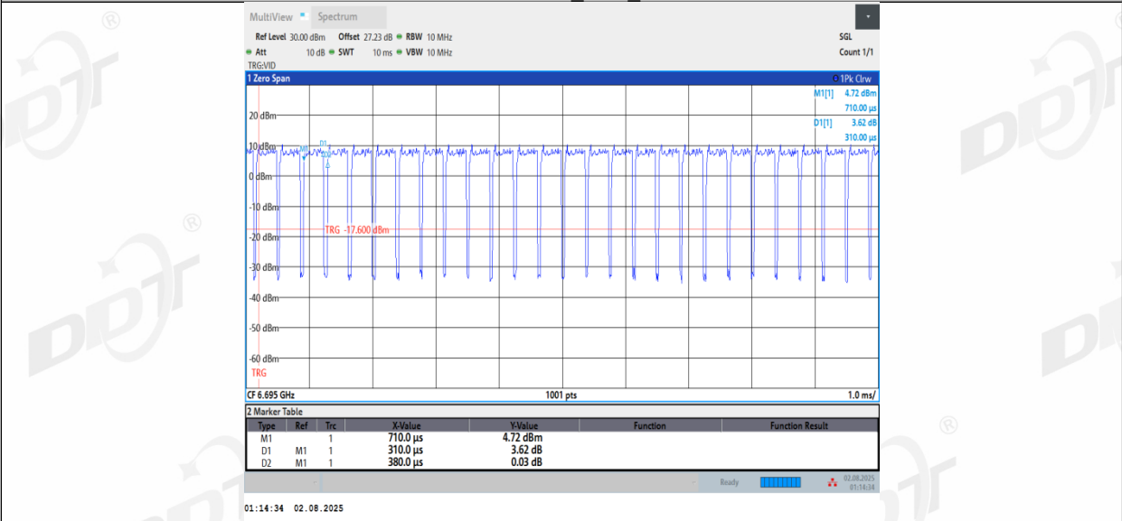
11BE20MIMO_Ant3_6695
