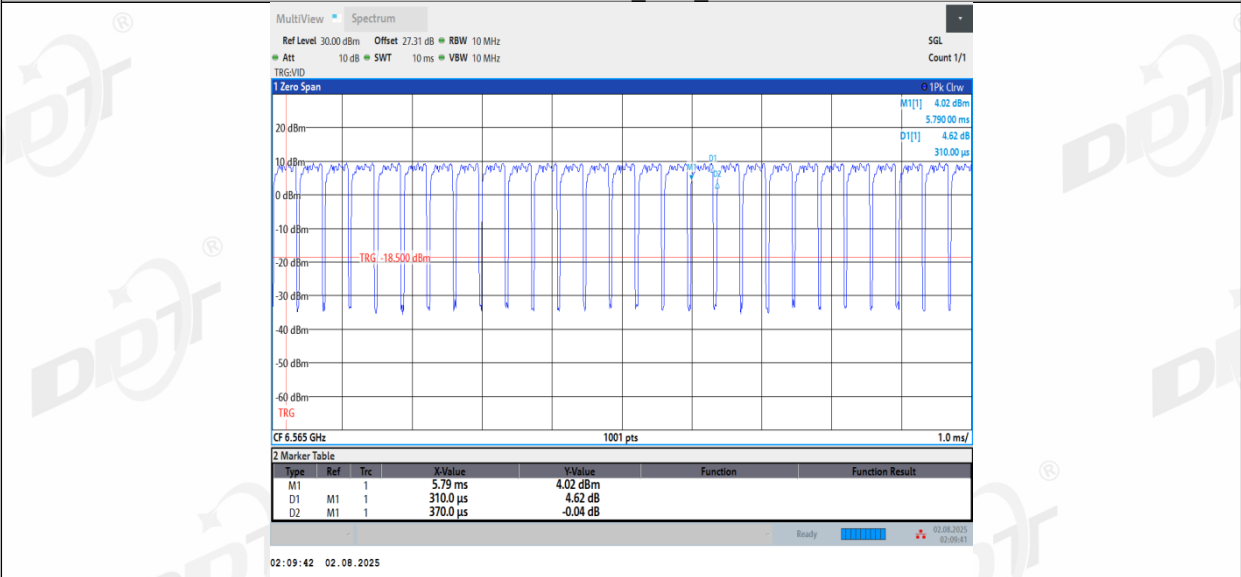
11BE40MIMO_Ant3_6565
