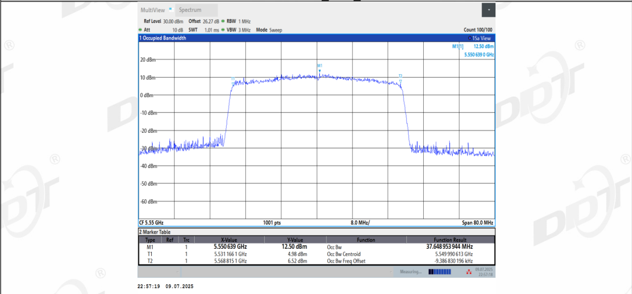
11AX40MIMO_Ant2_5550
