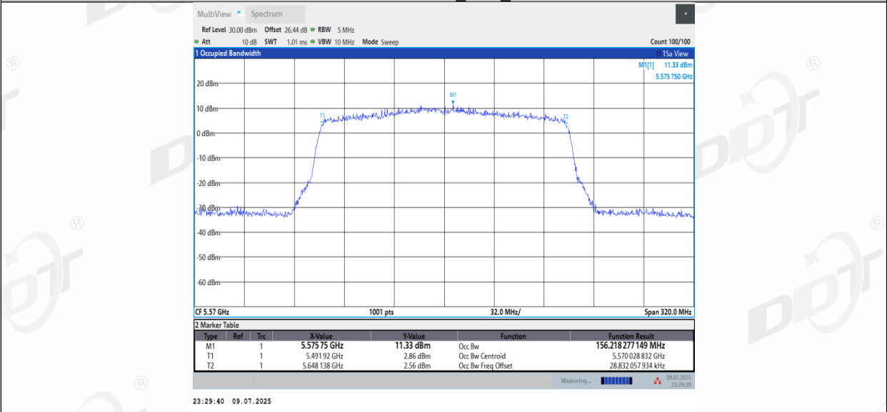
11AX160MIMO_Ant2_5570
