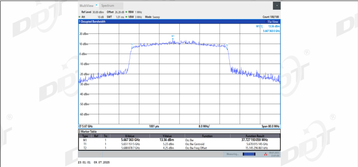
11AX40MIMO_Ant3_5670
