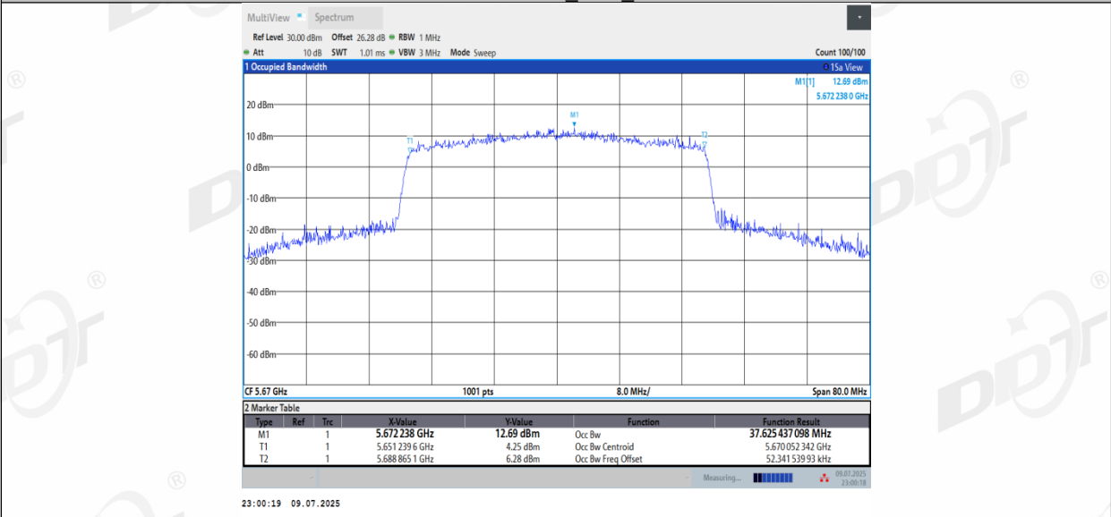
11AX40MIMO_Ant2_5670
