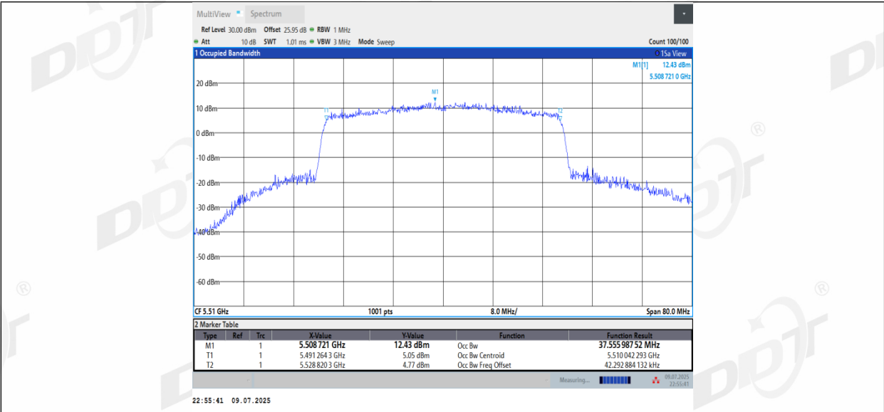
11AX40MIMO_Ant3_5510
