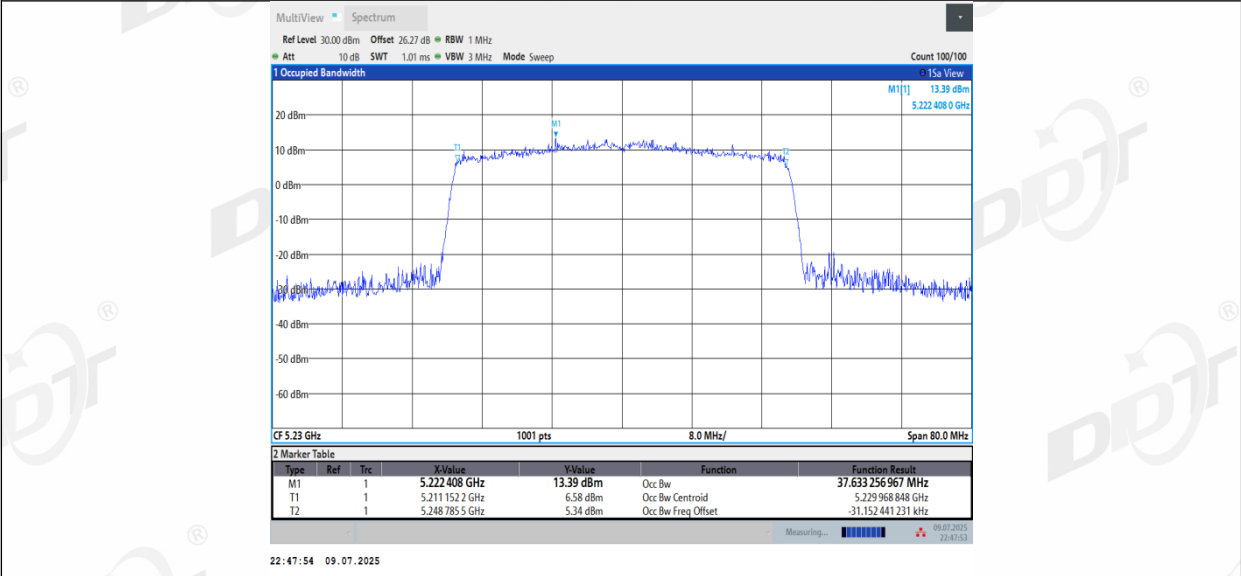
11AX40MIMO_Ant2_5230
