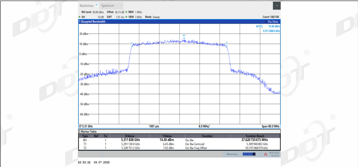
11AX40MIMO_Ant3_5310
