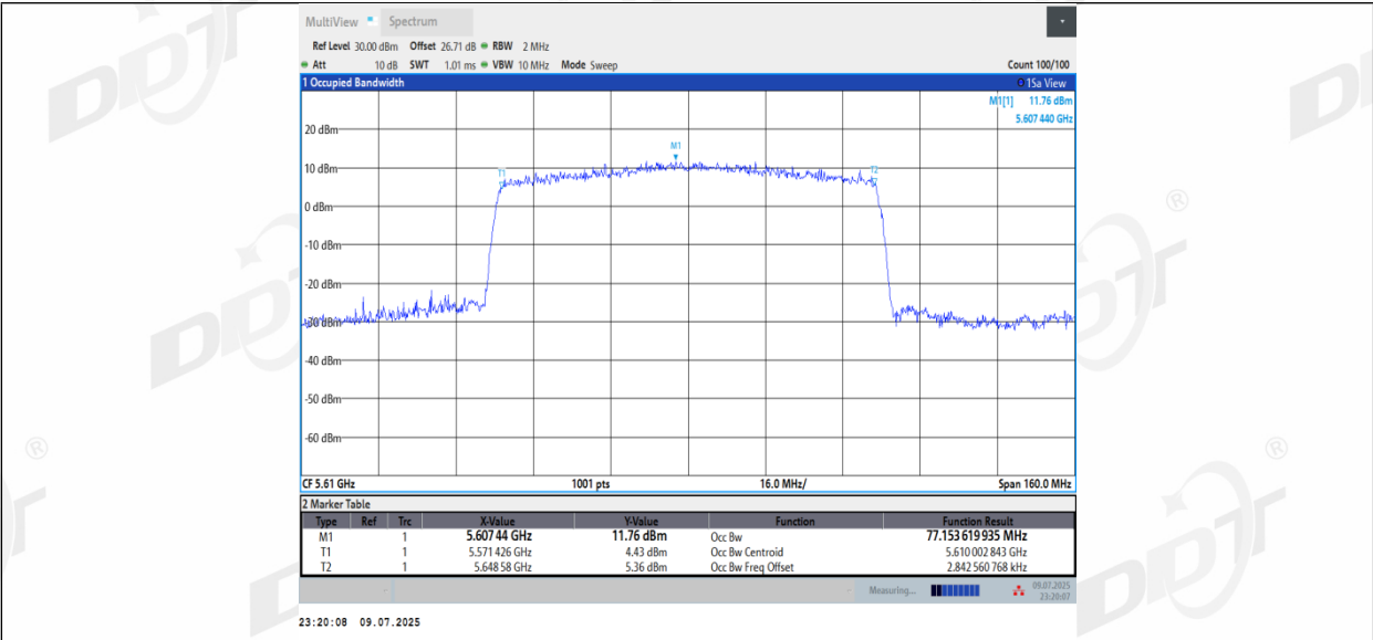
11AX80MIMO_Ant3_5610
