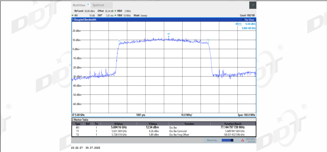
11AX80MIMO_Ant3_5690
