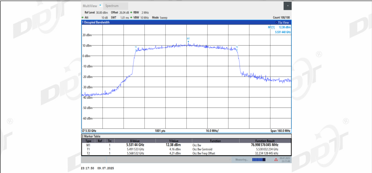
11AX80MIMO_Ant3_5530
