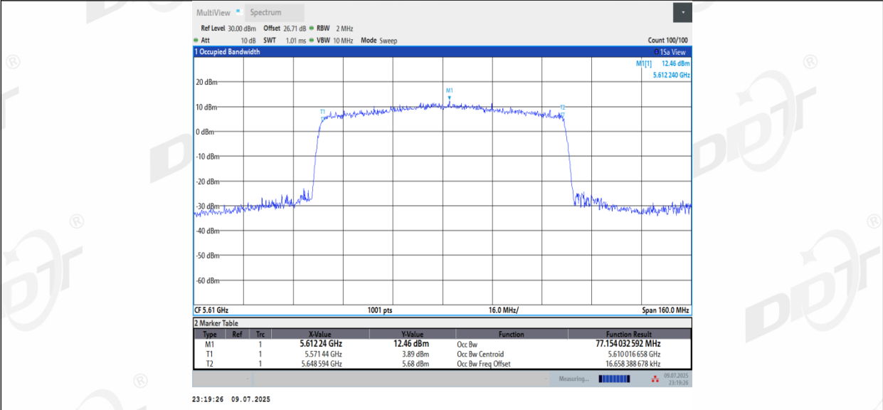
11AX80MIMO_Ant2_5610
