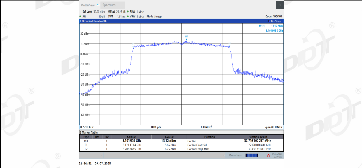
11AX40MIMO_Ant2_5190
