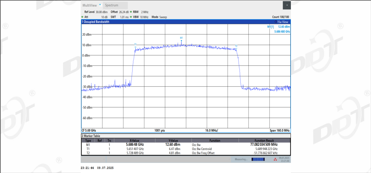
11AX80MIMO_Ant2_5690
