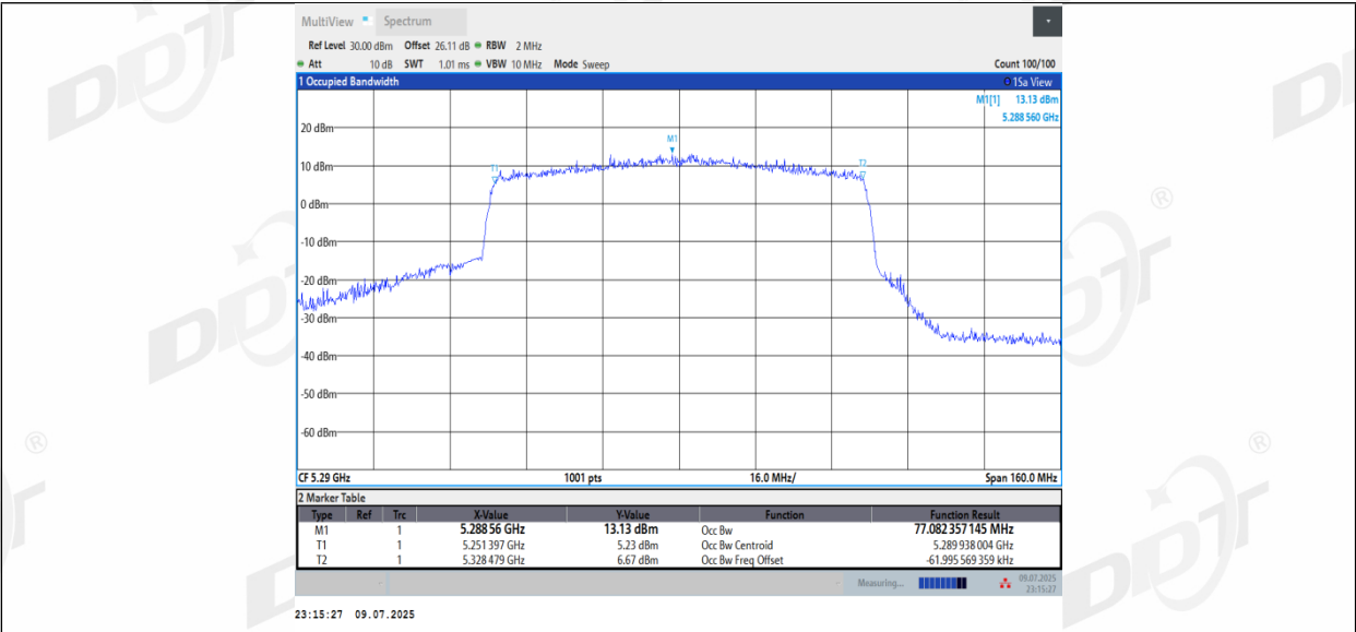
11AX80MIMO_Ant3_5290
