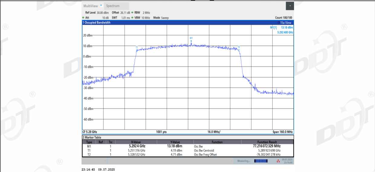
11AX80MIMO_Ant2_5290
