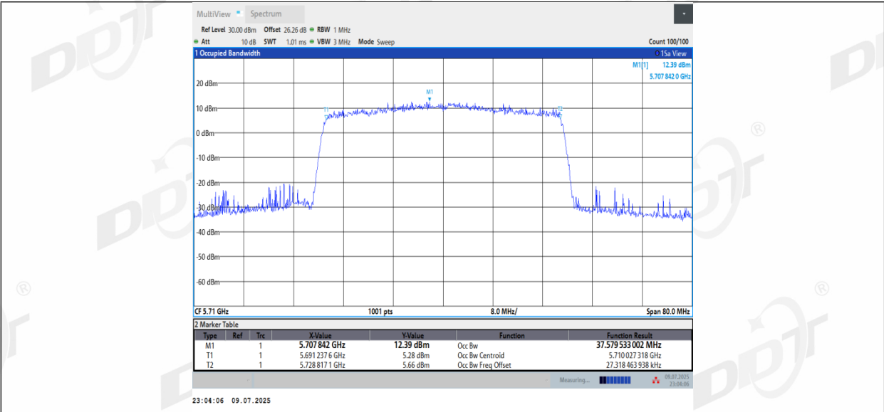
11AX40MIMO_Ant3_5710
