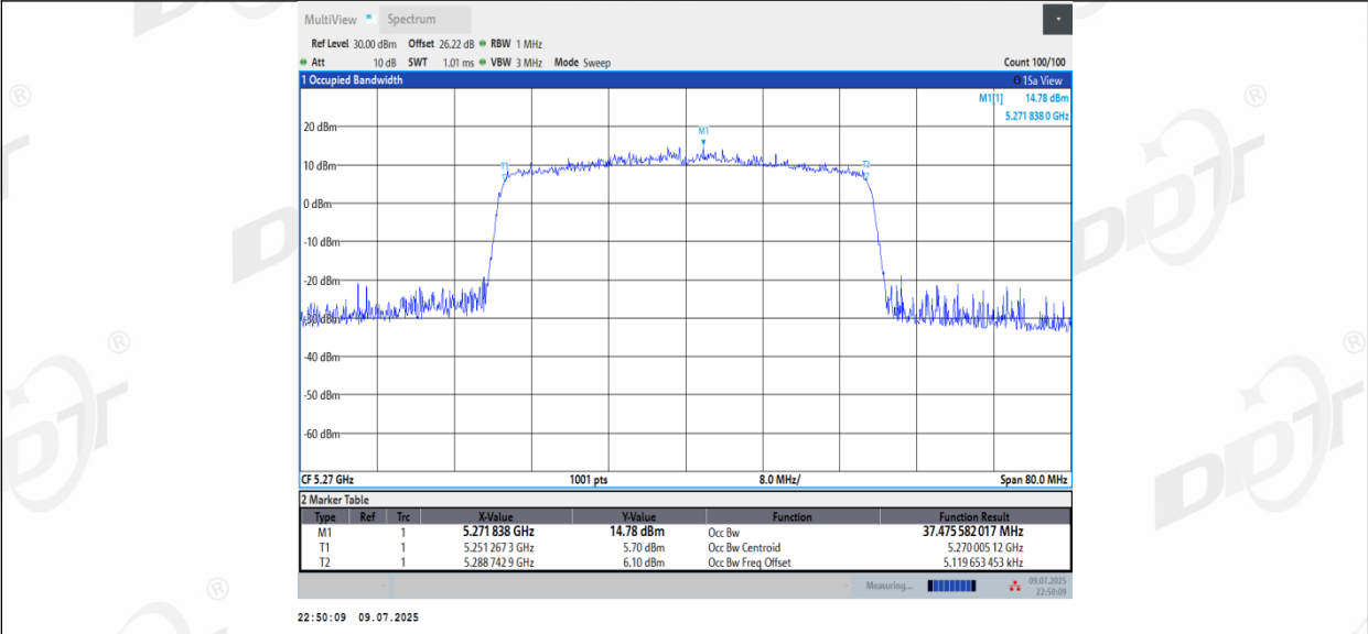
11AX40MIMO_Ant2_5270
