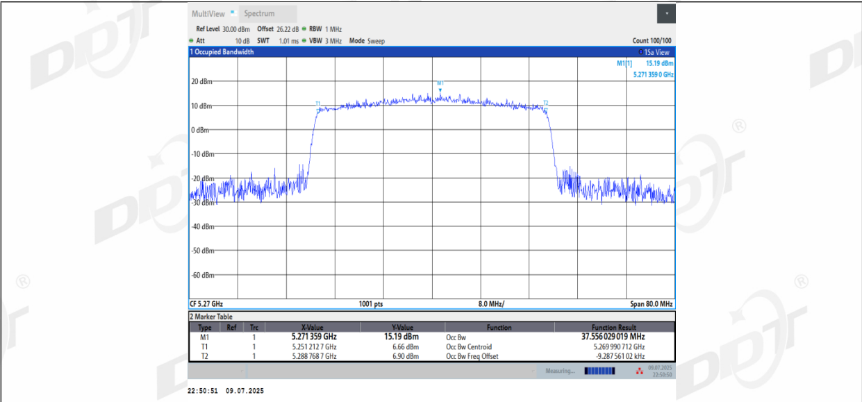
11AX40MIMO_Ant3_5270
