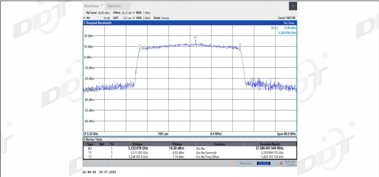
11AX40MIMO_Ant3_5230
