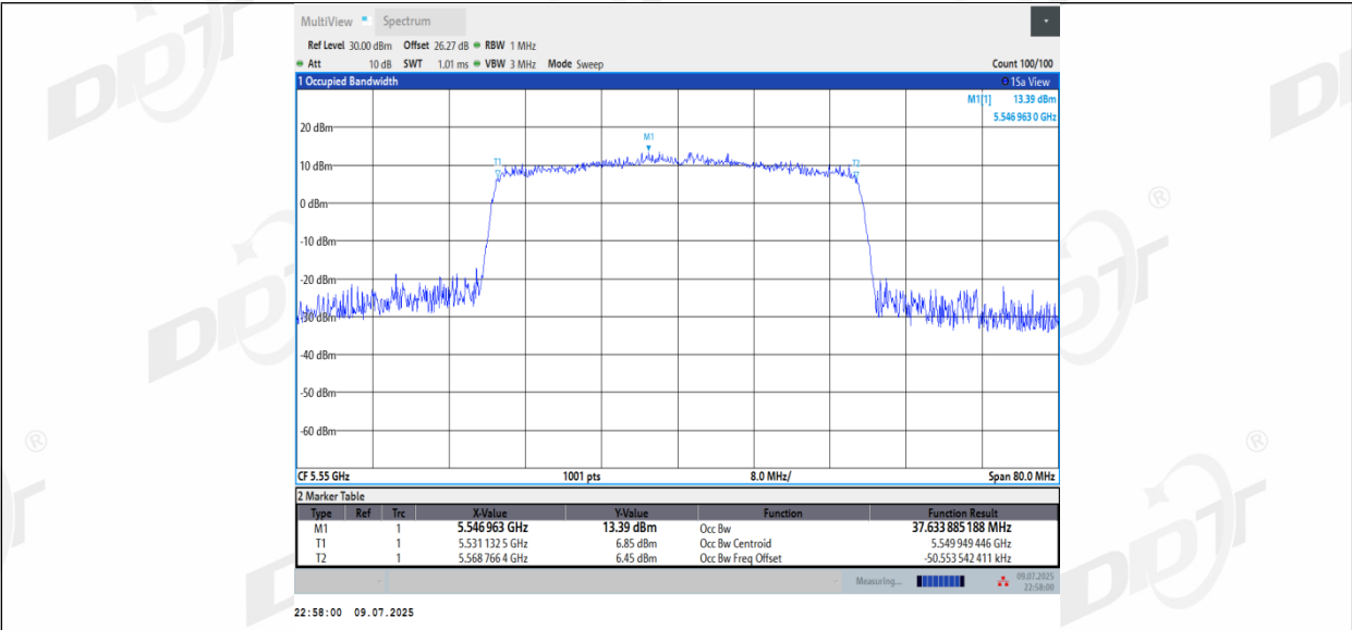
11AX40MIMO_Ant3_5550
