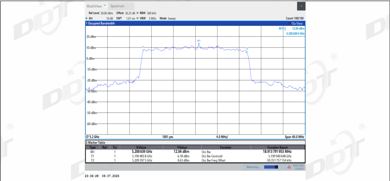
11BE20MIMO_Ant3_5200
