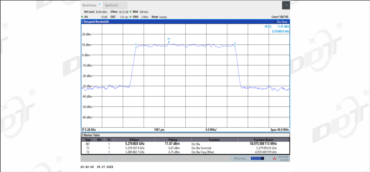
11BE20MIMO_Ant2_5280
