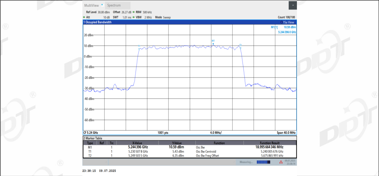
11BE20MIMO_Ant2_5240
