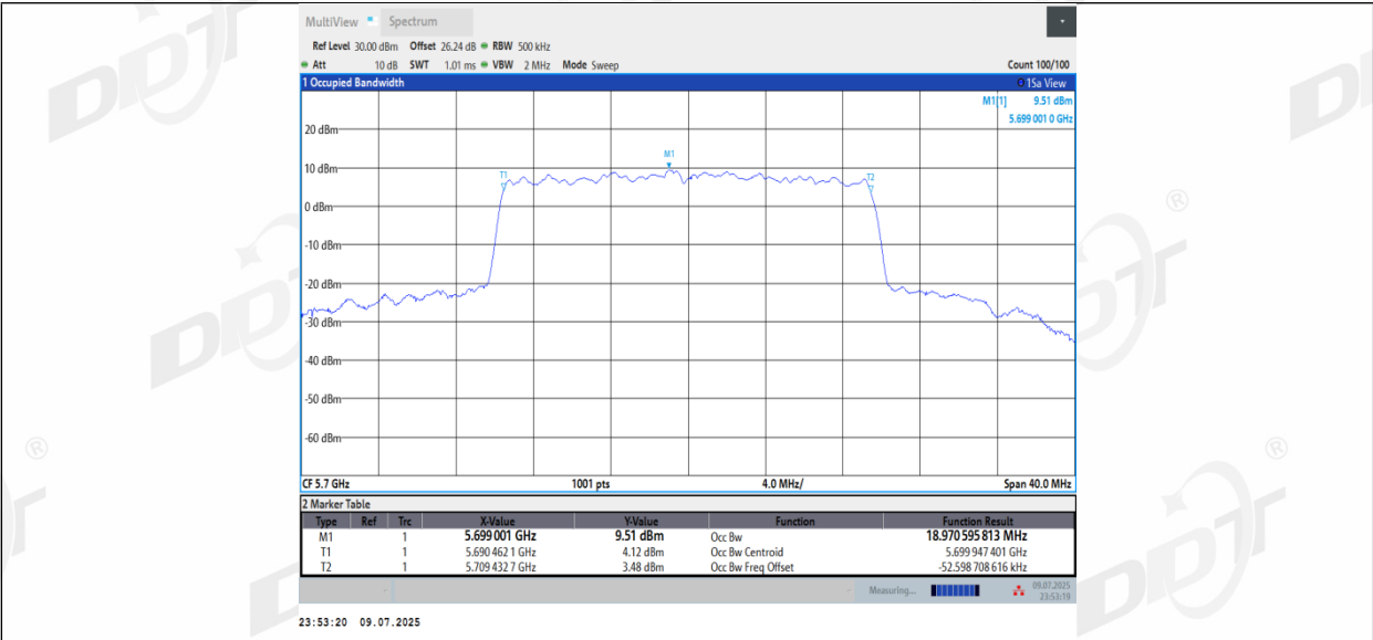
11BE20MIMO_Ant3_5700
