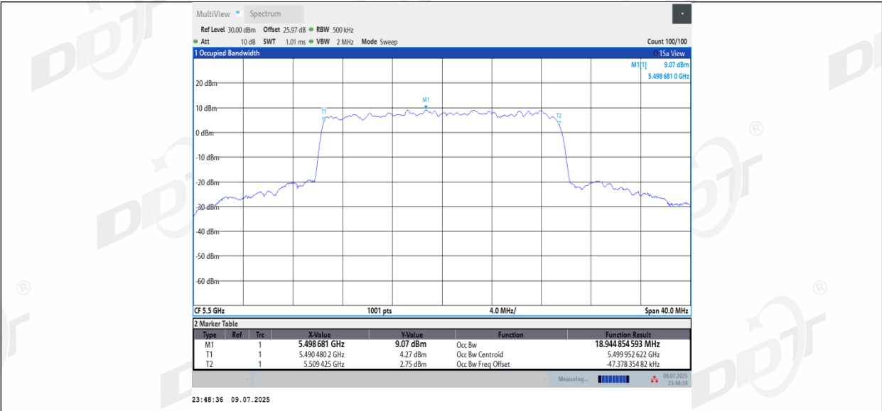
11BE20MIMO_Ant3_5500
