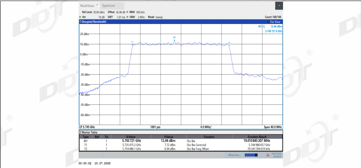
11BE20MIMO_Ant3_5745
