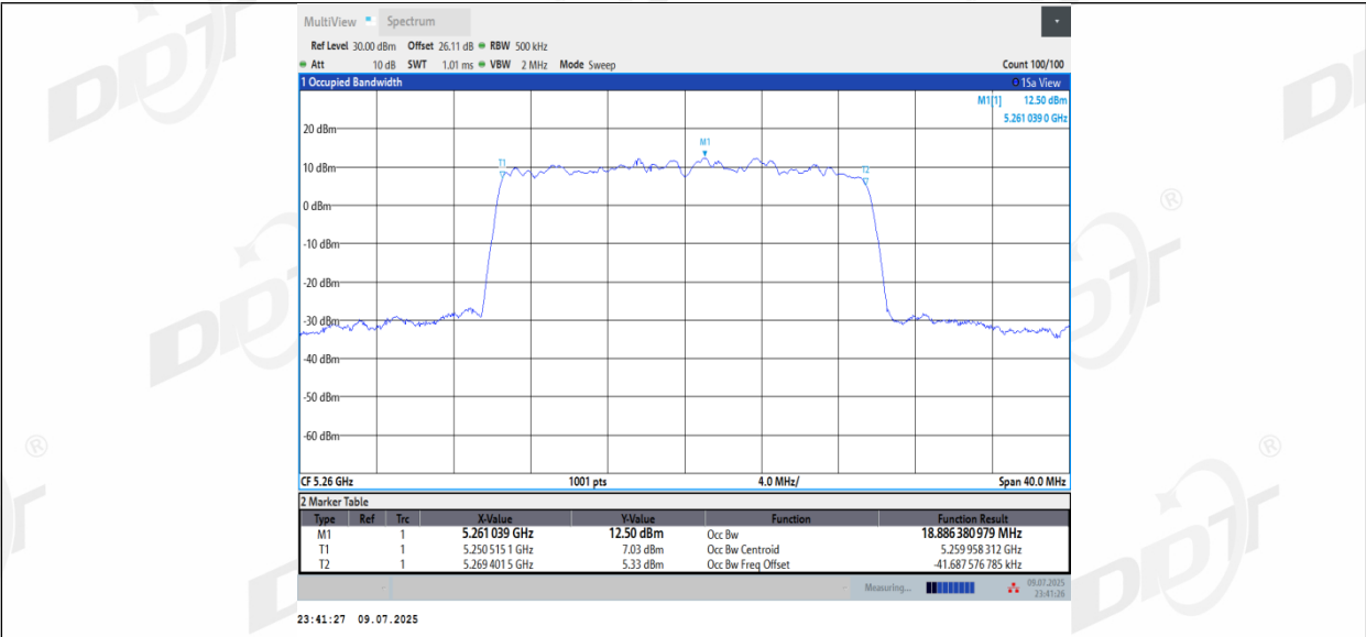
11BE20MIMO_Ant3_5260
