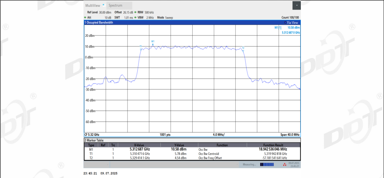
11BE20MIMO_Ant2_5320
