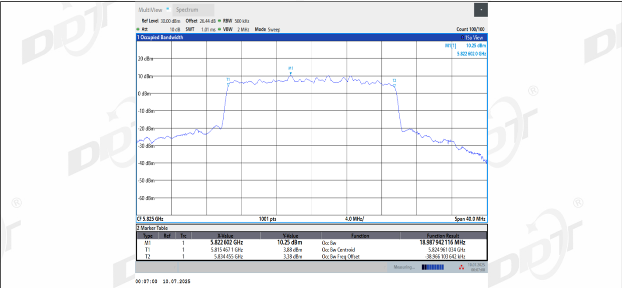
11BE20MIMO_Ant3_5825
