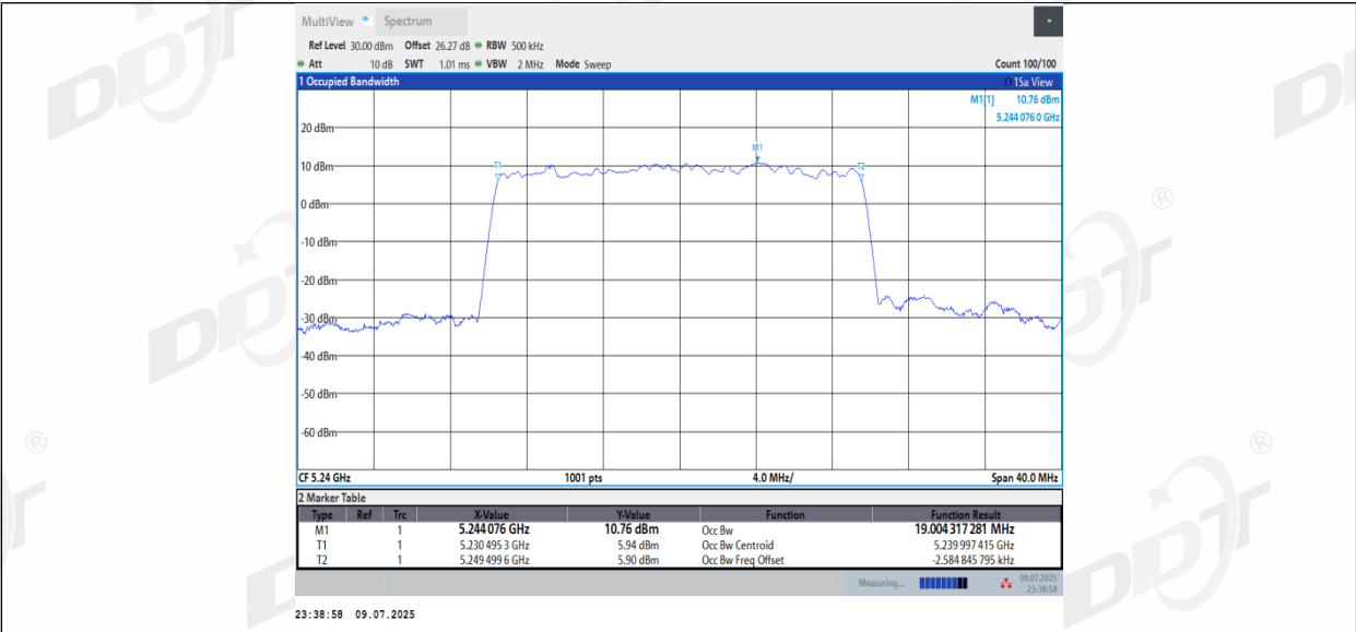
11BE20MIMO_Ant3_5240
