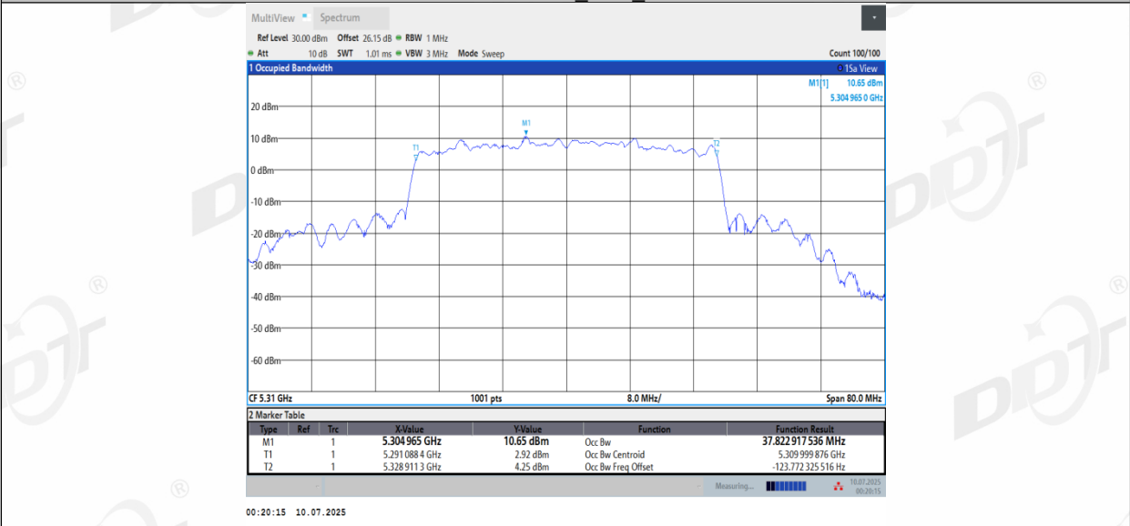
11BE40MIMO_Ant2_5310
