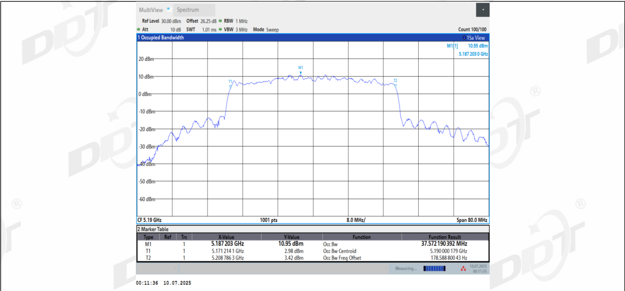
11BE40MIMO_Ant3_5190
