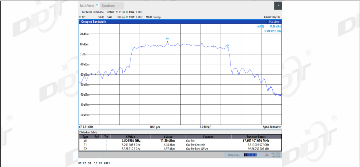
11BE40MIMO_Ant3_5310
