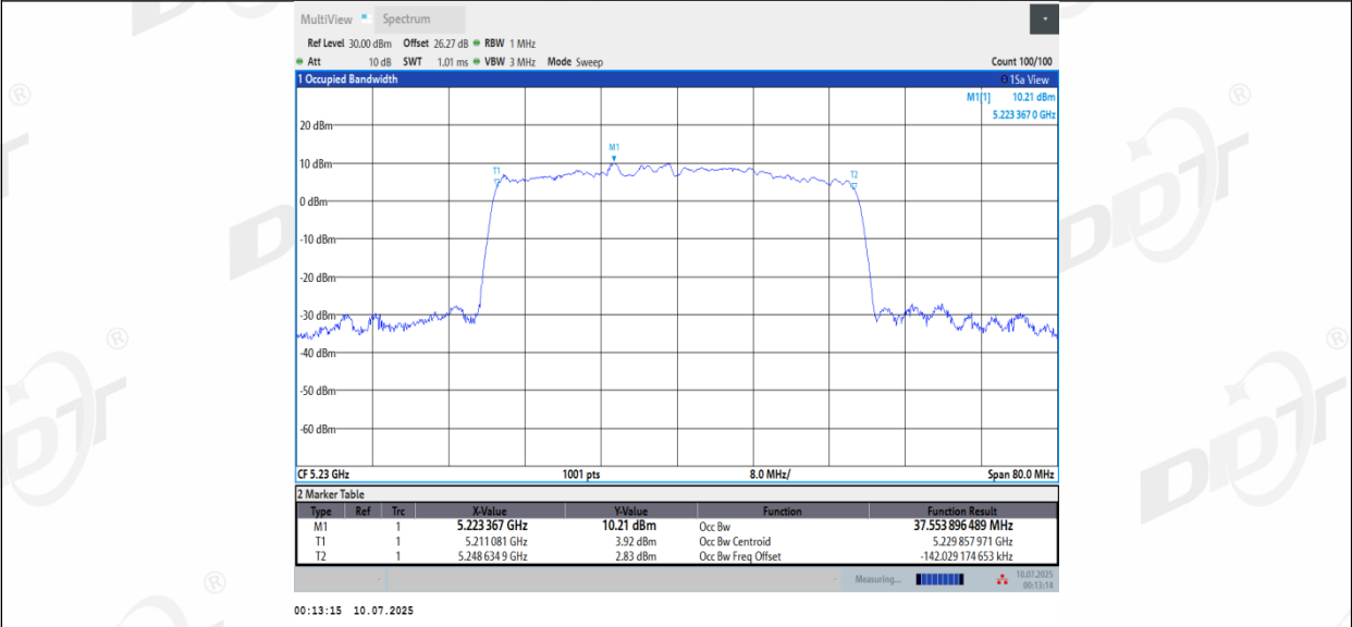
11BE40MIMO_Ant2_5230
