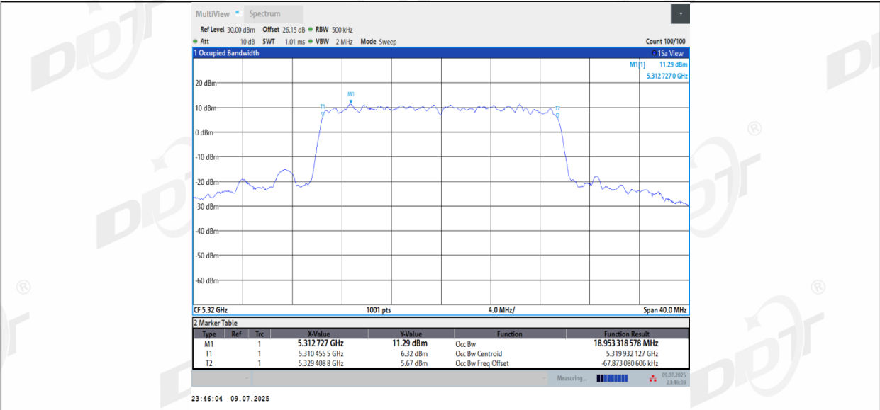
11BE20MIMO_Ant3_5320
