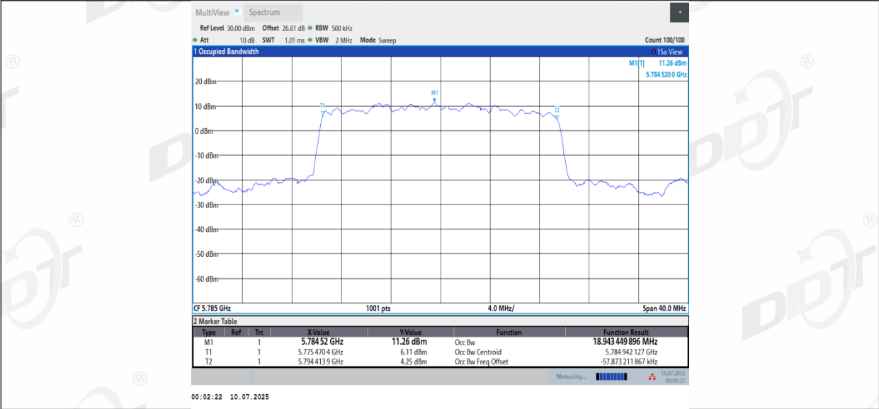
11BE20MIMO_Ant2_5785
