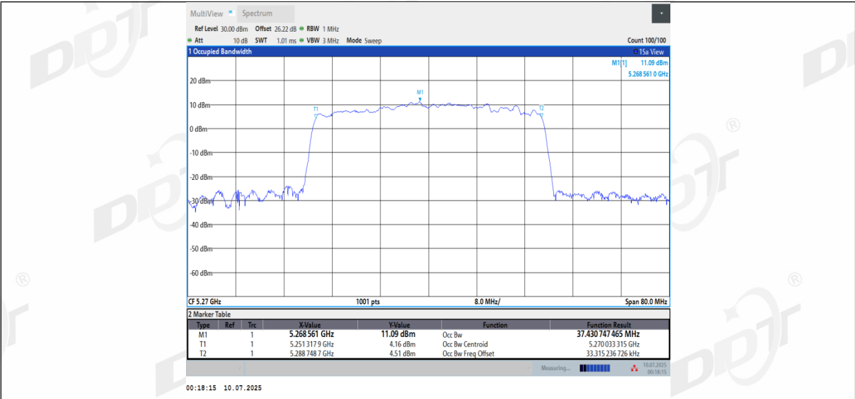
11BE40MIMO_Ant3_5270
